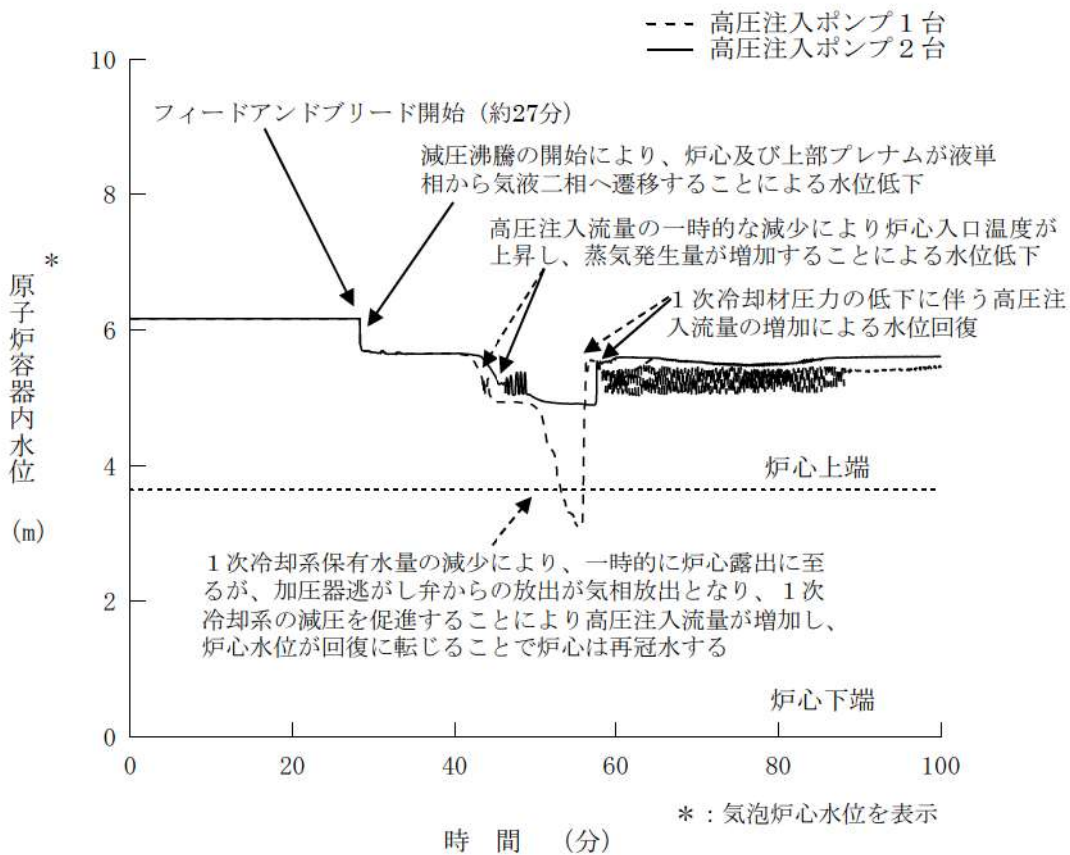
第 7. 1. 1. 20 図 原子炉容器内水位の推移 (高圧注入ポンプ 1 台の場合)
