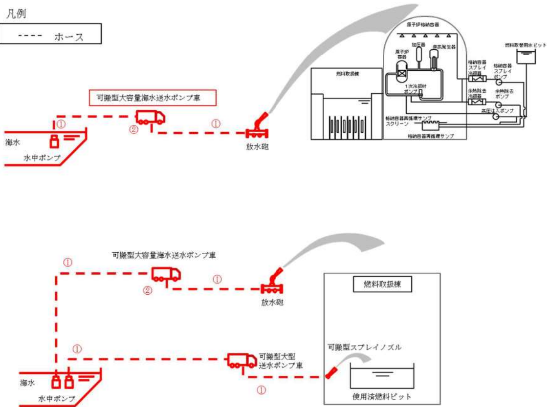
図 55-4-1 放水設備（大気への拡散抑制設備）及びスプレー設備（大気への拡散抑制設備）による大気への放射性物質の拡散抑制
