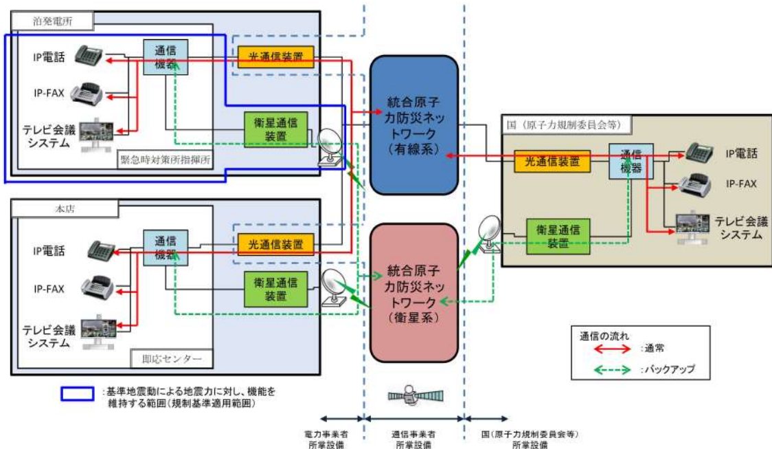
図 4-8 通信連絡設備の耐震設計範囲
