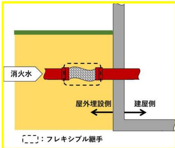
第 1-23 図：地震変位対策の実施例
