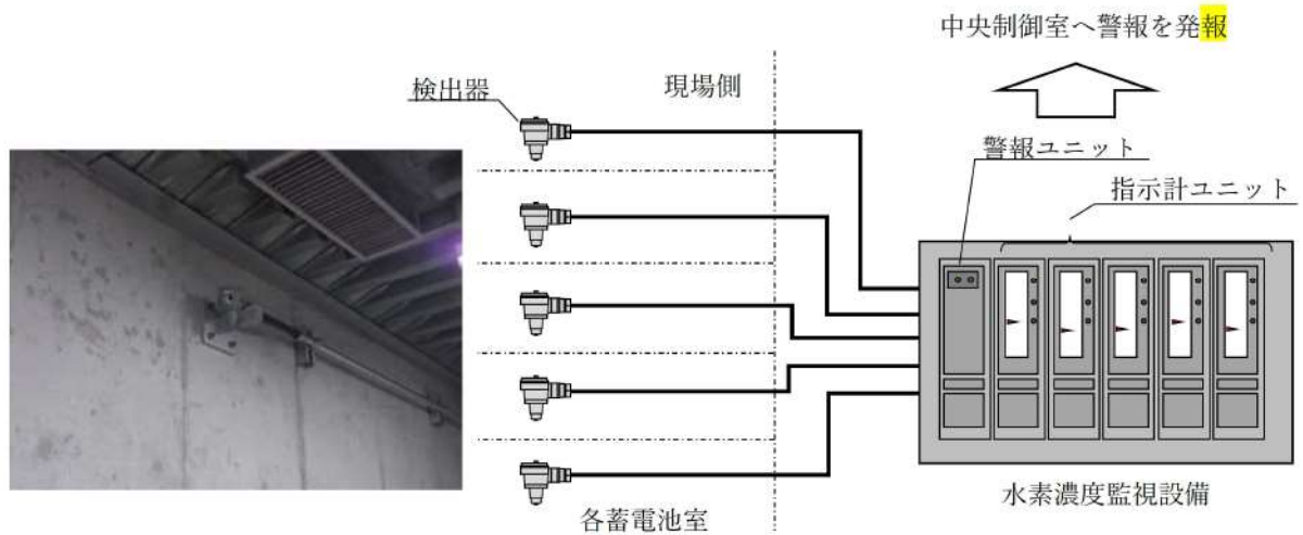
第 1-4 図：水素漏えい監視設備の概要
