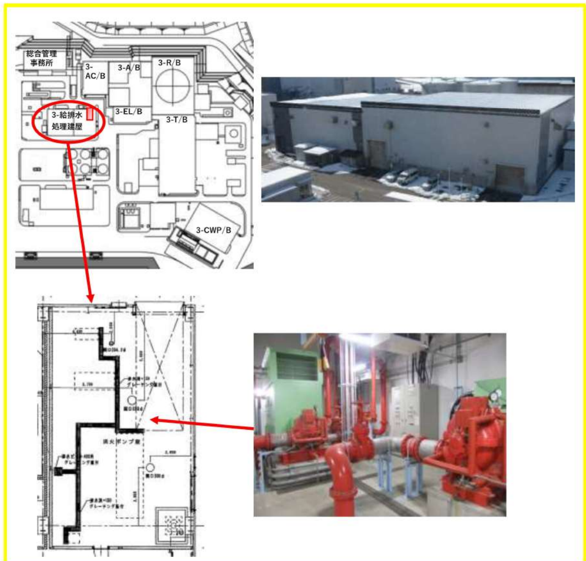
第 1-21 図：消火ポンプ設置エリアの風水害対策
