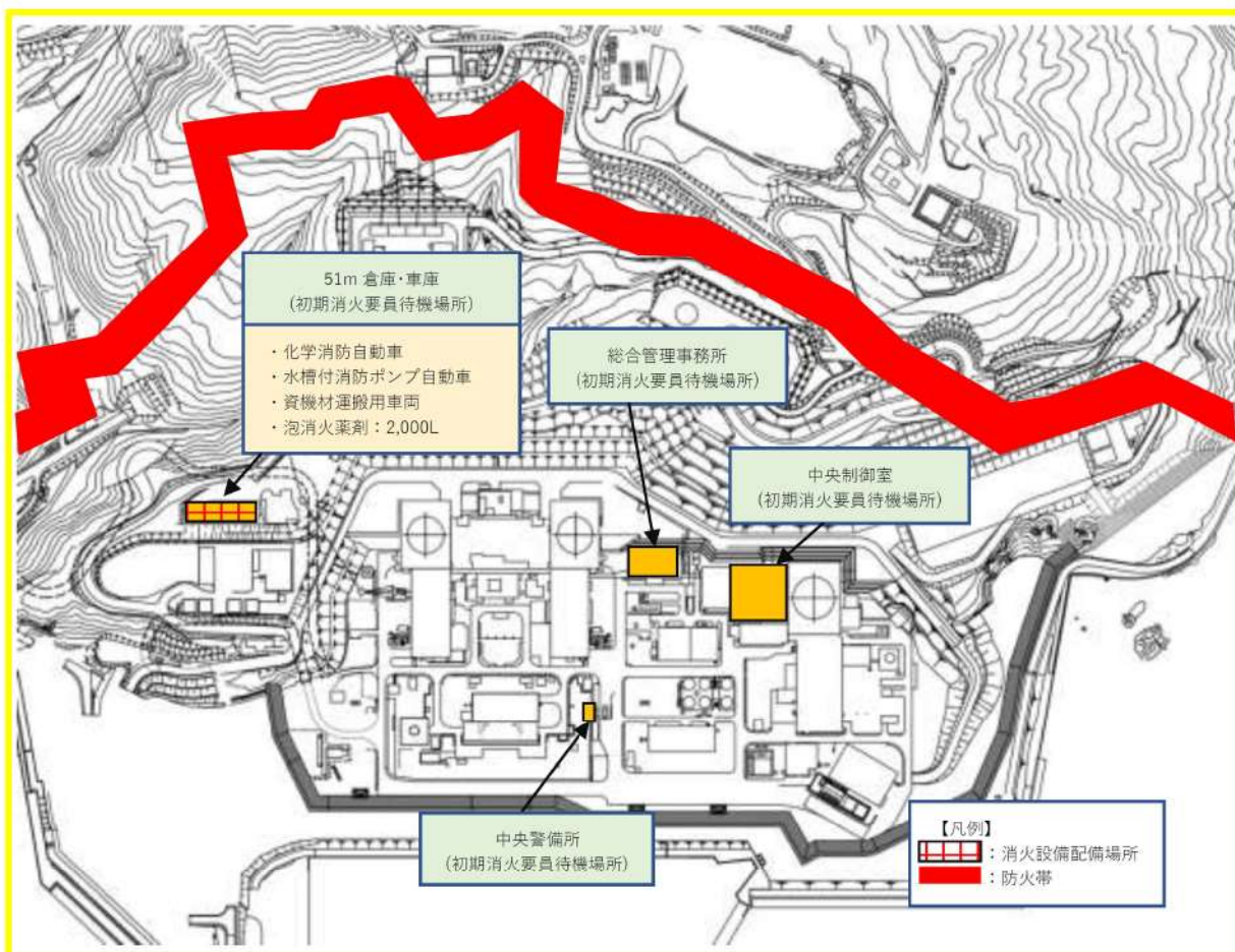
第 1-16 図：移動式消火設備の配置の概要
