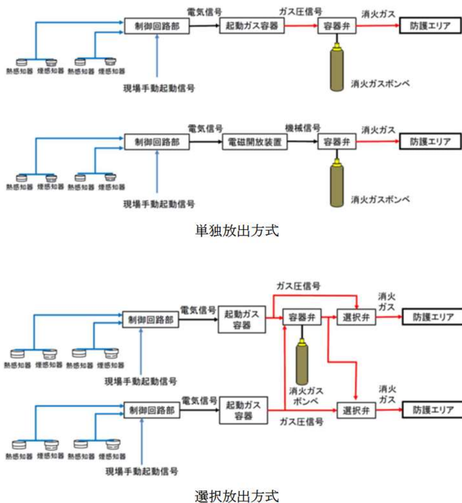
第1-14図：系統分離に応じた独立性を考慮した消火設備の概要図
