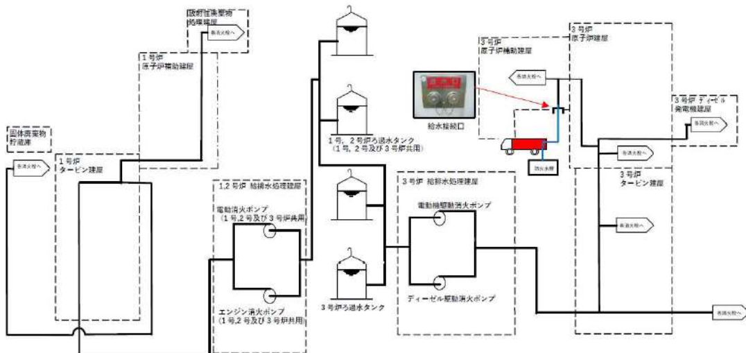
第 1-22 図：給水接続口接続概要図
