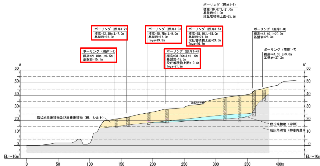
A-A' 断面
