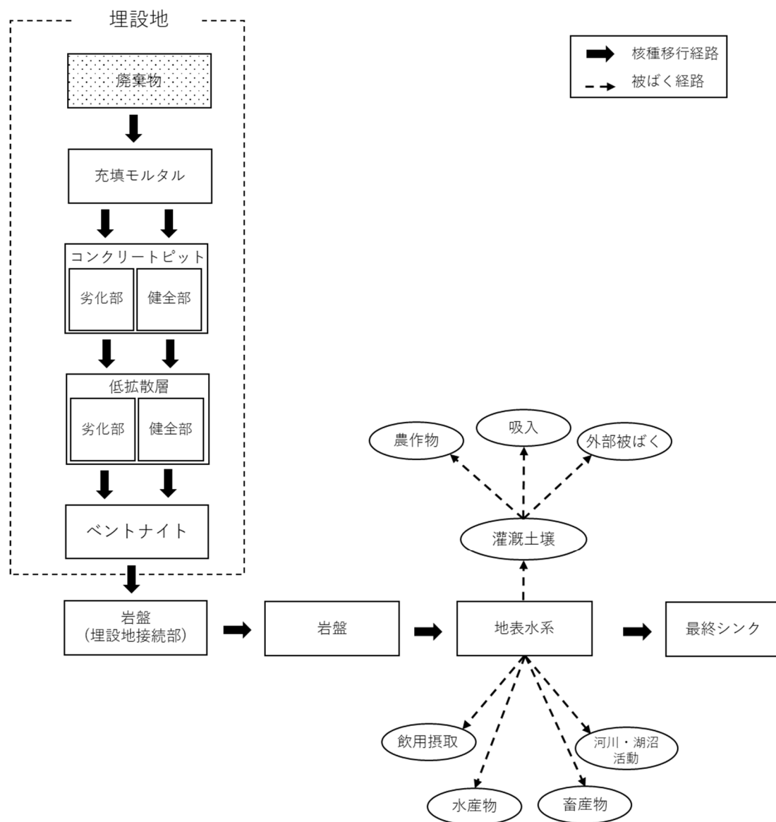
図5 中深度処分評価モデルの概念図
