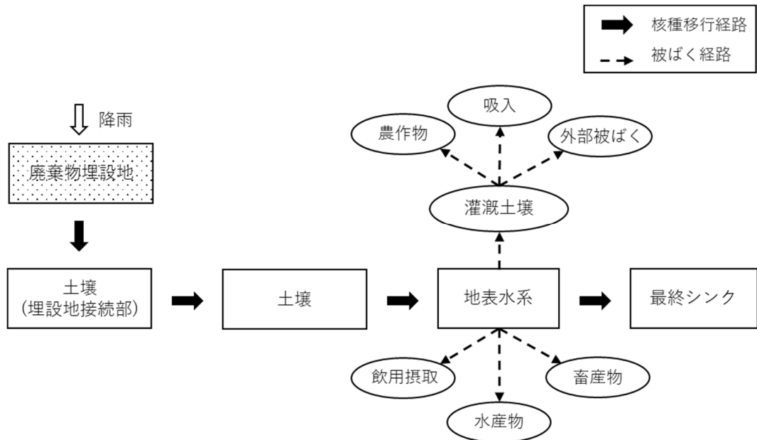
図3 トレンチ処分評価モデル概念図
