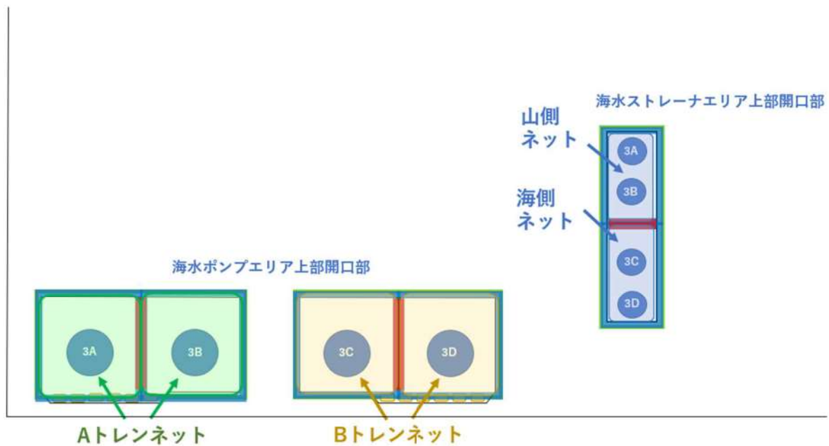
図3 竜巻防護ネット 平面図
