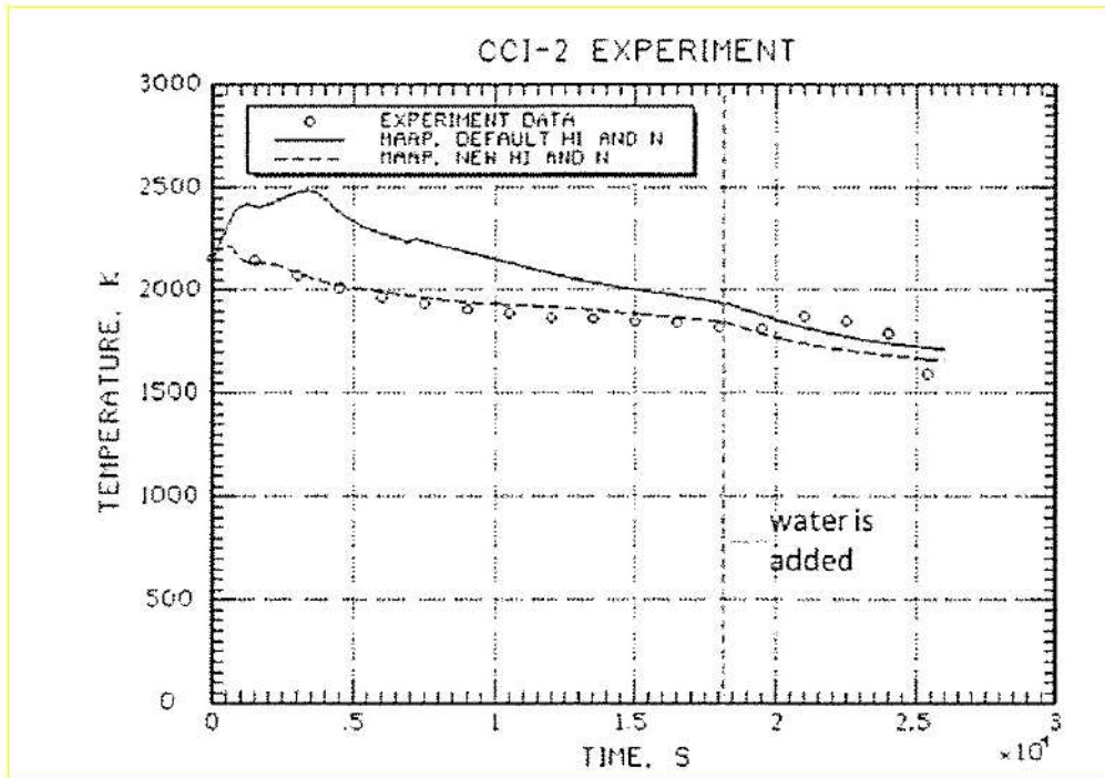
図 3.1-41 CCI-2 実験のコリウム温度の実験データと MAAP 解析結果の比較 MAAP New 熱伝達係数 (破線) : 床面方向 300\text{W}/\text{m}^2/\text{K} , 壁面方向 300\text{W}/\text{m}^2/\text{K} , n=0 )
