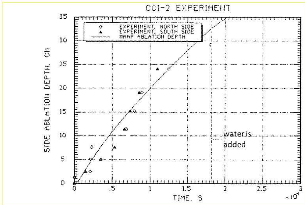
図 3.1-43 CCI-2 実験の壁面方向侵食の実験データと MAAP 解析結果の比較
