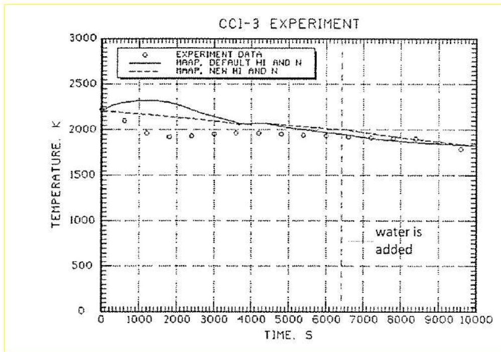
図 3.1-44 CCI-3 実験のコリウム温度の実験データと MAAP 解析結果の比較
