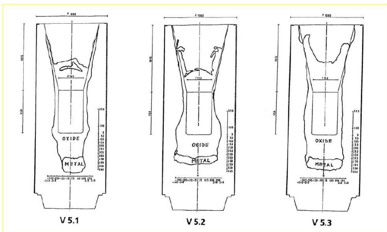
図 3.1-57 BETA 試験 実験後のコンクリート侵食状況を示す模式図
