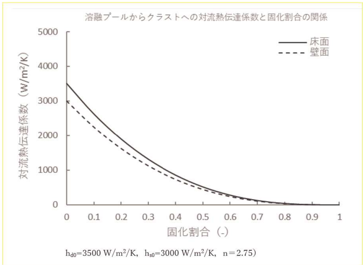
図 3.1-40 溶融プールからクラストへの対流熱伝達係数
