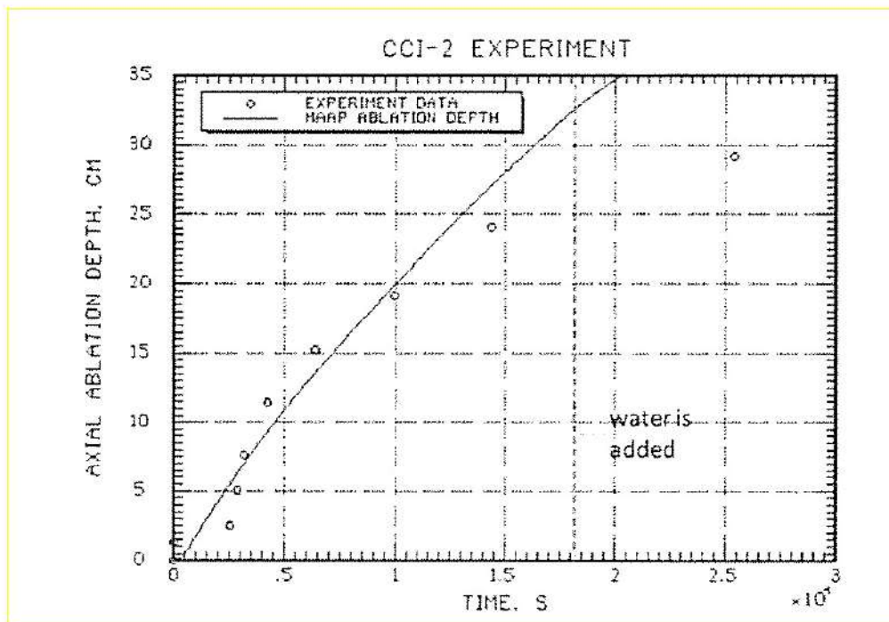
図 3.1-42 CCI-2 実験の床面方向侵食の実験データと MAAP 解析結果の比較
