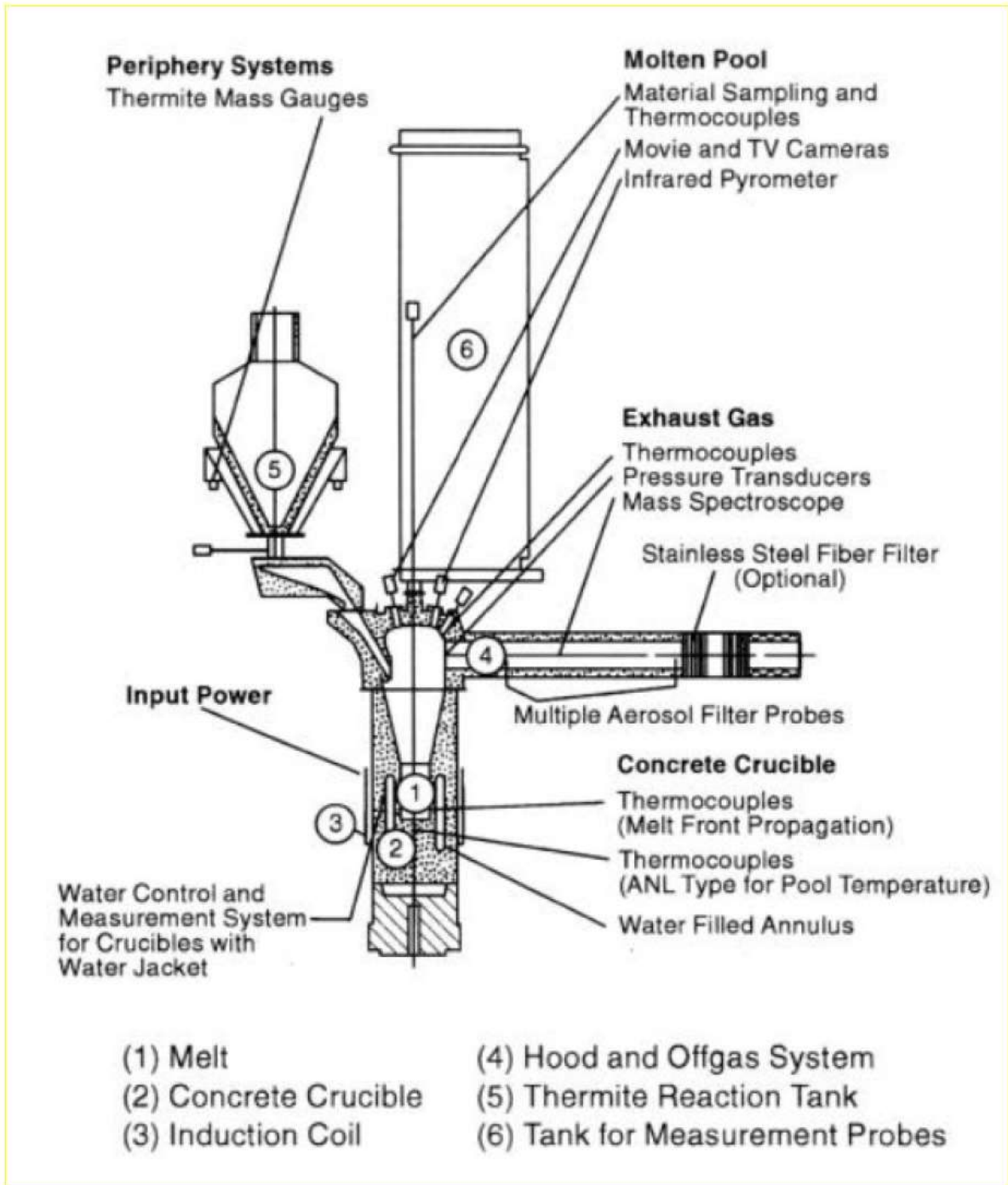
图 3.1-56 BETA 試驗 實驗裝置
