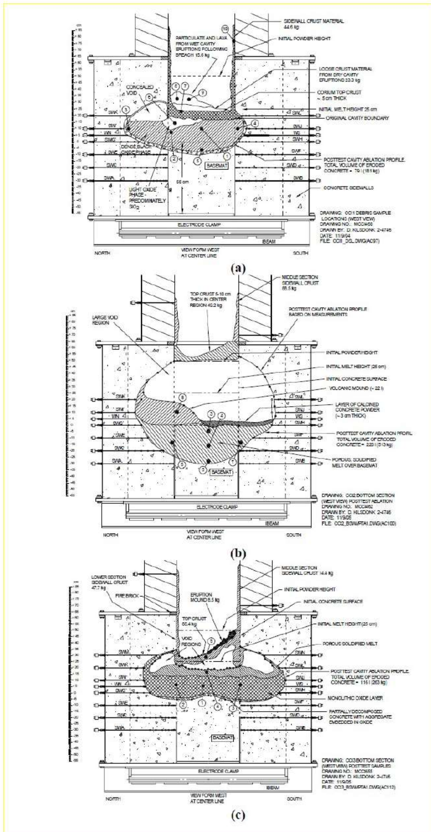
図 3.1-39 CCI 実験における侵食状態の模式図
