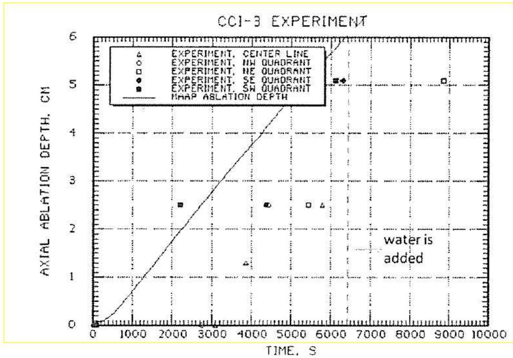
図 3.1-45 CCI-3 実験の床面方向侵食の実験データと MAAP 解析結果の比較
