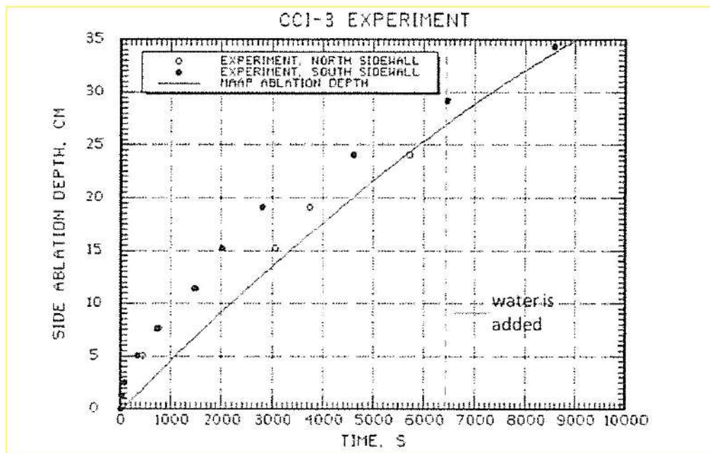
図 3.1-46 CCI-3 実験の壁面方向侵食の実験データと MAAP 解析結果の比較
