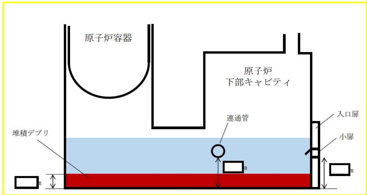
図1 原子炉下部キャビティ堆積デブリ状況
