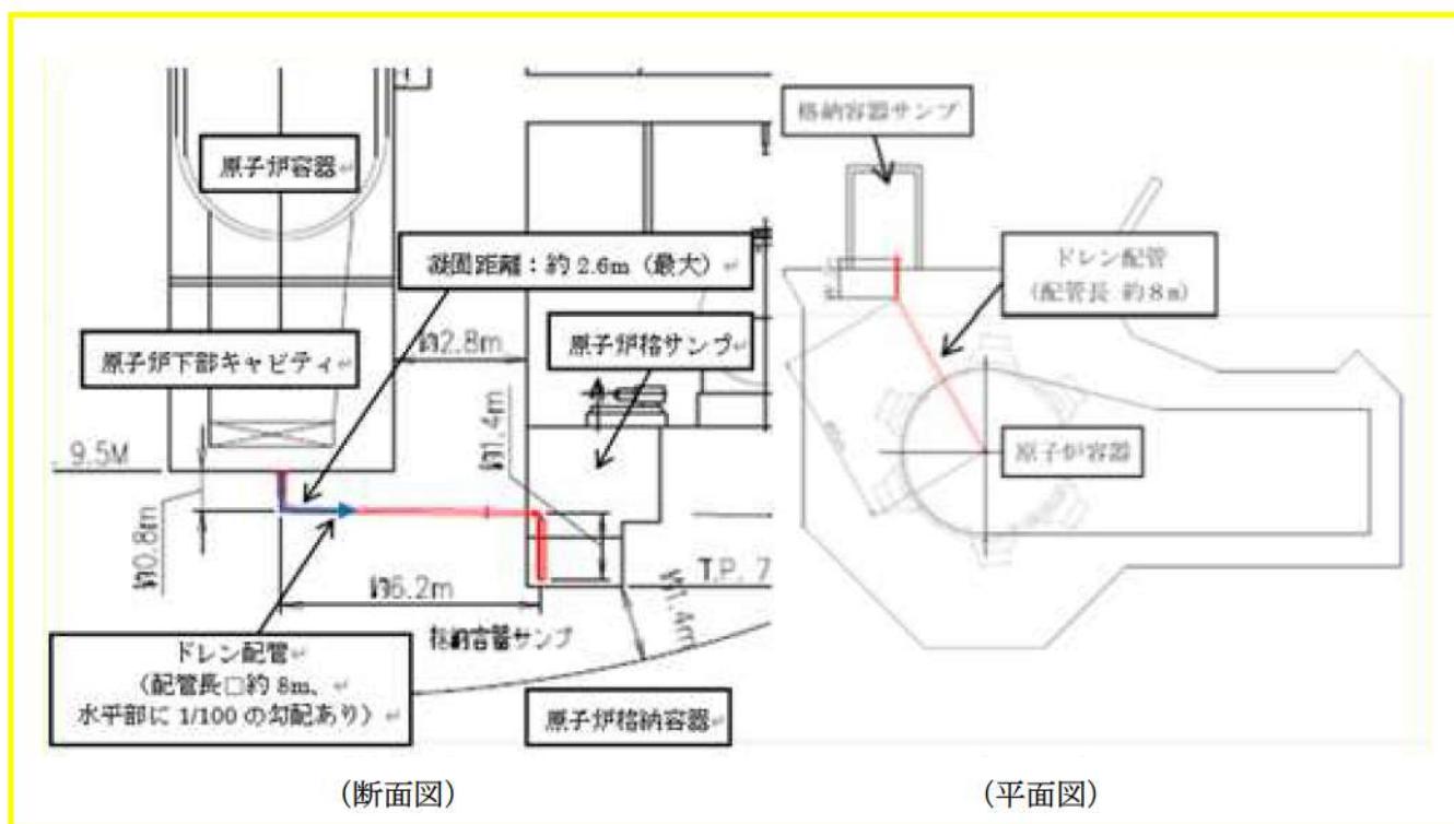
図1 原子炉格納容器の構造図
