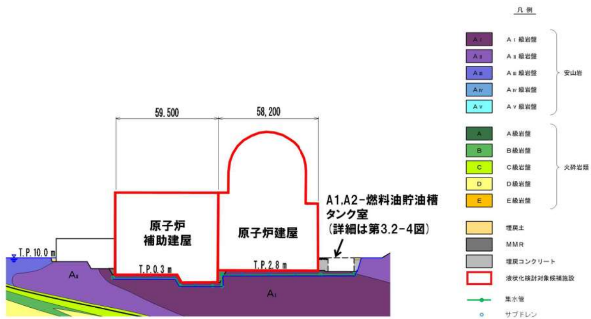
第 3.2-1 図 原子炉建屋，原子炉補助建屋，A1, A2-燃料油貯油槽タンク室断面図(①-①')
