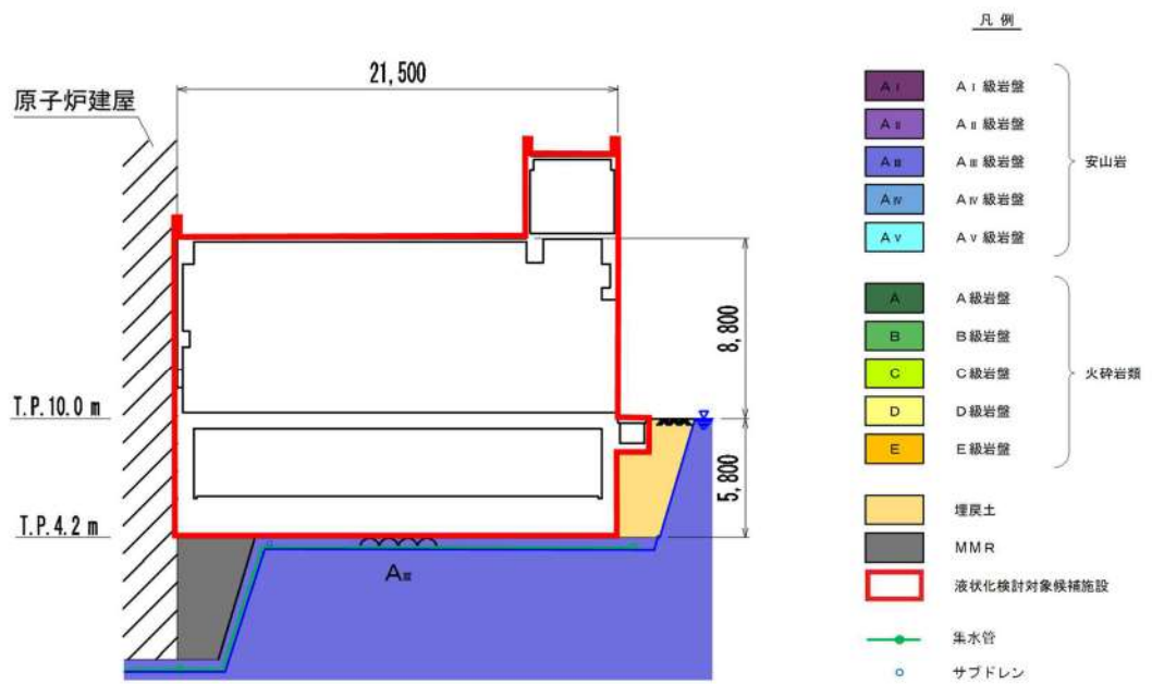
第 3.2-3 図 ディーゼル発電機建屋断面図
