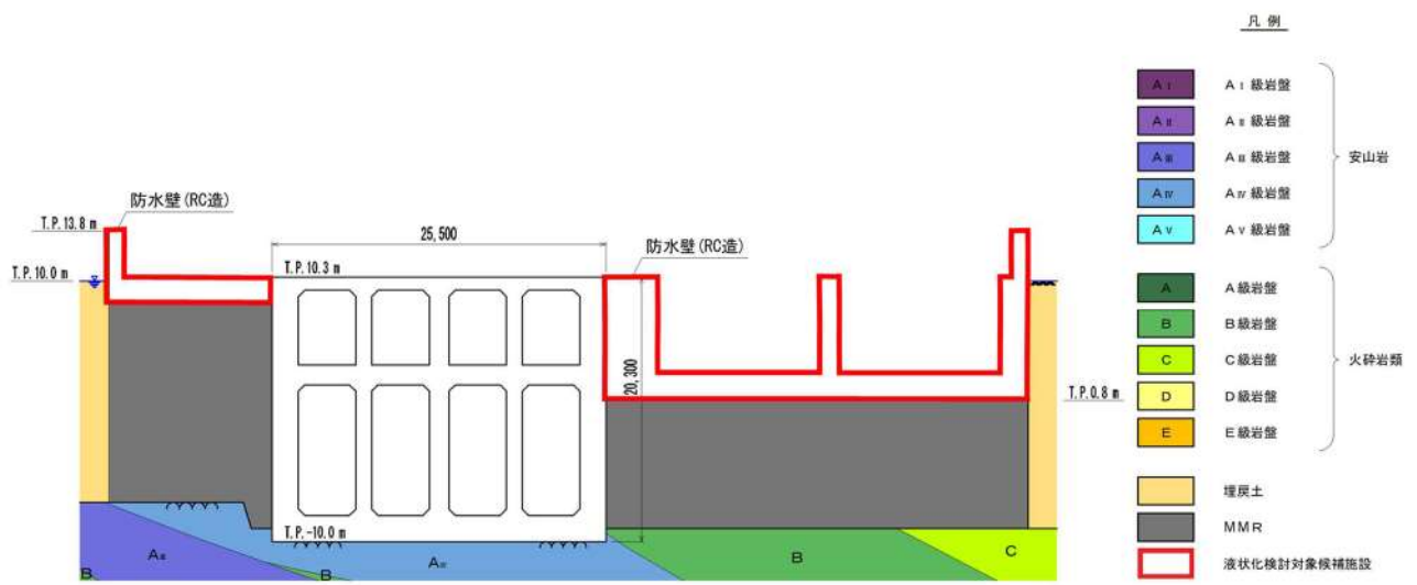
第 3.2-14 図 3号炉取水ピットスクリーン室防水壁断面図
