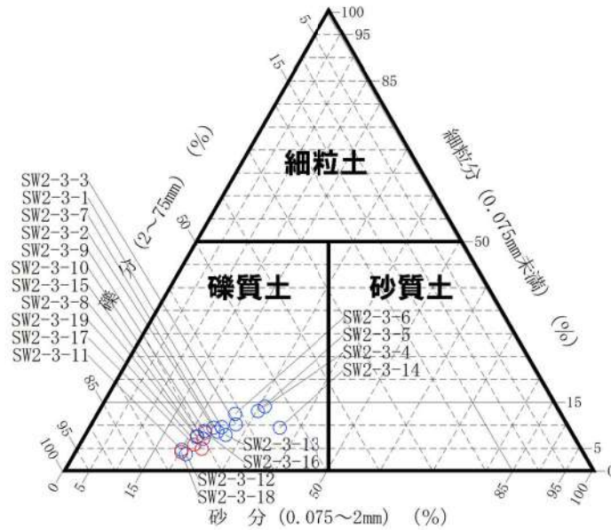
添付 8-4 図 三角座標による分類 (SW2-3)
