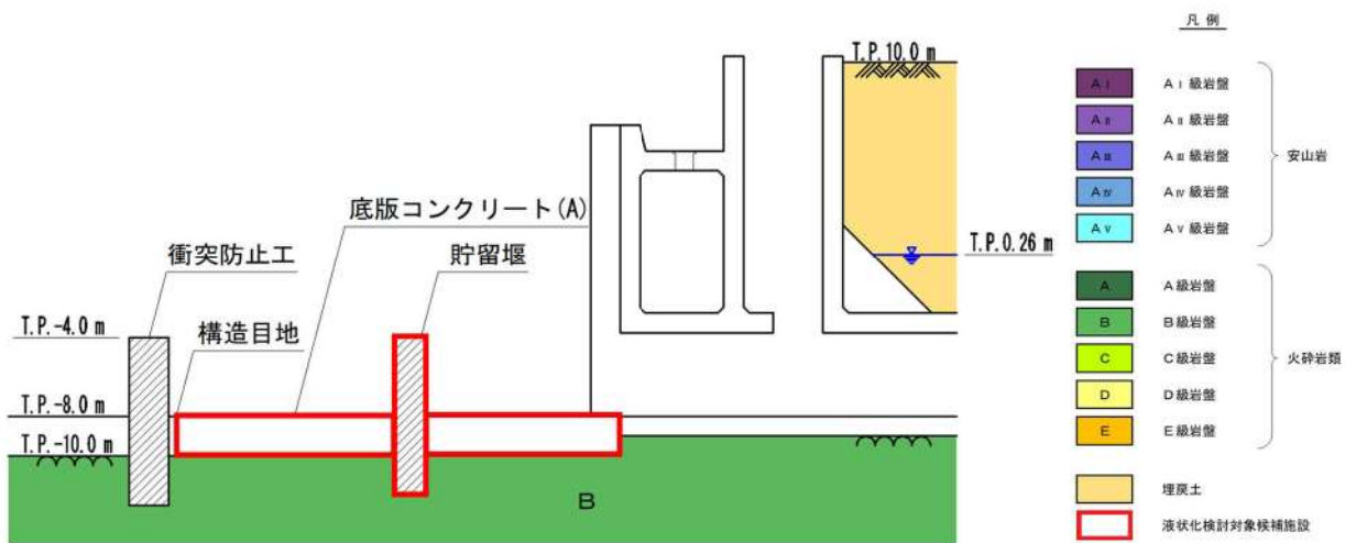
第 3.2-19 図 貯留堰部断面図
