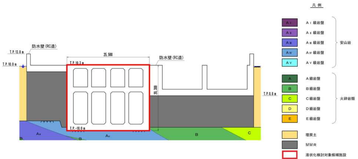
第 3.2-8 図 取水ピットスクリーン室断面図
