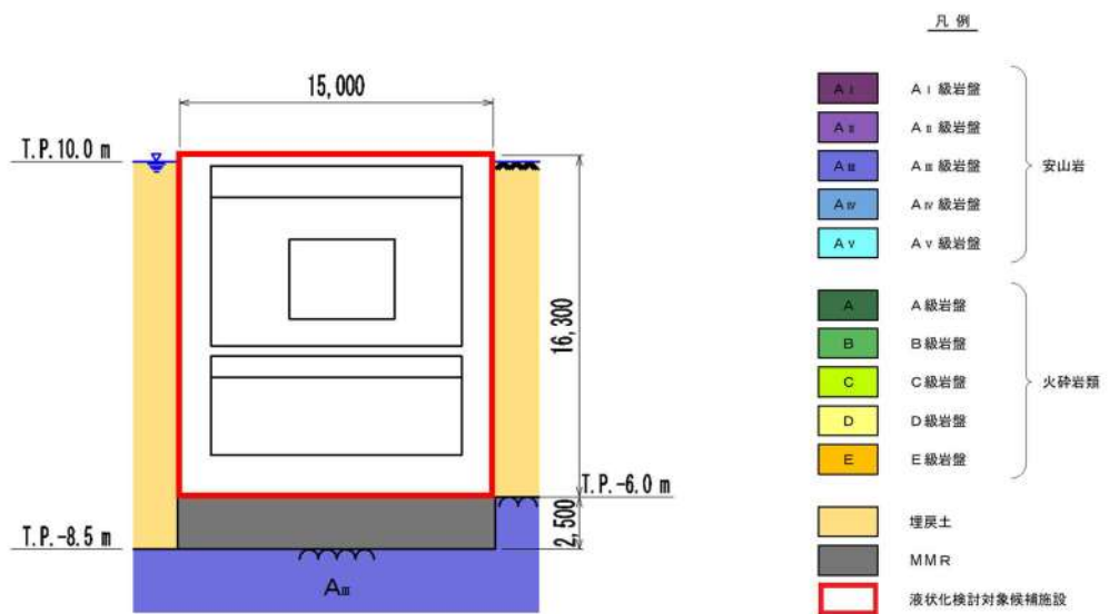
第 3.2-10 図 原子炉補機冷却海水ポンプ出口ストレーナ室断面図
