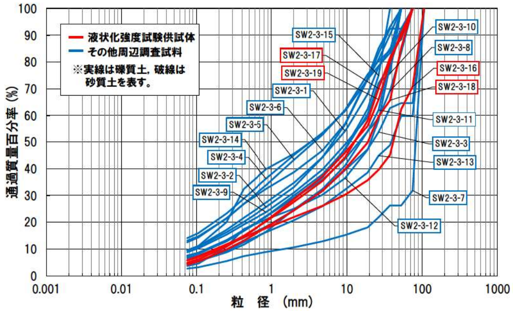
添付 8-3 図 粒度分布 (SW2-3)
