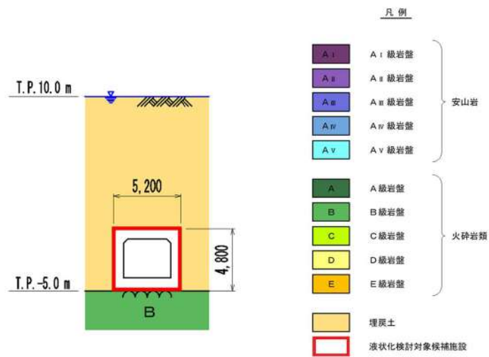
第 3.2-11 図 原子炉補機冷却海水管ダクト断面図
