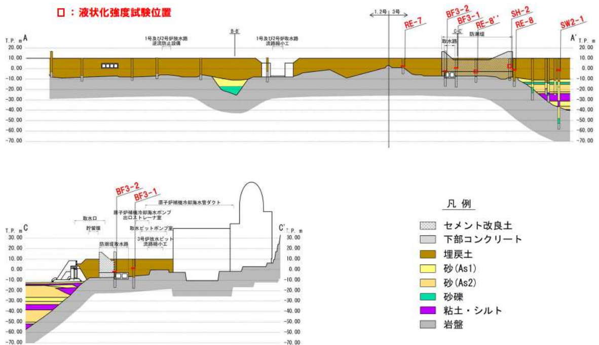
第 4.2-3 図 液状化強度試験に用いる試料採取位置断面図(3号埋戻土)
