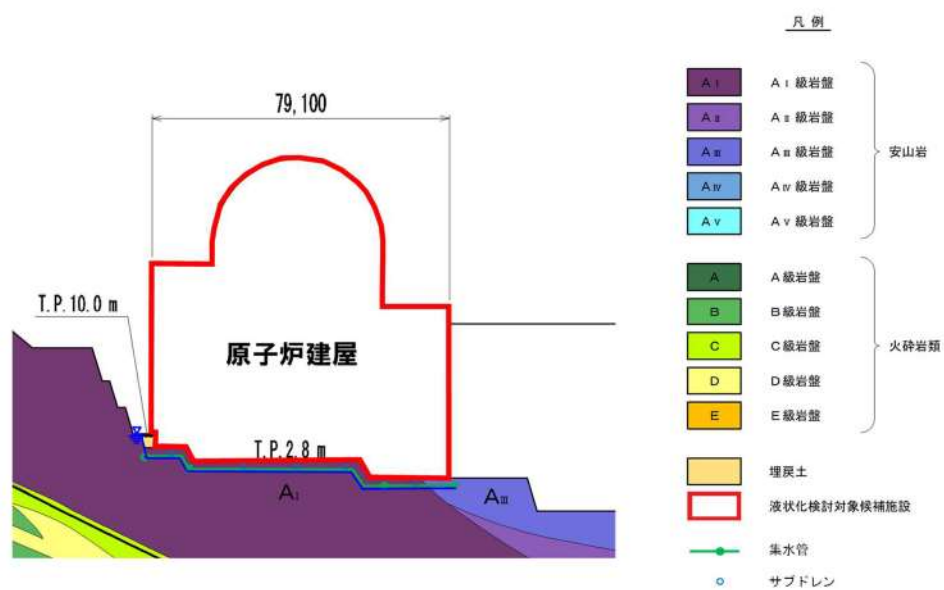
第 3.2-2 図 原子炉建屋断面図(②-②')
