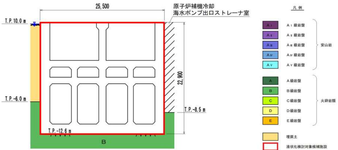
第 3.2-9 図 取水ピットポンプ室断面図
