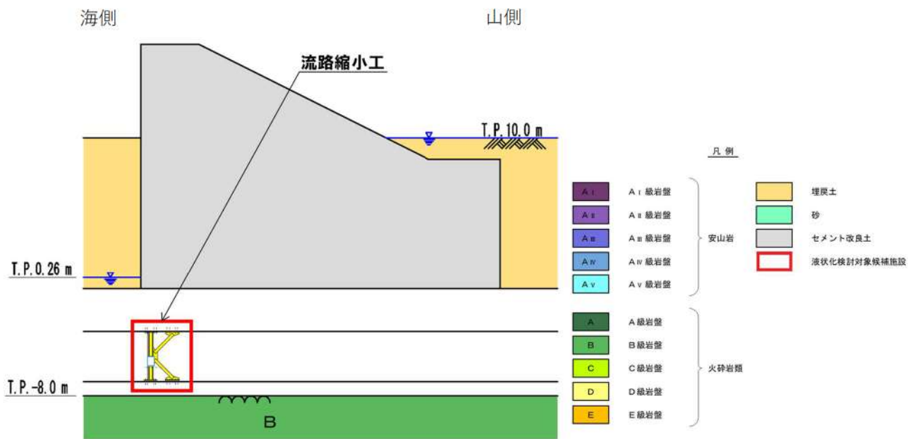
第 3.2-17 図 1 号及び 2 号炉取水路流路縮小工断面図
