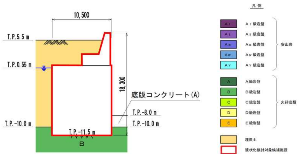
第 3.2-6 図 取水口断面図
