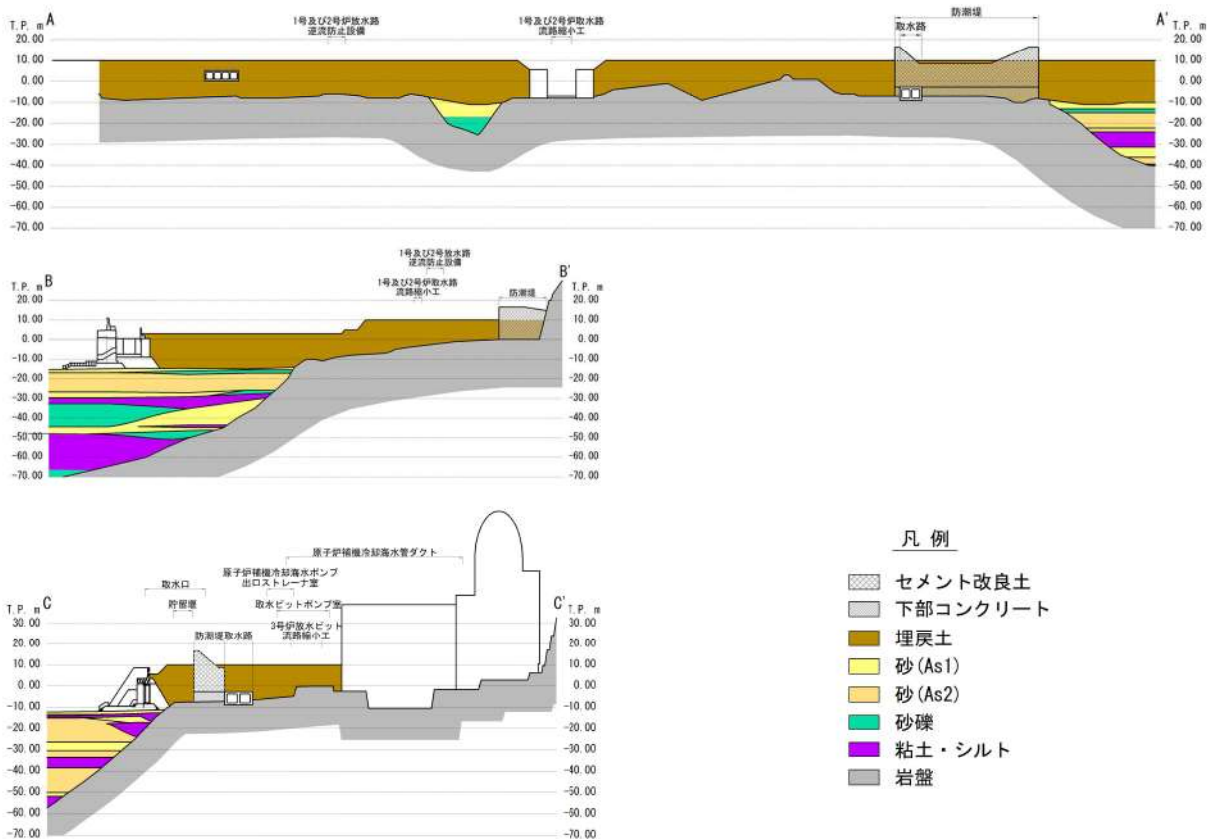
第 2.1-3 図 地質断面図
