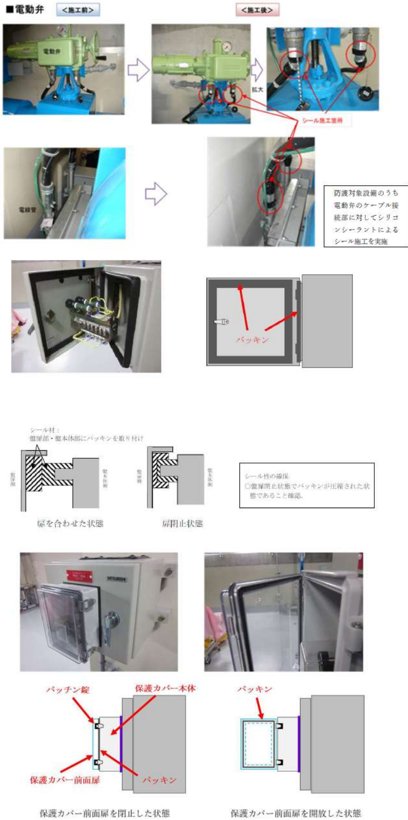
図2 現場での被水状況を考慮した被水対策について
