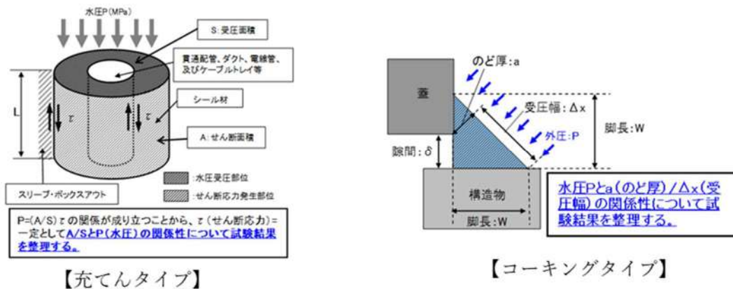
図 9 シリコンシーラント及び充てんシリール材の耐水圧試験概要図
