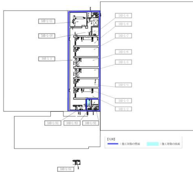
図 1 溢水防護対策施工対象の壁及び床の配置図 (10/11)
