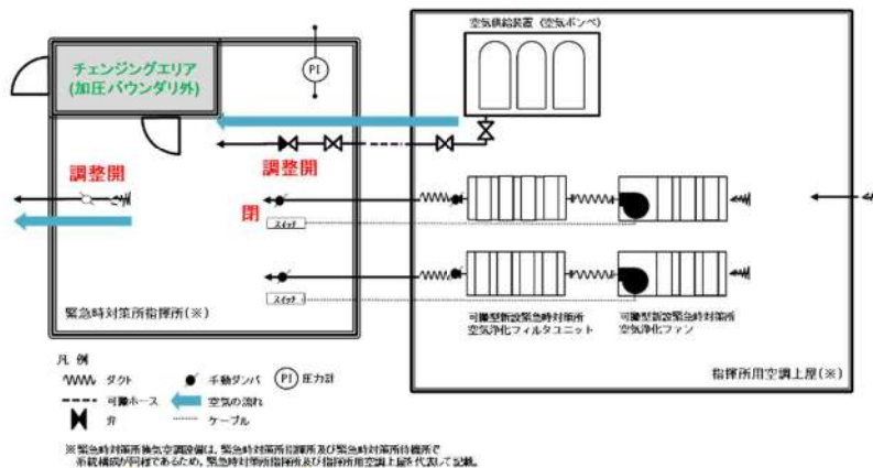
緊急時対策所空気供給装置による正圧化時の気密性, 正圧化機能に関する試験・検査性 概略図 (プルーム通過中)
