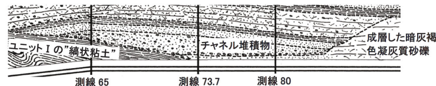
自衛隊駐屯地の露頭に認められるSpflの軽石を含むチャンネル堆積物 (Spflの再堆積層と解釈) (井上ほか,2022)
