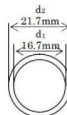
図2 配管断面図
