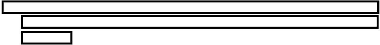
第2図 B-使用済燃料ピットに実運用を考慮した体数のウラン・プルトニウム混合酸化物新燃料及びウラン新燃料を貯蔵した場合の計算体系(水平方向, B-使用済燃料ピット全体)
