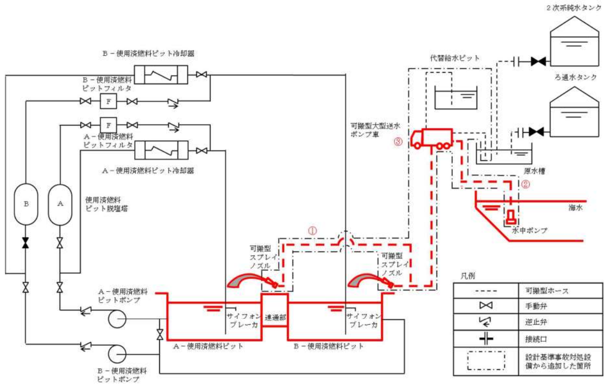
図 54-4-2 使用済燃料ピットへのスプレィ
