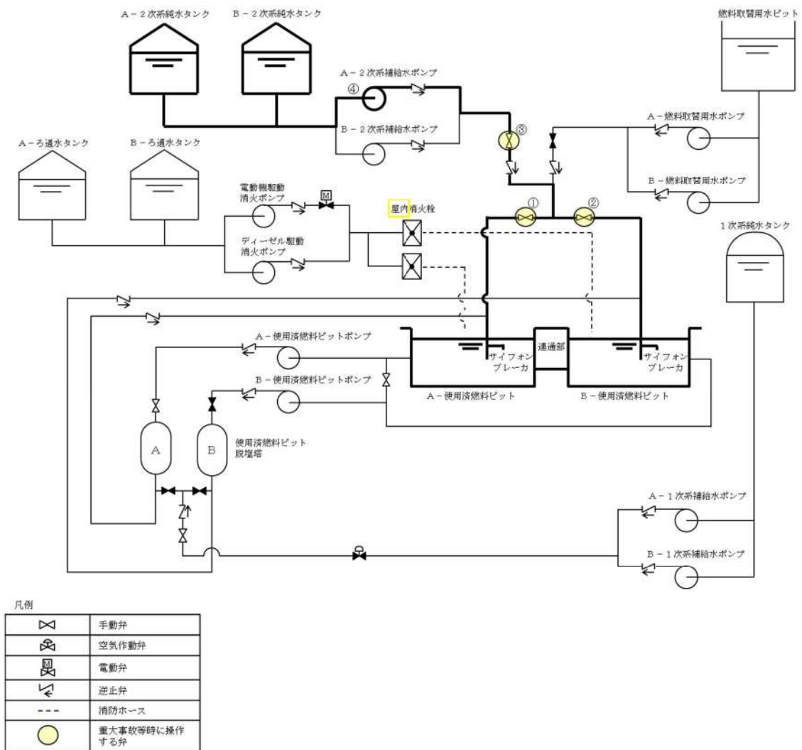
図 54-16-2 2次系補給水ポンプによる使用済燃料ピットへの注水の概要図
