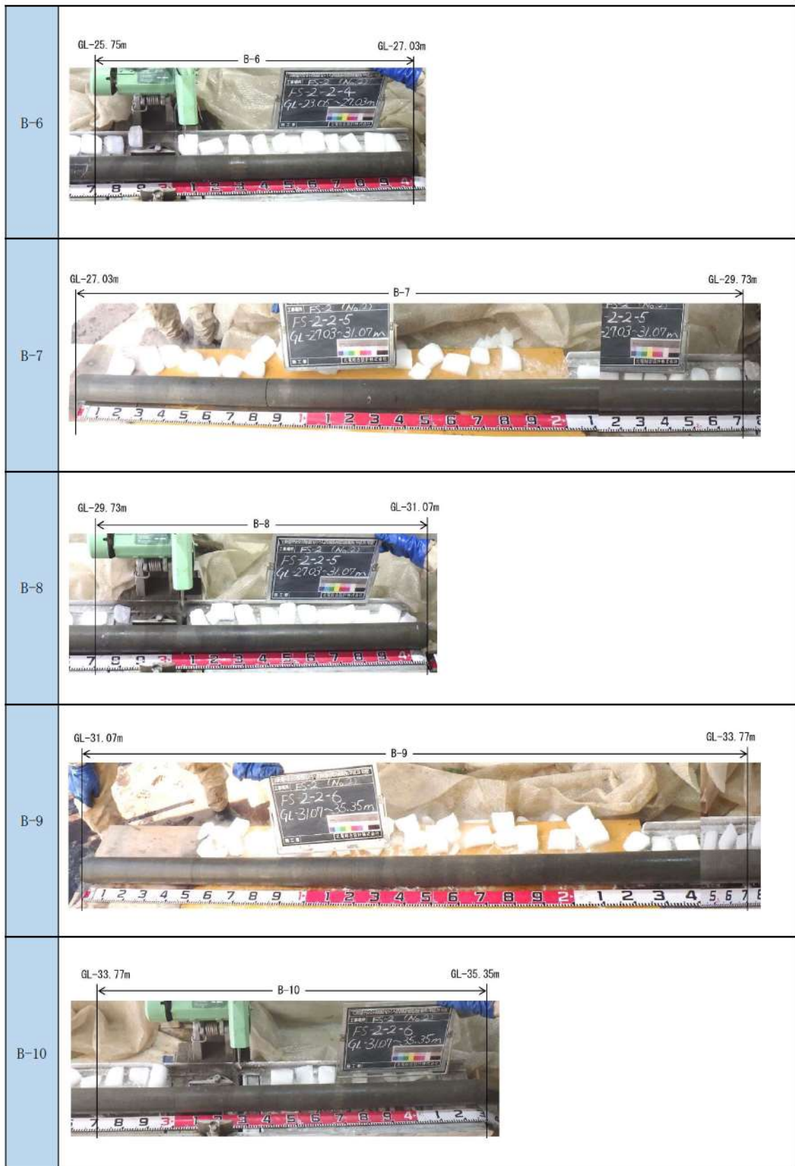
添付 1-34 図(6/10) ボーリング柱状図・コア写真 (FS-2)
