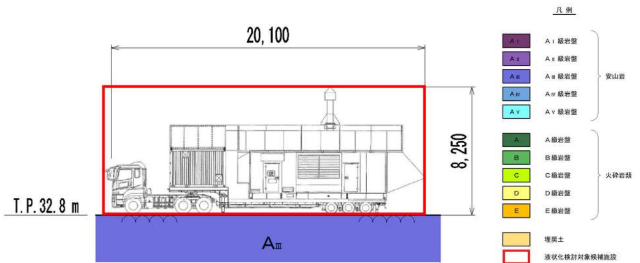
第 3.2-21 図 代替非常用発電機設置位置断面図
