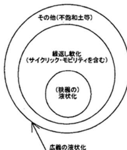
第 5.2-1 図 液状化に関連する言葉の定義
