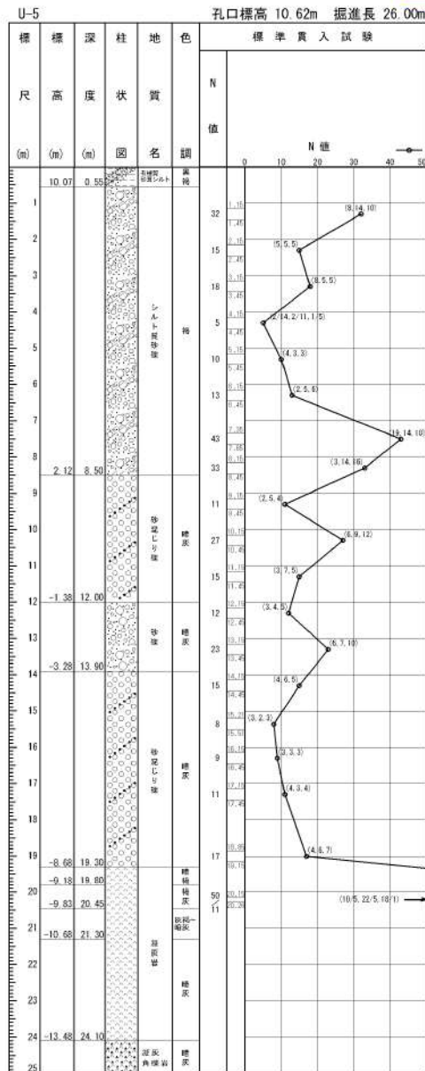
添付 1-13 図(1/2) ボーリング柱状図・コア写真 (U-5)
