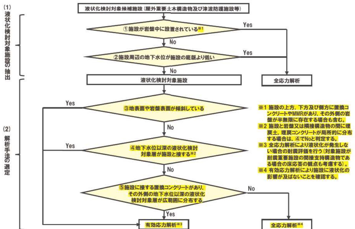
第 3.1-2 図(2) 液状化検討対象施設の選定及び解析手法選定フロー (屋外重要土木構造物及び津波防護施設等)
