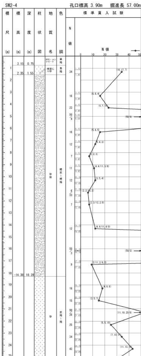
添付 1-53 図(1/3) ボーリング柱状図・コア写真 (SW2-4)
