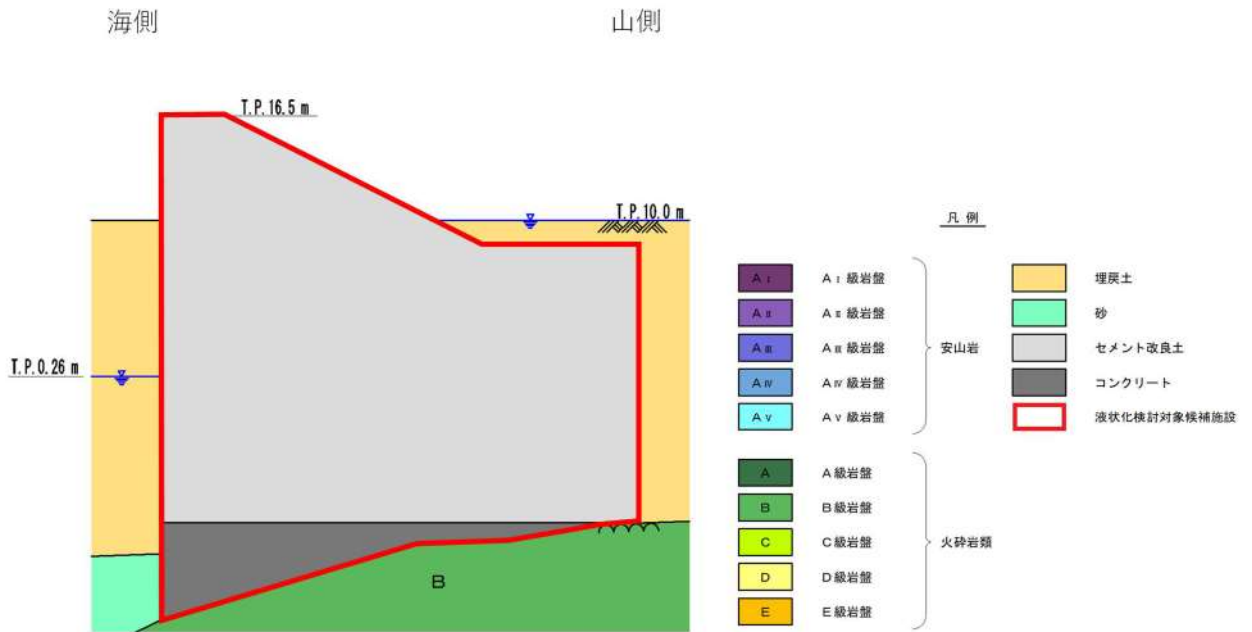
第 3.2-13 図 防潮堤断面図
