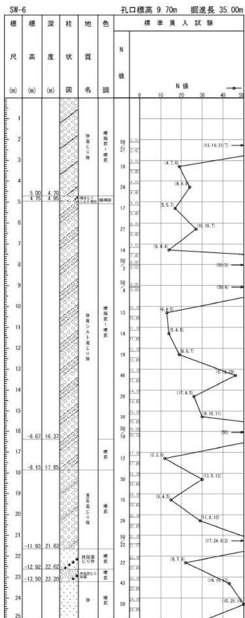
添付 1-36 図(1/2) ボーリング柱状図・コア写真 (SW-6)
