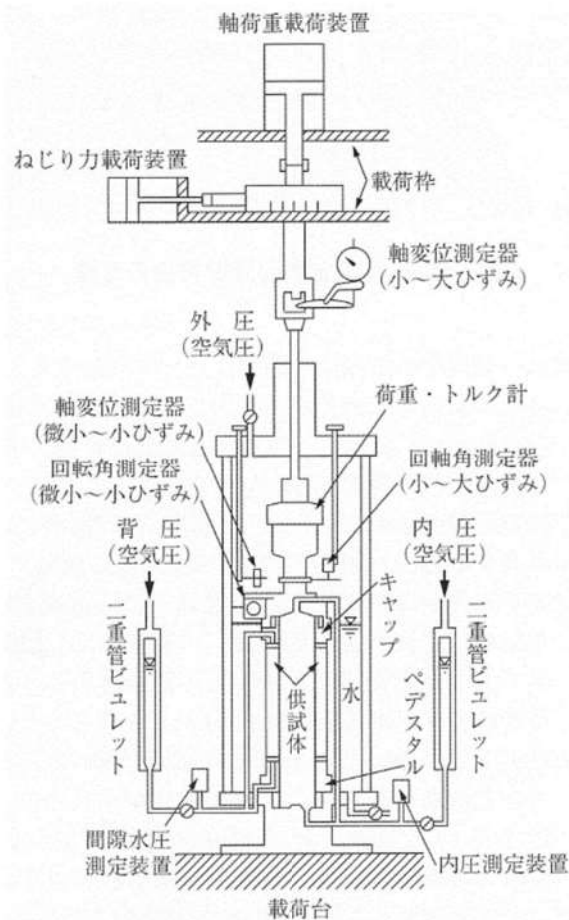
第 5. 1-1 図 繰返し非排水三軸試験装置の概要
