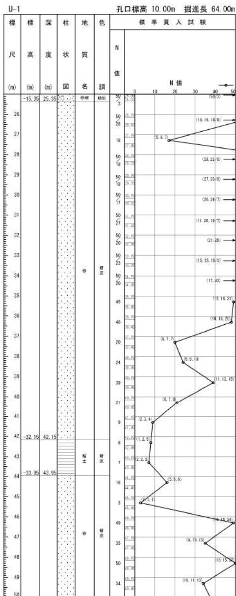
添付 1-41 図(2/3) ボーリング柱状図・コア写真 (U-1)
