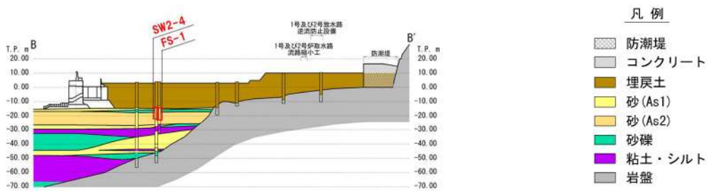
第 4.2-5 図 液状化強度試験に用いる試料採取位置断面図(砂層)
