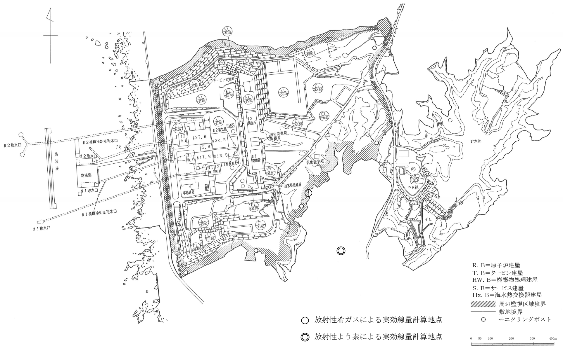
第1図 実効線量計算地点図
