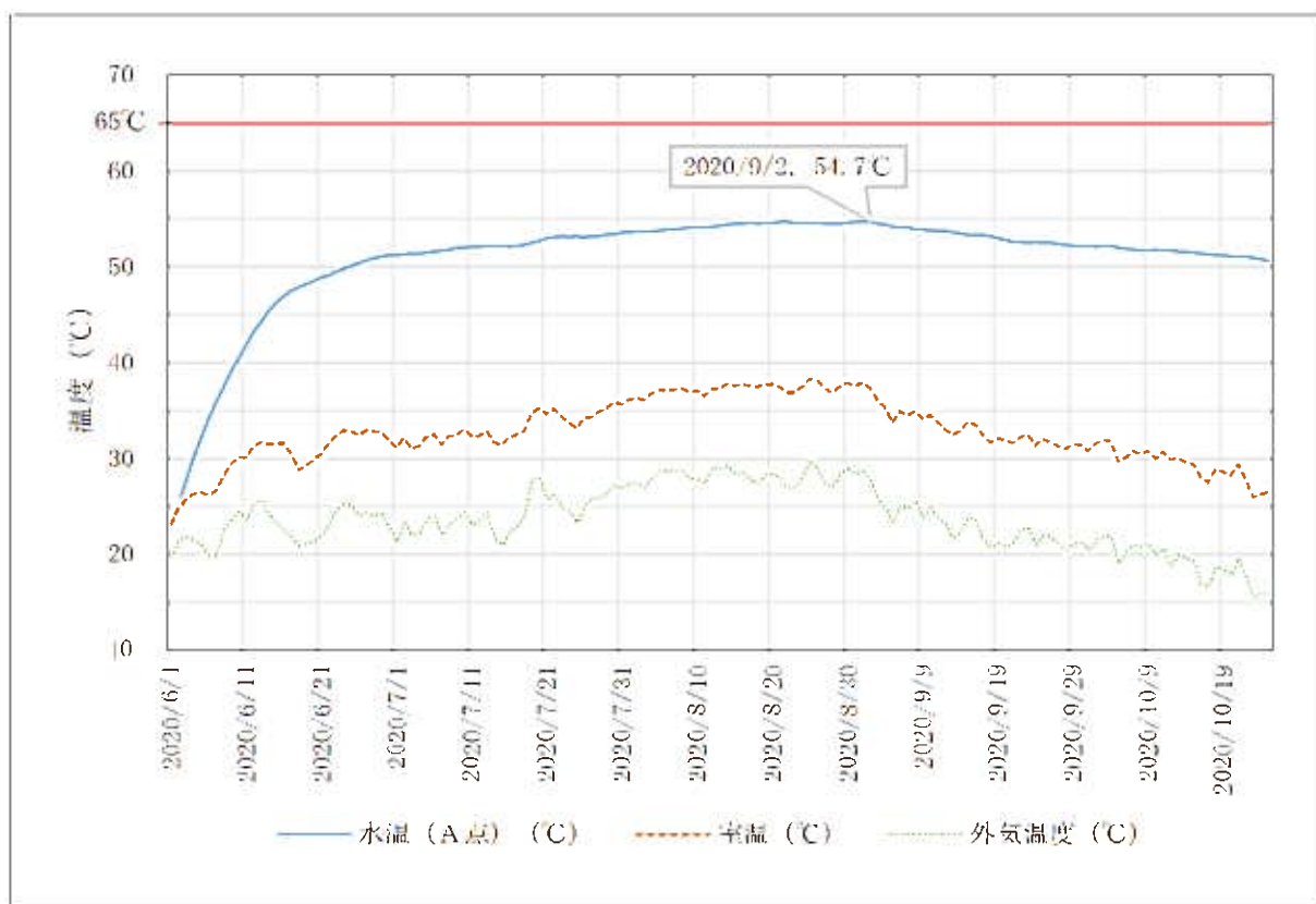
第4図 水温測定結果
