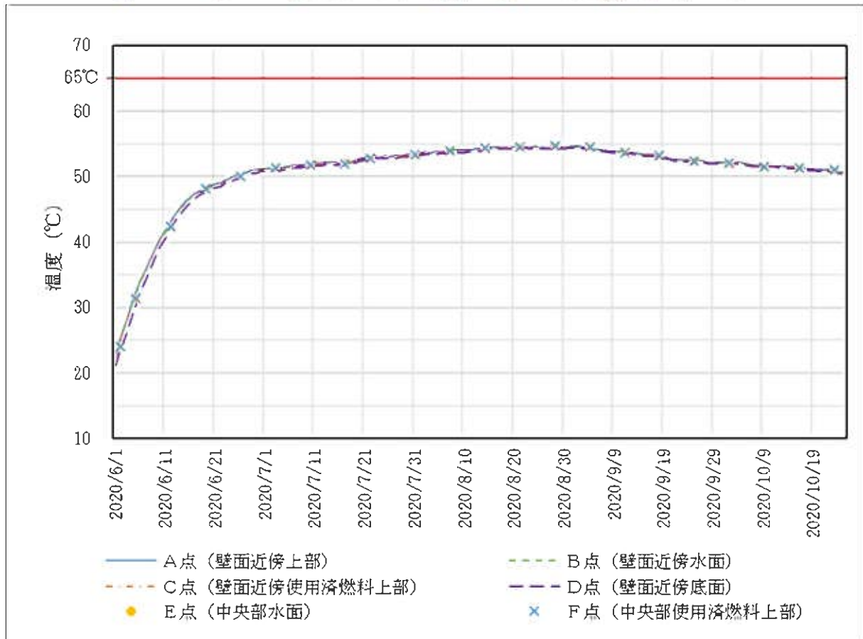
第5図 水温測定結果 (A点～F点)
