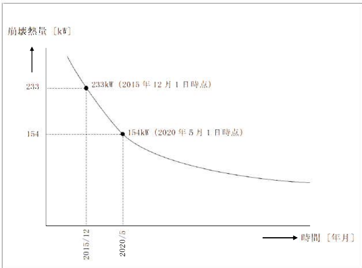
第1図 玄海1号炉使用済燃料ピット内の使用済燃料の崩壊熱推移
