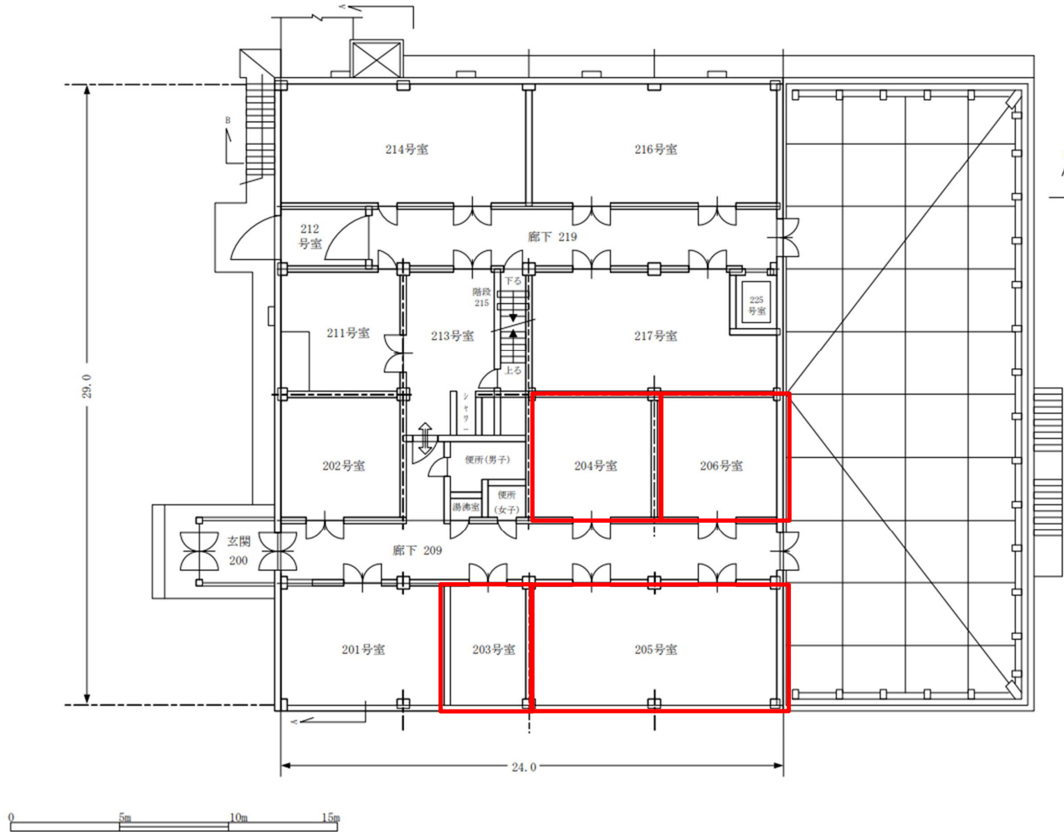
開発試験棟1階の平面図
