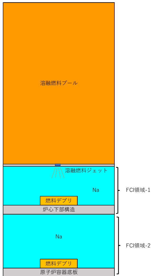
図1 ADYTUM による ULOF 時の溶融燃料挙動解析モデルの概念
