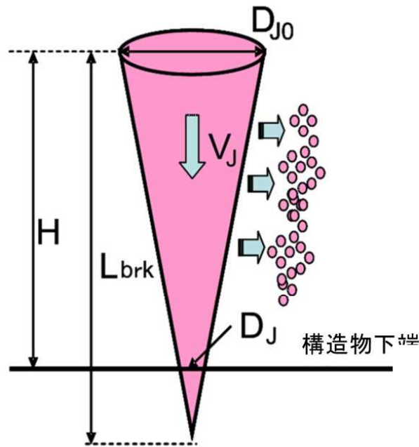
図2 ジェットブレイクアップモデル
