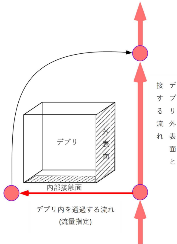
図4 デブリ冷却モデルの概念
