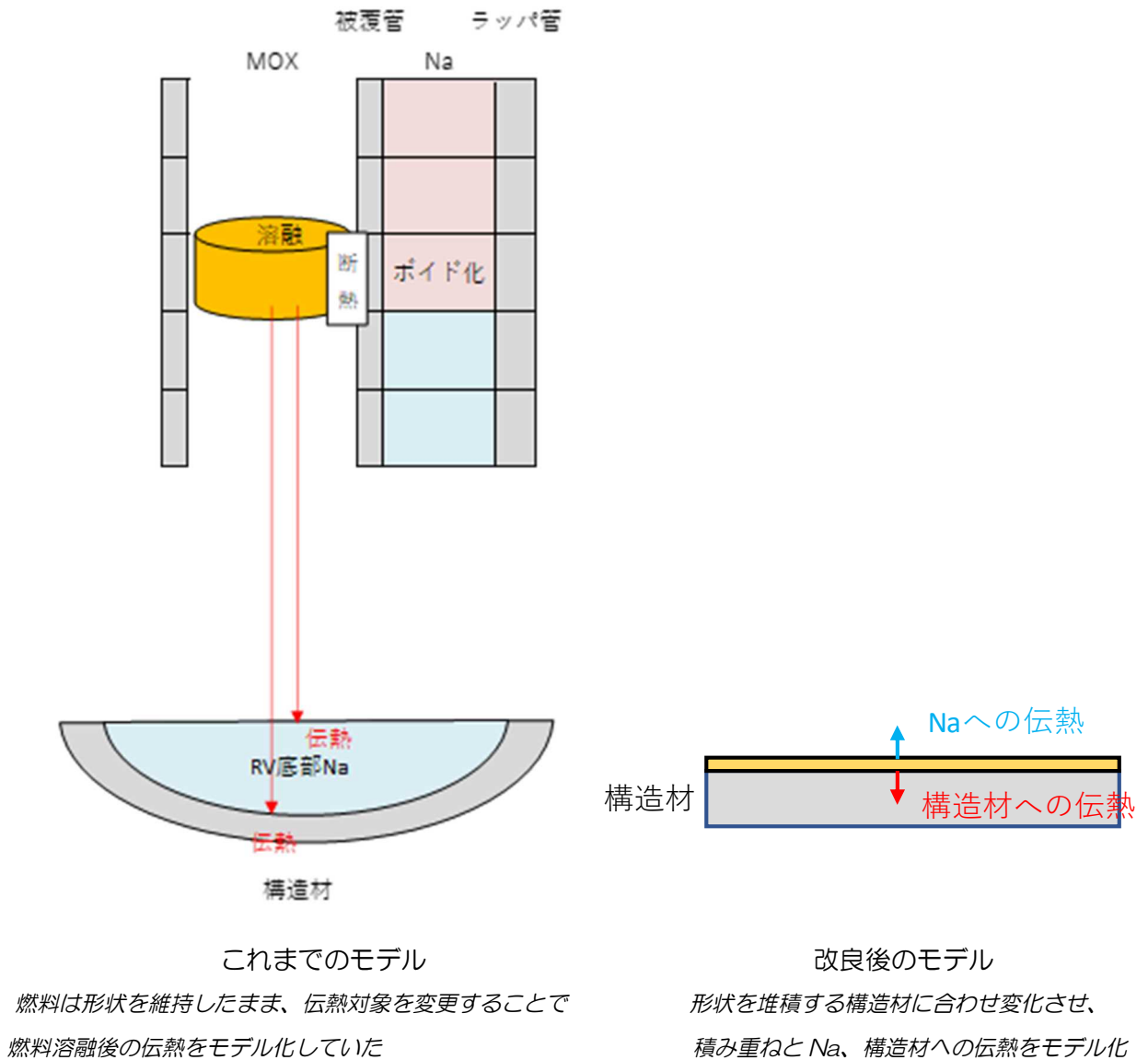
図3 燃料溶融時の解析モデルの改良
