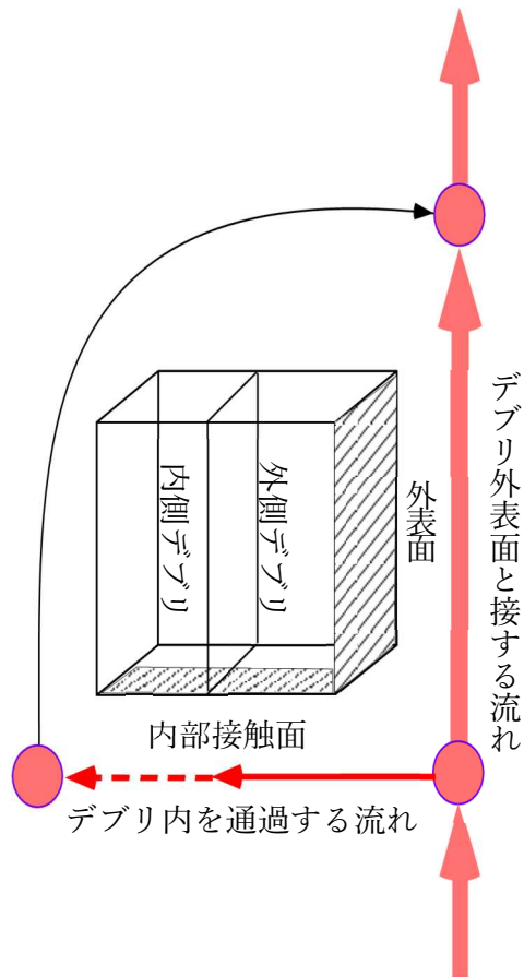
図5 デブリ冷却モデル（デブリ2領域モデル）の概念
