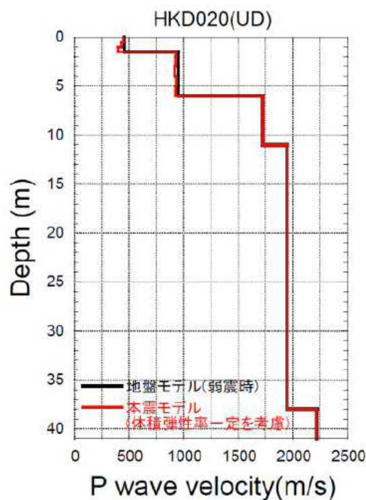
P波速度
