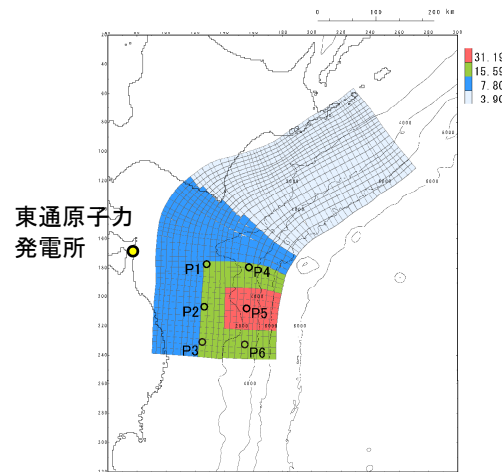
基準断層モデル②
