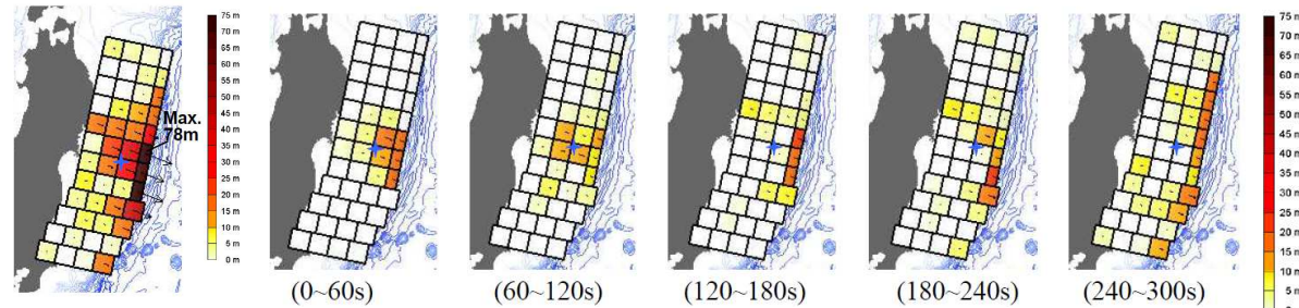
すべり量分布(合計) (確定波源モデル)
