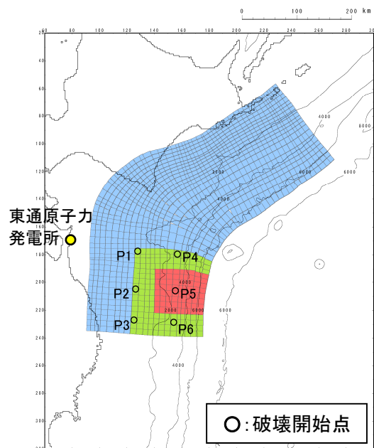
基準断層モデル①
