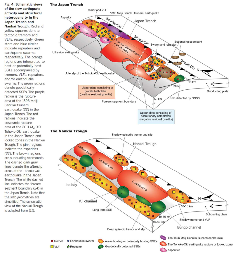
日本海溝および南海トラフにおけるスロー地震活動と構造的不均質性の関係(概略図) (Nishikawa et al. (2019))
