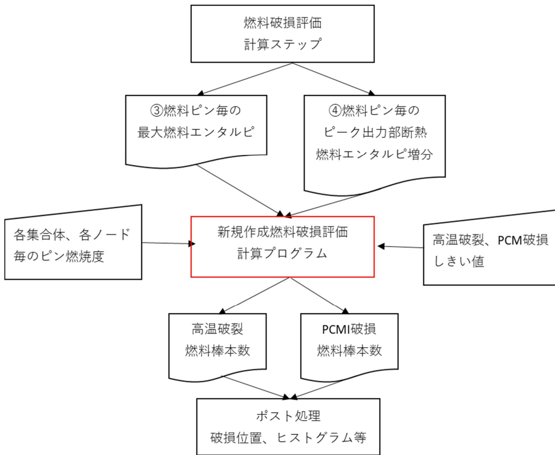
図3 燃料破損評価コードを用いた燃料破損本数（破損モードを含む。）及び燃料破位置評価並びに事後処理の流れ
