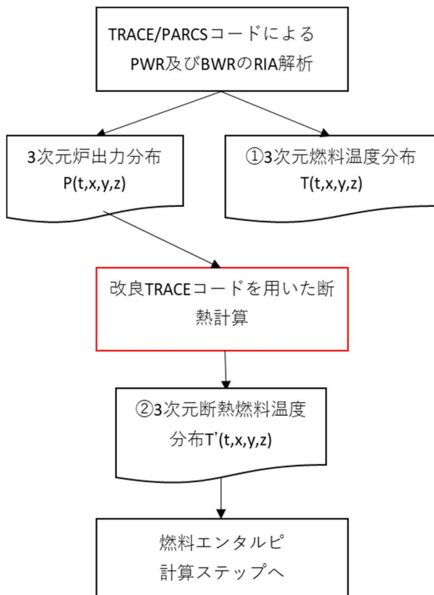
図1 改良 TRACE コードを用いた 3次元断熱燃料温度分布評価の流れ
