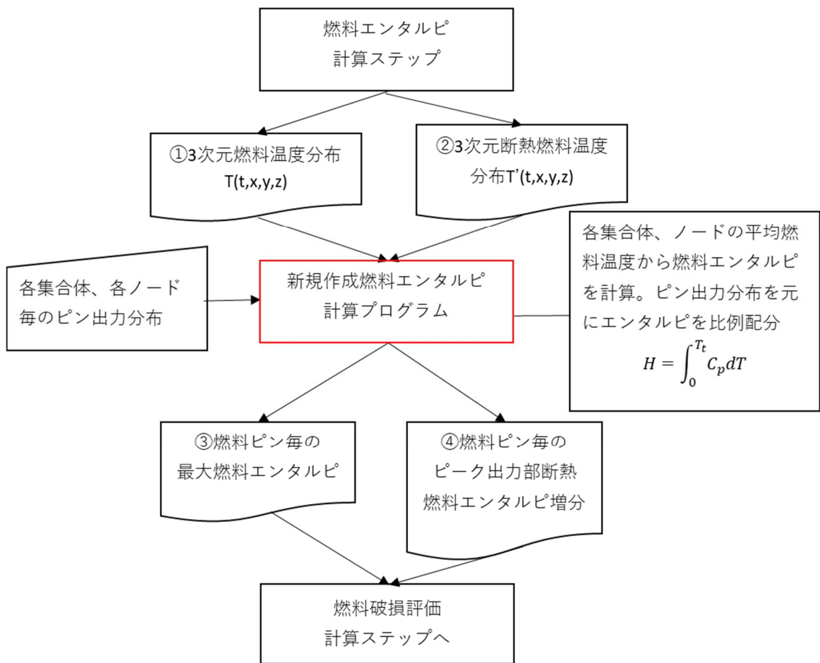
図2 燃料棒毎の最大燃料エンタルピー及びピーク出力部断熱燃料エンタルピー増分の評価の流れ
