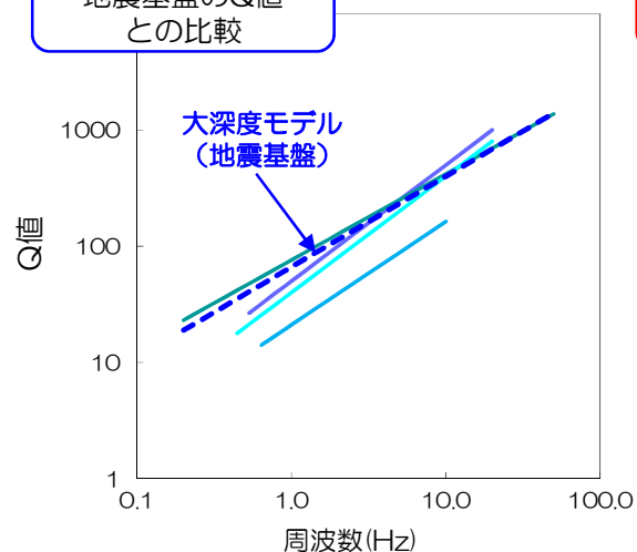
地震基盤以浅のQ値との比較
