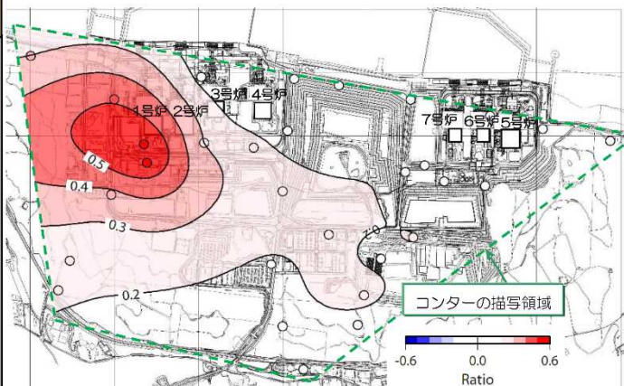
水平アレイ観測記録に基づく 敷地南西側から到来する地震波が増幅する領域 注) コンターは観測点間で補間しており、観測点がない端部は外挿となるため 緑点線以内の領域を描写している。
