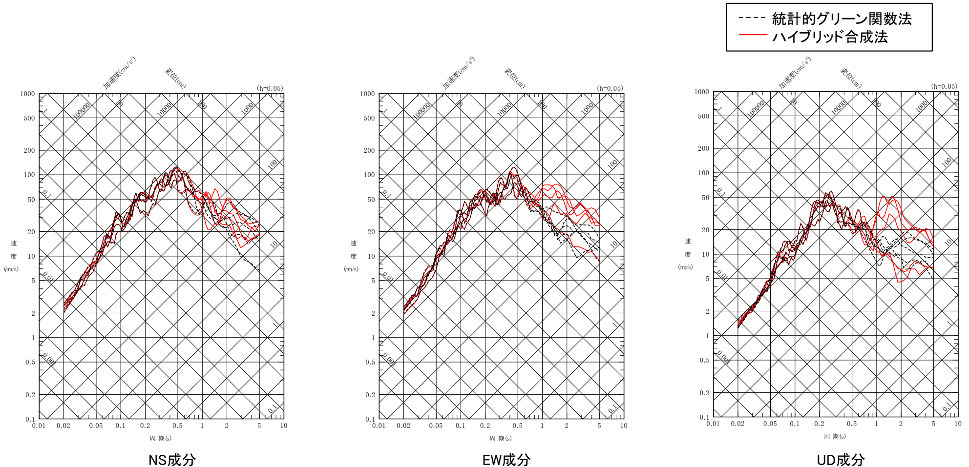
ハイブリッド合成法と統計的グリーン関数法による地震動評価の比較 F-14断層による地震 アスペリティ位置と短周期レベルの不確かさケースの応答スペクトル
