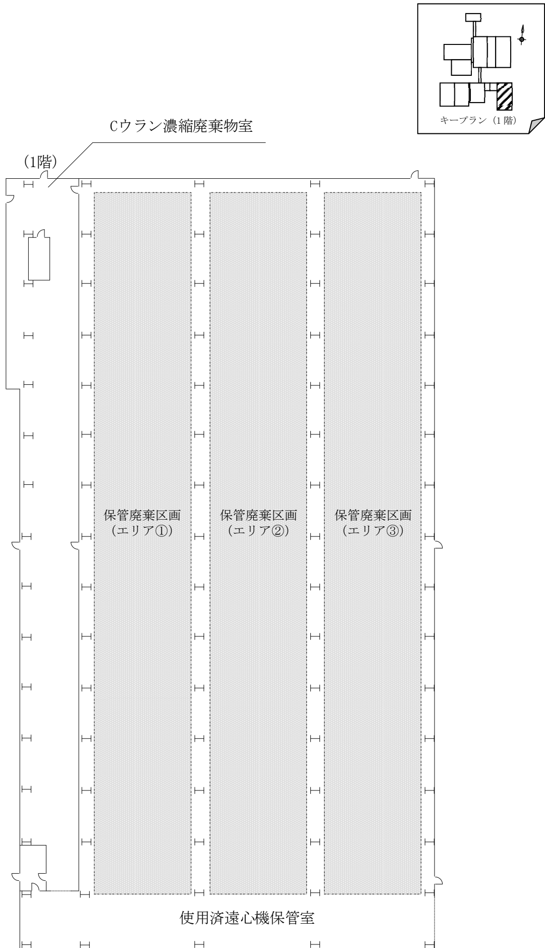
図 2.5.5 固体廃棄物の廃棄設備 機器配置概略図 (固体廃棄物保管廃棄区画)
