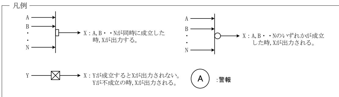
図-1-2-2(2/2) 均質・ブレンディング設備 インターロック (2号均質槽F) (工程用モニタ HF 濃度高による UF 6 漏えい拡大防止のインターロック)
