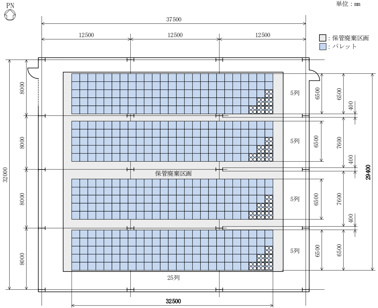
図1 A ウラン濃縮廃棄物室の保管廃棄区画
