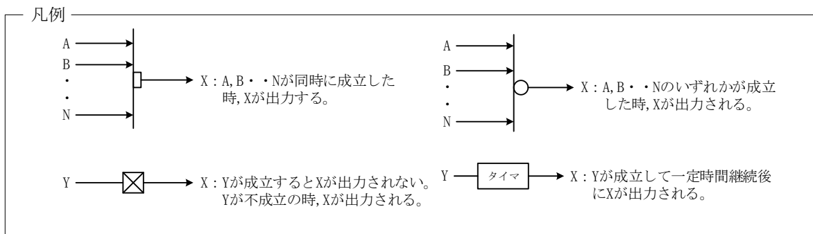
図-1-2-4(1/2) 均質・ブレンド設備 インターロック (2号均質槽) (2号局所排風機2台停止による加熱停止のインターロック)
