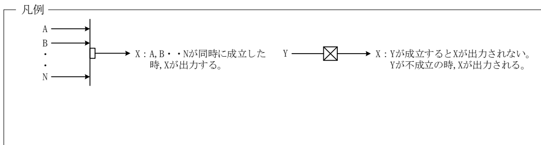
図-1-2-7(2/3) 均質・ブレンド設備 インターロック (2号製品シリンダ槽) (UF 6 シリンダ類交換時の誤操作防止のインターロック)
