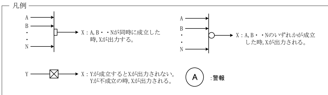
図-1-2-8(2/2) 均質・ブレンディング設備 インターロック (2号均質槽F) (地震発生時のUF 6 漏えい防止インターロック (緊急遮断弁閉, 加熱停止))
