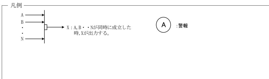
図-1-2-10 (1/2) 均質・ブレンディング設備 インターロック (2号均質槽) (回収側槽類圧力異常上昇によるガス移送停止のインターロック)
