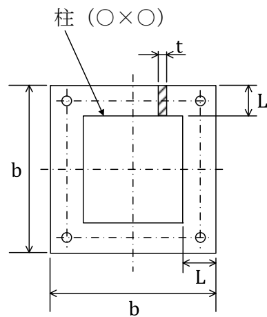
図4 ベースプレートの応力評価の計算モデル
