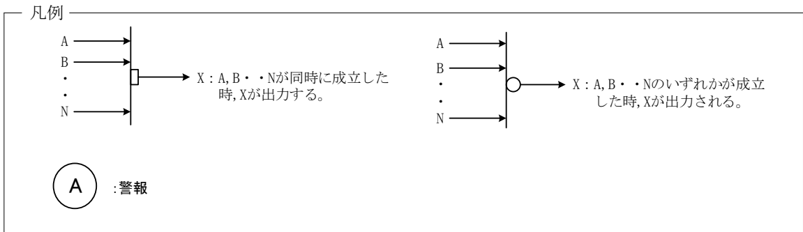
図-1-2-21 均質・ブレンド設備 インターロック (2号サンプル小分け装置) (サンプルシリンダ圧力異常高又は小分け装置温度異常高による加熱停止のインターロック)
