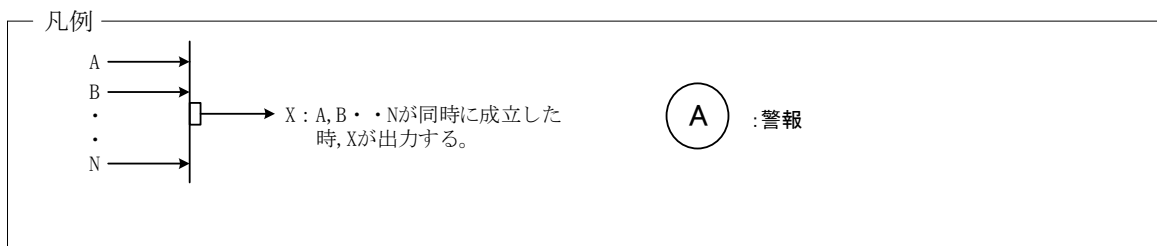
図-1-2-17 均質・ブレンド設備 インターロック (2号原料シリンダ槽) (重量異常高による過充填防止のインターロック)
