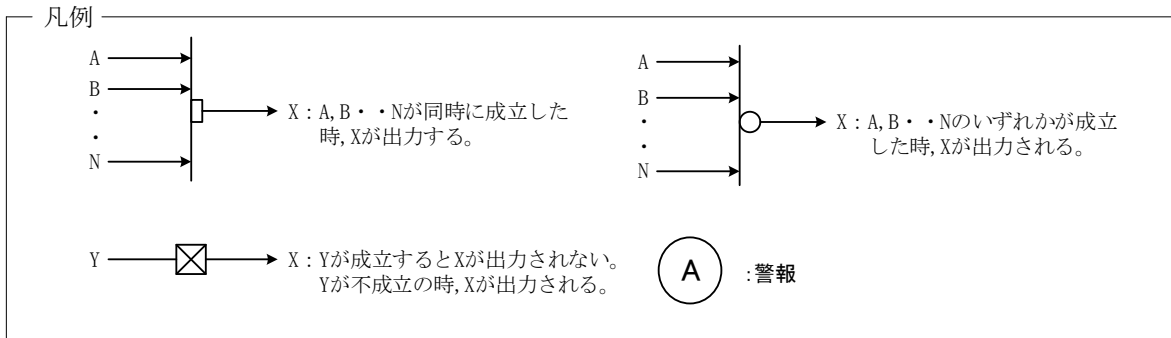
図-1-2-2(1/2) 均質・ブレンディング設備 インターロック (2号均質槽) (工程用モニタ HF 濃度高による UF 6 漏えい拡大防止のインターロック)
