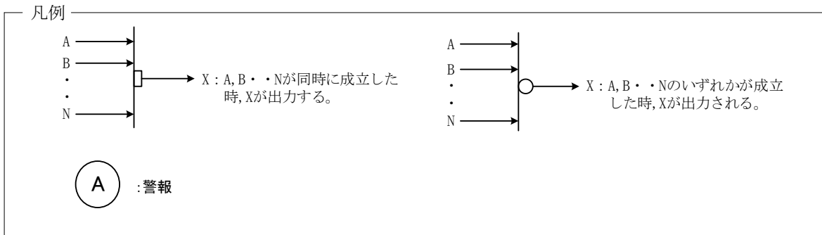
図-1-2-29 液体廃棄物の廃棄設備 インターロック（凝集槽） （受け入れ停止による漏えい防止機能）
