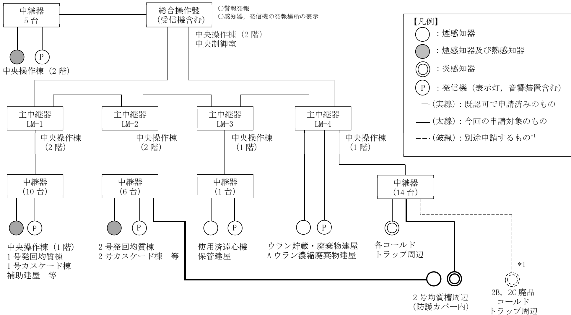
図-1 自動火災報知設備の系統概略図
