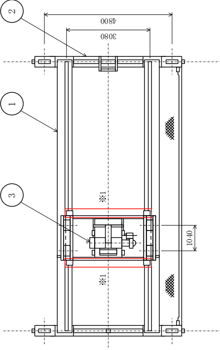
平面図
