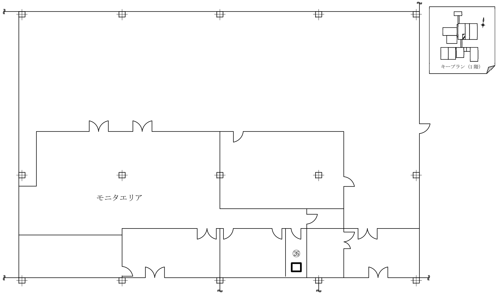
図 2.4.1 液体廃棄物の廃棄設備 機器配置概略図 (4 / 7)
