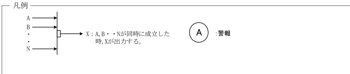
図-1-2-13 均質・ブレンド設備 インターロック (2号製品シリンダ槽) (重量異常高による過充填防止のインターロック)
