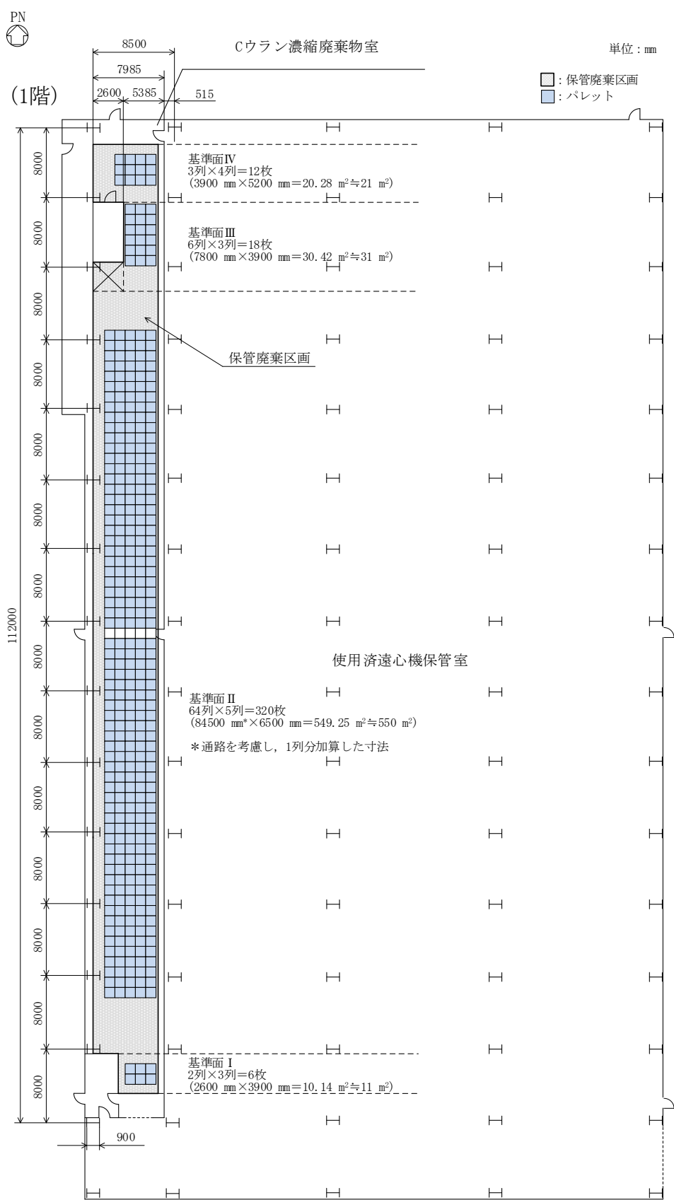
図4 Cウラン濃縮廃棄物室の保管廃棄区画
