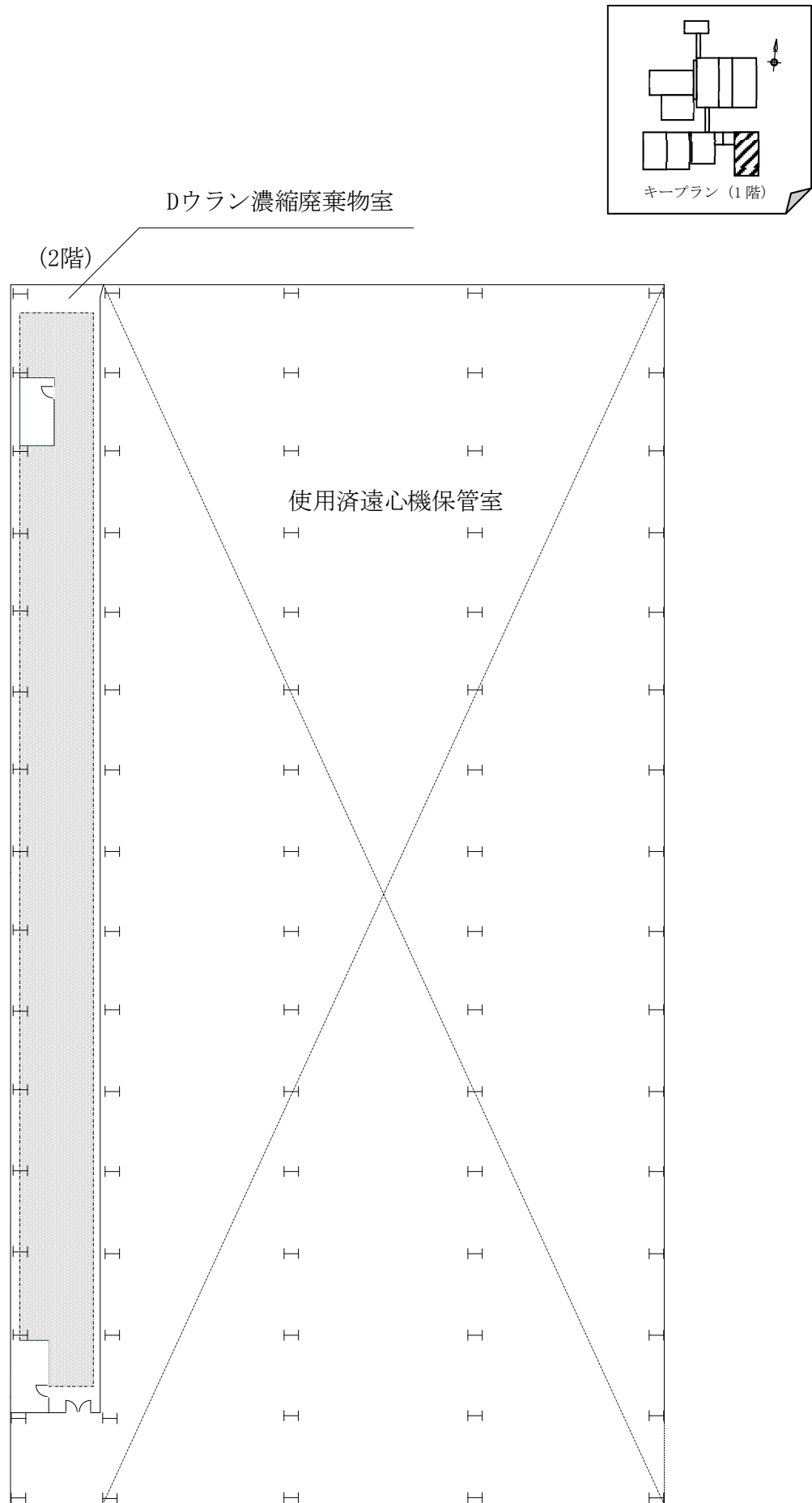
図 2.5.4 固体廃棄物の廃棄設備 機器配置概略図 (固体廃棄物保管廃棄区画)
