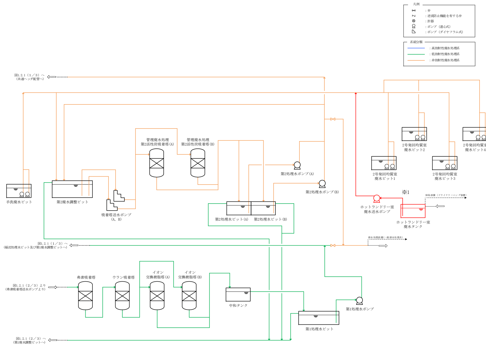
図 1.2.1 液体廃棄物の廃棄設備 系統概略図 (3/3) 変更前
