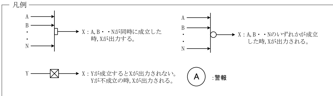
図-1-2-23 均質・ブレンディング設備 インターロック (2号局所排気装置) (工程用モニタ HF 濃度高による UF 6 漏えい拡大防止のインターロック)
