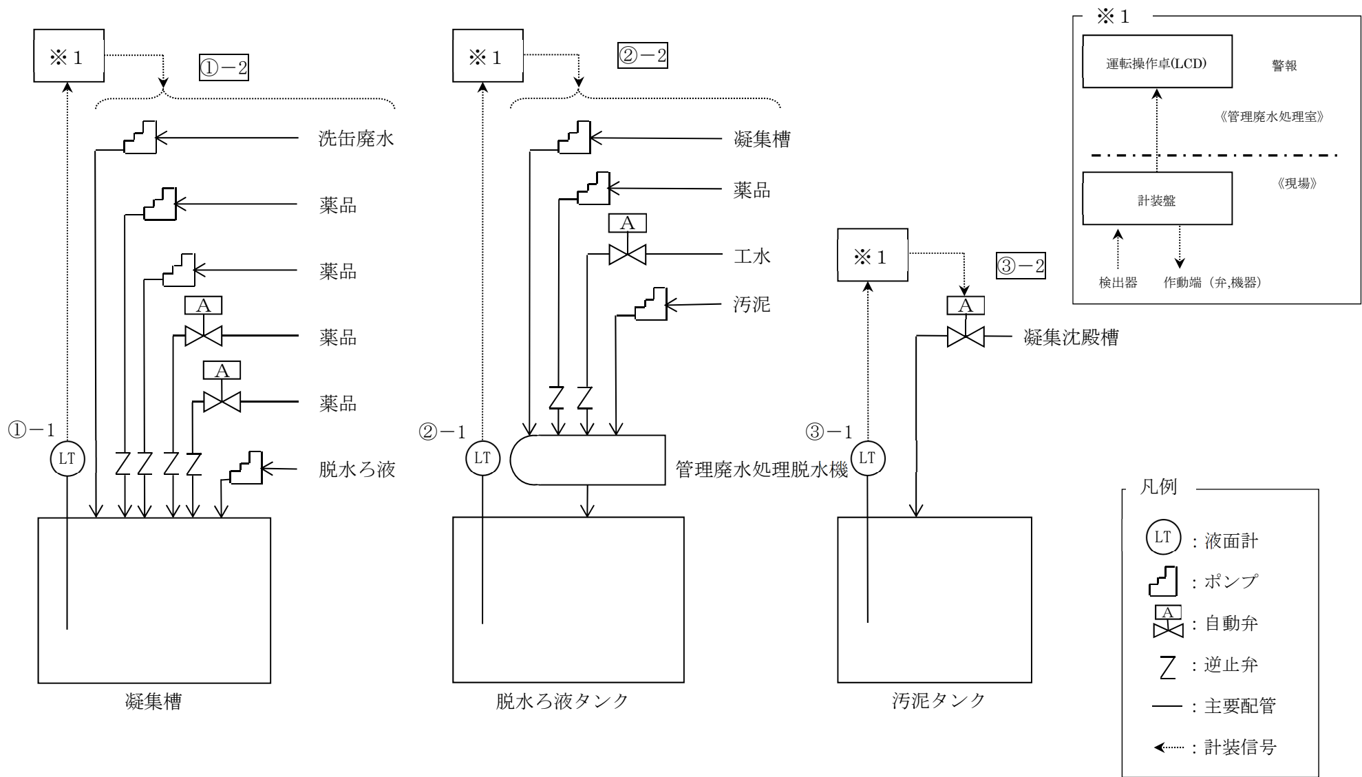
図-1-1-9 液体廃棄物の廃棄設備 インターロック動作概要図
