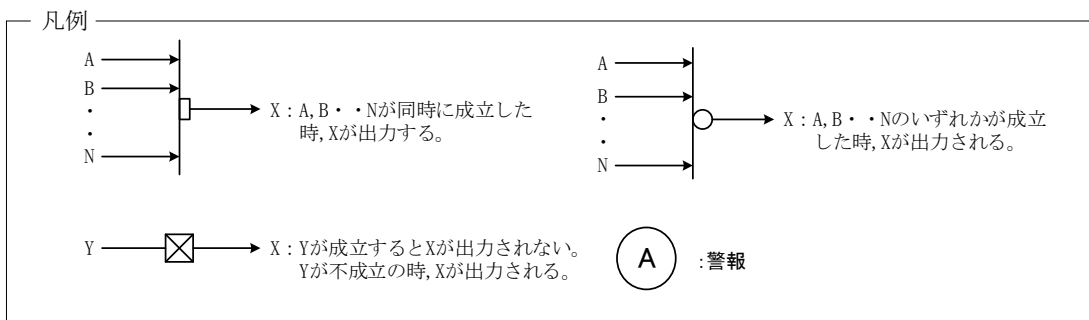
図-1-2-26 均質・ブレンド設備 インターロック (2号均質パージ系コールドトラップ) (地震発生時の加熱停止のインターロック)
