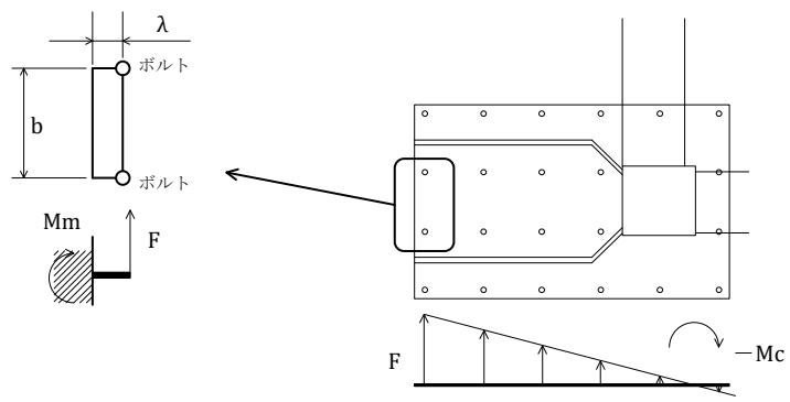
図8 後打ちプレートモデル概略図
