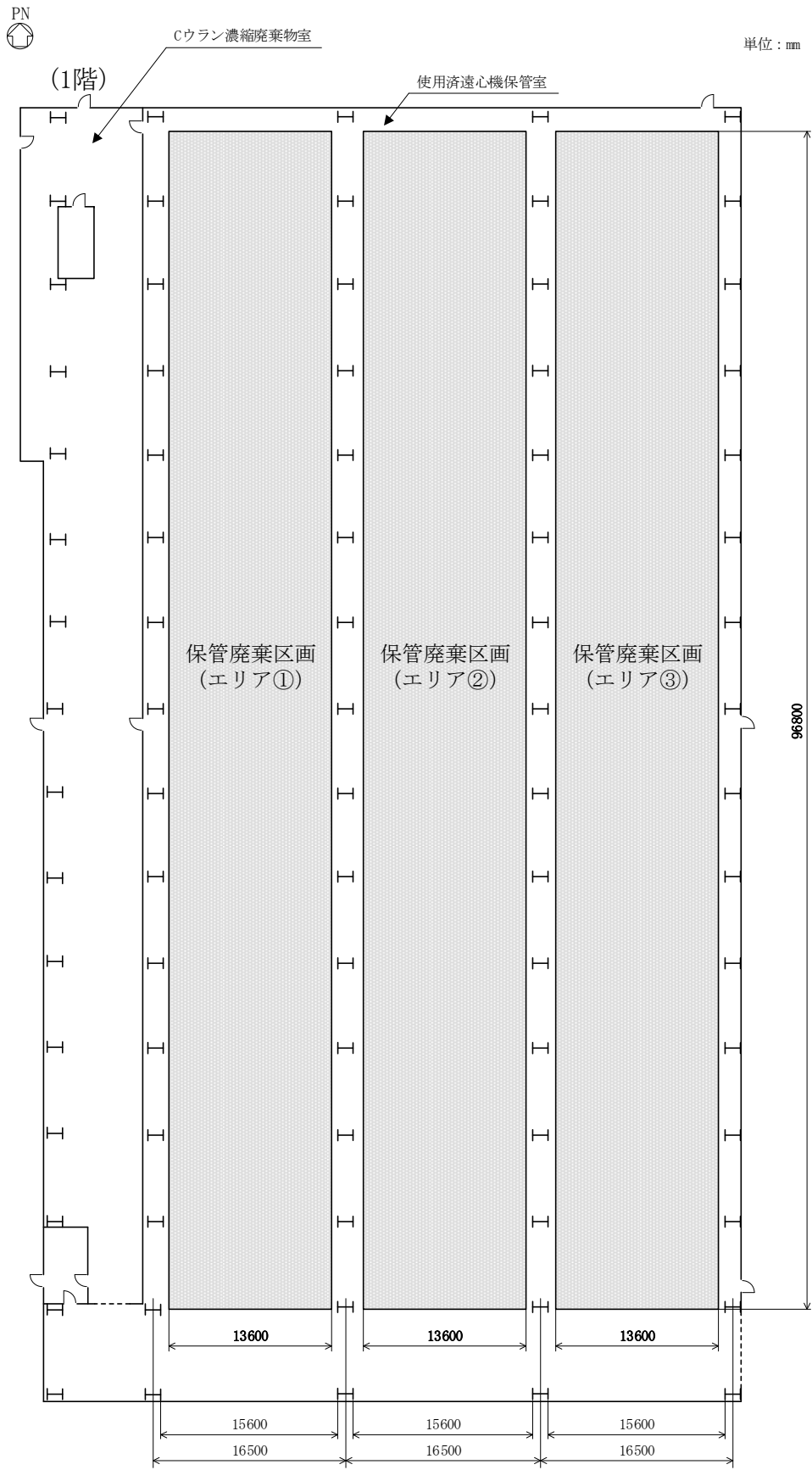
図7 使用済遠心機保管室の保管廃棄区画
