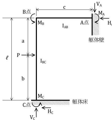
図 7 支持架構モデル概略図
