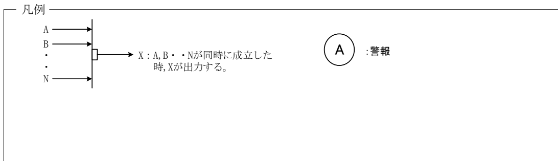
図-1-2-10 (2/2) 均質・ブレンディング設備 インターロック (2号均質槽) (回収側槽類圧力異常上昇によるガス移送停止のインターロック)
