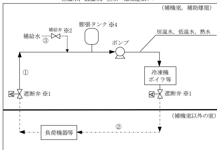
恒温水、低温水、熱水 循環運転フロー
