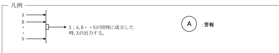
図-1-2-1(2/2) UF 6 処理設備 インターロック (2号一般パージ系コールドトラップ) (回収側槽類圧力異常上昇によるガス移送停止のインターロック)
