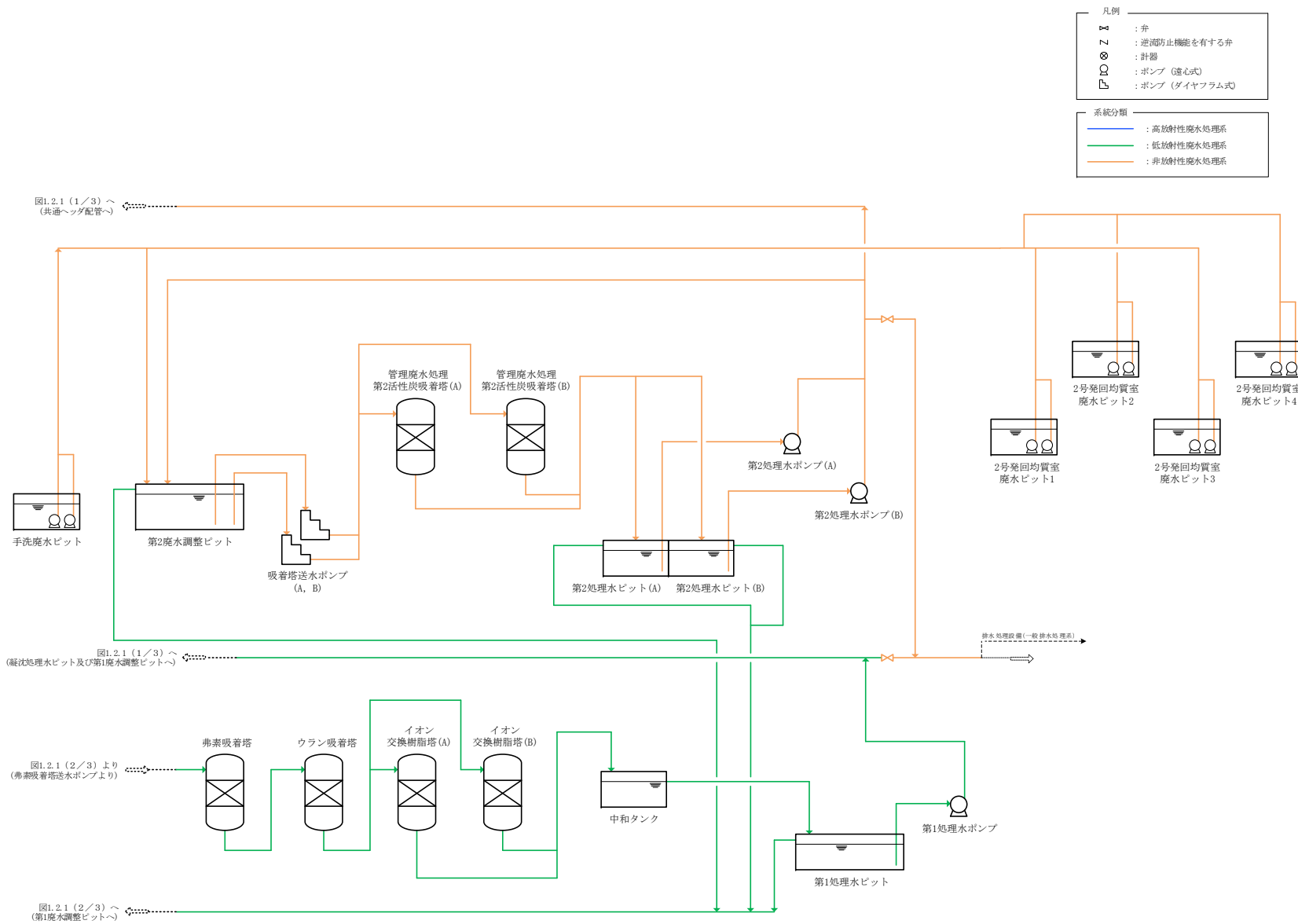
図 1.2.1 液体廃棄物の廃棄設備 系統概略図 (3/3) 変更後
