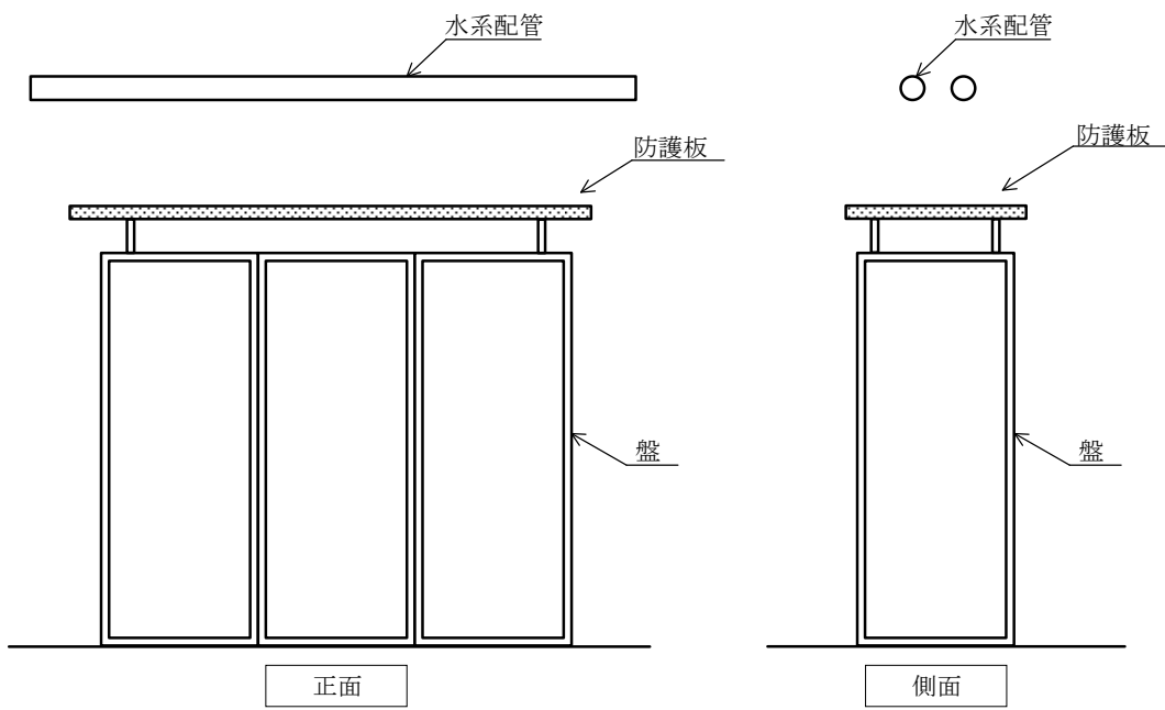
図-5 防護板の設置概要図
