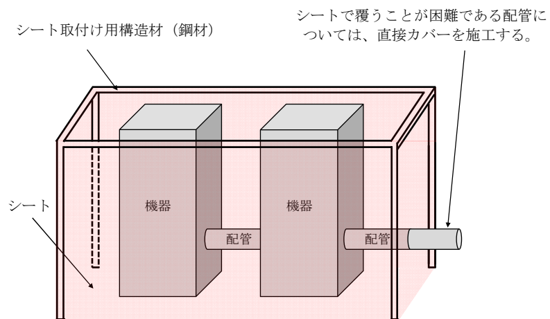
図3 (2/4) UF 6 の直接暴露の防止に関する概要図 (機器を覆うように施工する場合)
