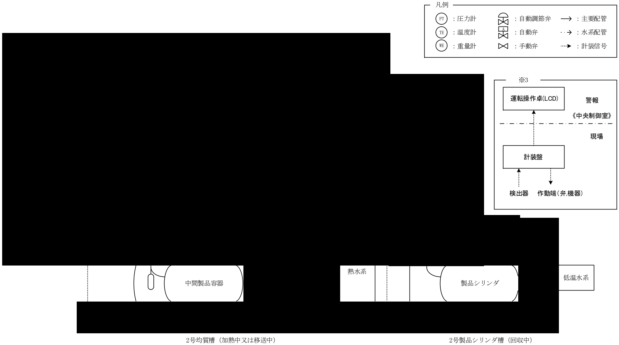
図-1-1-3 均質・ブレンド設備 インターロック動作概要図 (2号均質槽他) (製品・廃品 UF 6 の充填)
