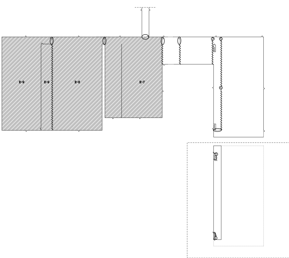
図 2.7.2 非常用設備 機器配置概略図（火災区域構造物（ウラン貯蔵・廃棄物建屋））（2 / 2）
