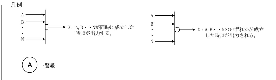
図-1-2-11 均質・ブレンド設備 インターロック (2号製品シリンダ槽 F) (圧力異常高又は温度異常高による加熱停止のインターロック)
