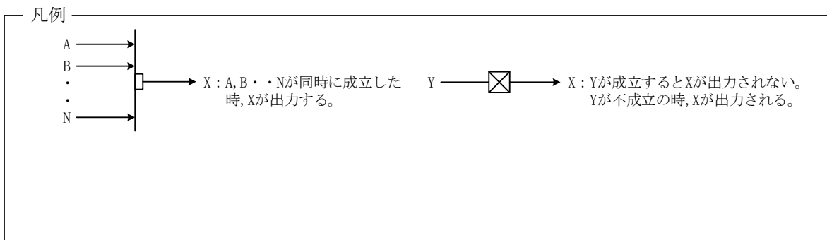
図-1-2-7(1/3) 均質・ブレンド設備 インターロック (2号均質槽) (UF 6 シリンダ類交換時の誤操作防止のインターロック)
