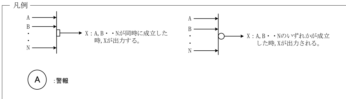
図-1-2-5(1/2) 均質・ブレンド設備 インターロック (2号均質槽) (均質槽槽内圧力異常高による運転停止のインターロック)
