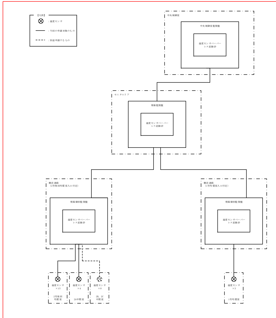
図 1.5.2 非常用設備（温度センサ） 系統概略図
