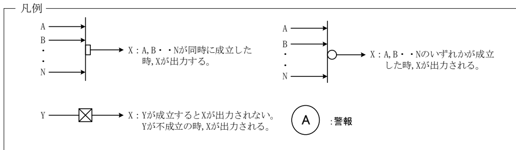
図-1-2-24 均質・ブレンディング設備 インターロック (2号局所排気装置) (地震発生時のUF 6 漏えい防止インターロック (ダンパ閉によるUF 6 閉じ込め))
