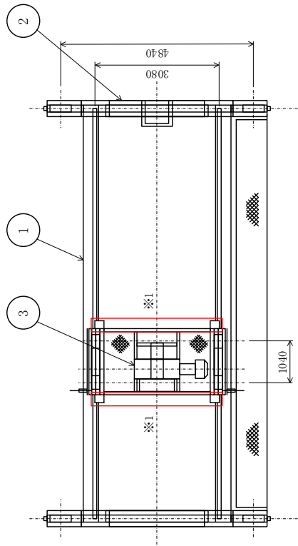
平面図
