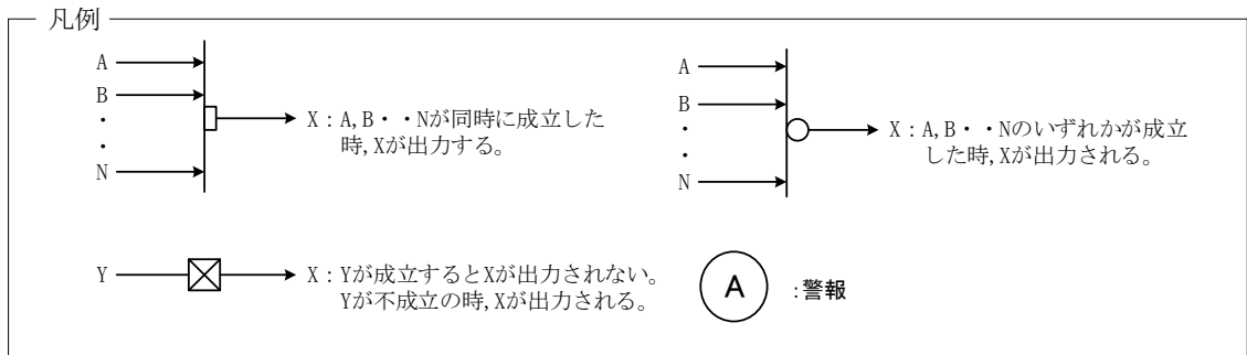
図-1-2-22 均質・ブレンド設備 インターロック (2号サンプル小分け装置) (地震発生時の加熱停止のインターロック)
