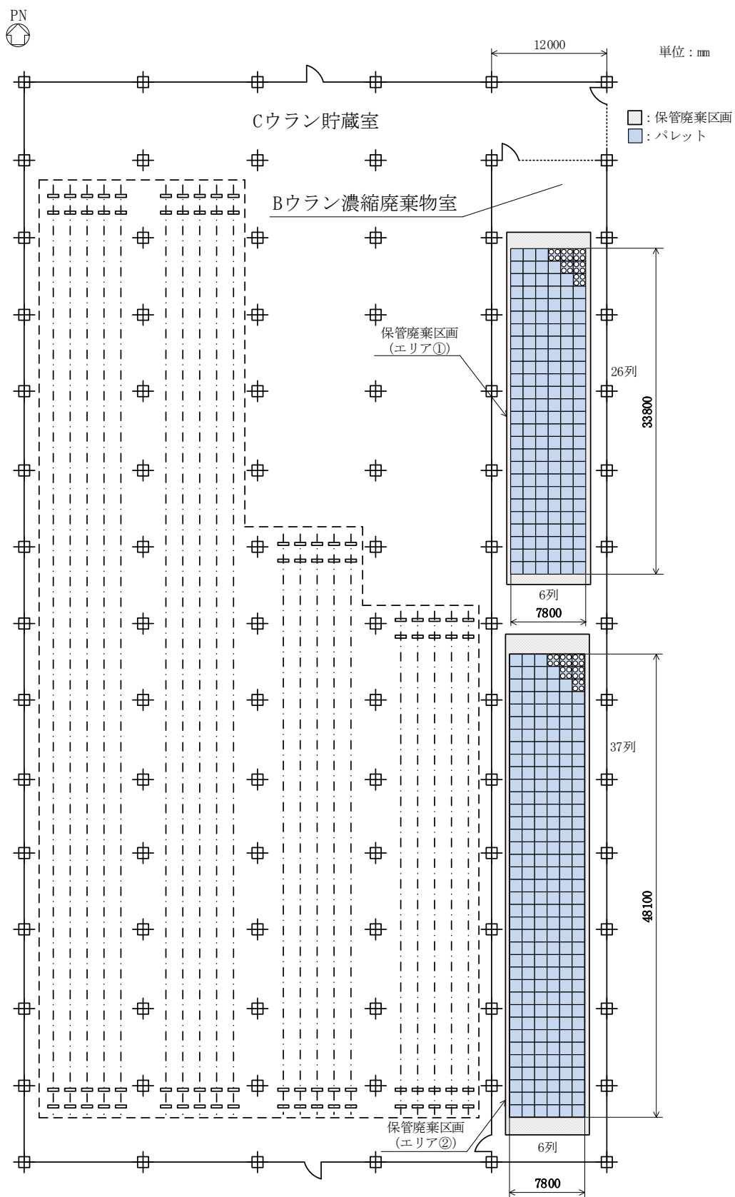
図3 Bウラン濃縮廃棄物室の保管廃棄区画
