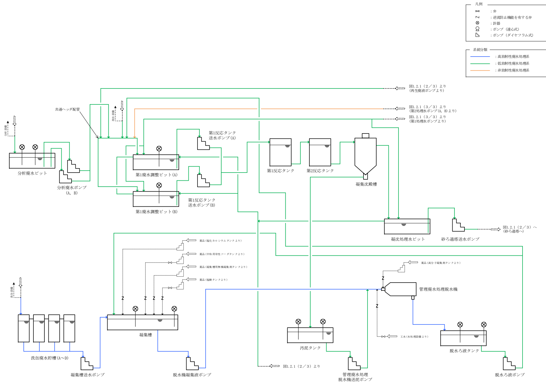
図 1.2.1 液体廃棄物の廃棄設備 系統概略図 (1 / 3)
