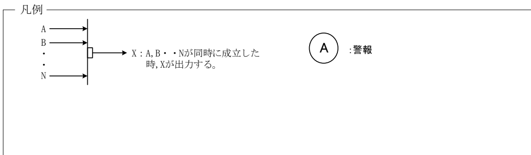
図-1-2-14(2/2) 均質・ブレンド設備 インターロック (2号製品シリンダ槽 F) (回収側槽類圧力異常上昇によるガス移送停止のインターロック)
