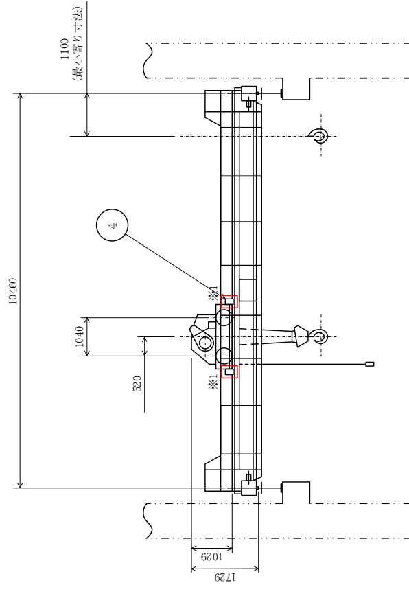
正面図
