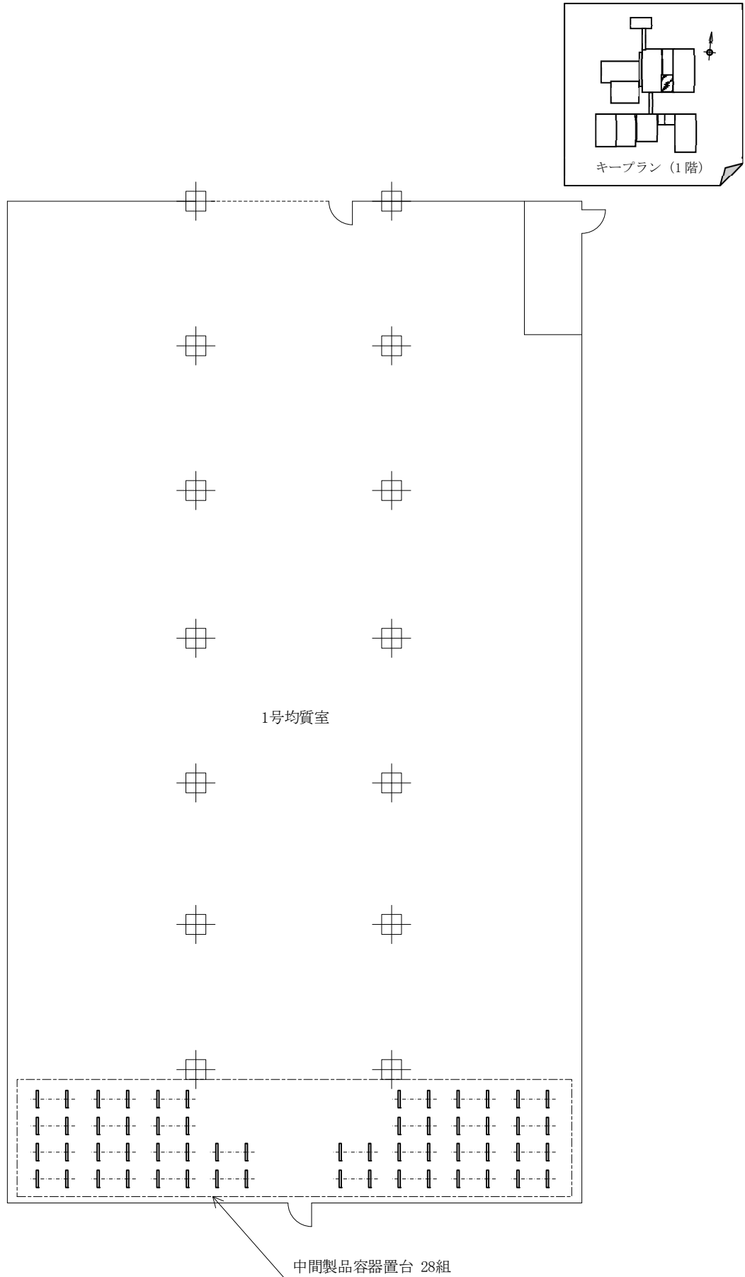
図 2.2.1 貯蔵設備 機器配置概略図 (4 / 5)
