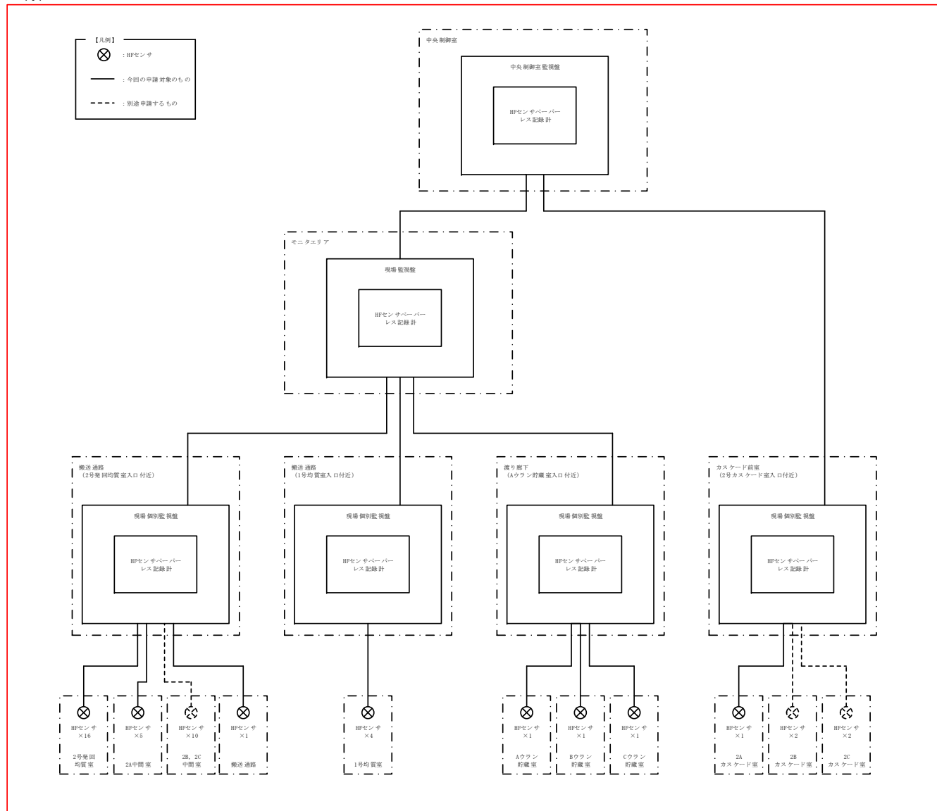
図 1. 4. 1 放射線監視・測定設備 (HF センサ) 系統概略図
