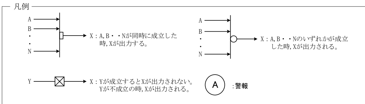
図-1-2-3(1/2) 均質・ブレンド設備 インターロック (2号均質槽) (減圧槽故障による均質槽加熱停止インターロック)
