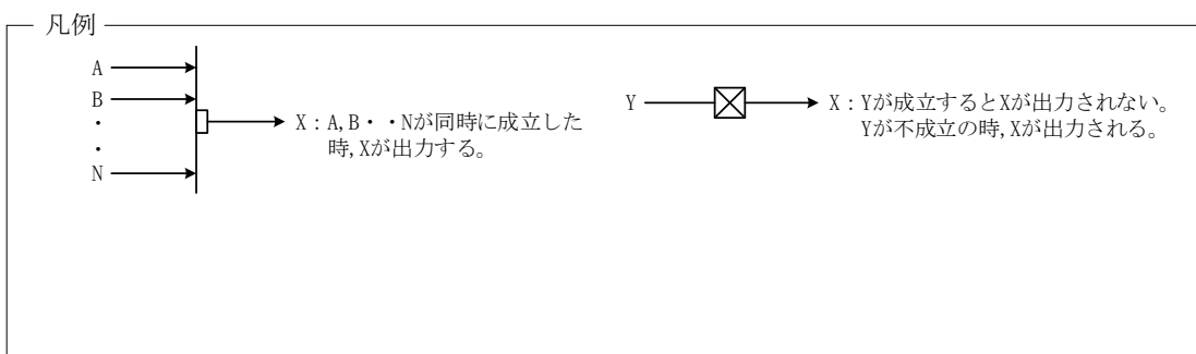
図-1-2-20 均質・ブレンド設備 インターロック (2号サンプル小分け装置) (2号局所排風機2台停止による加熱停止のインターロック)
