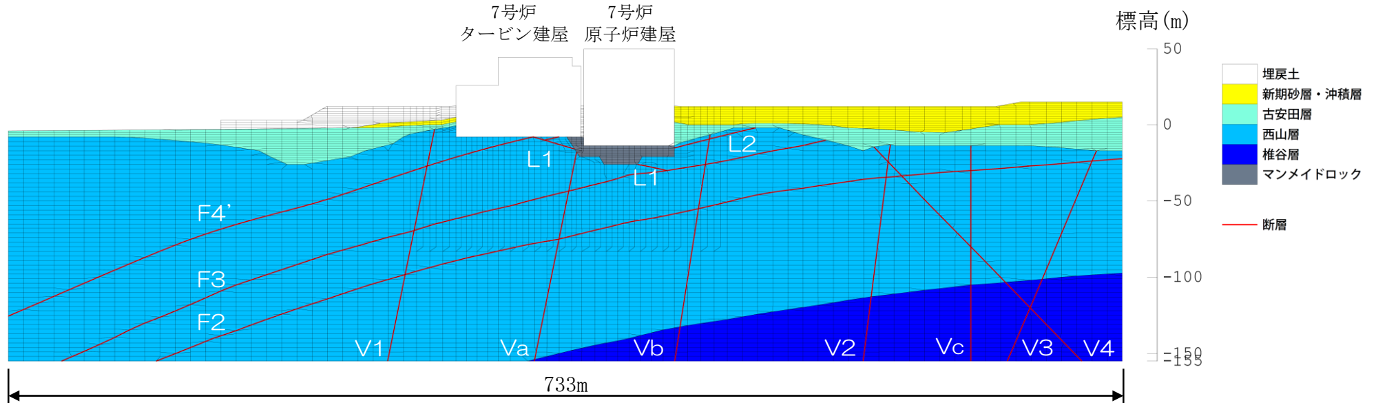
7号炉原子炉建屋 汀線直交断面 C-C'
