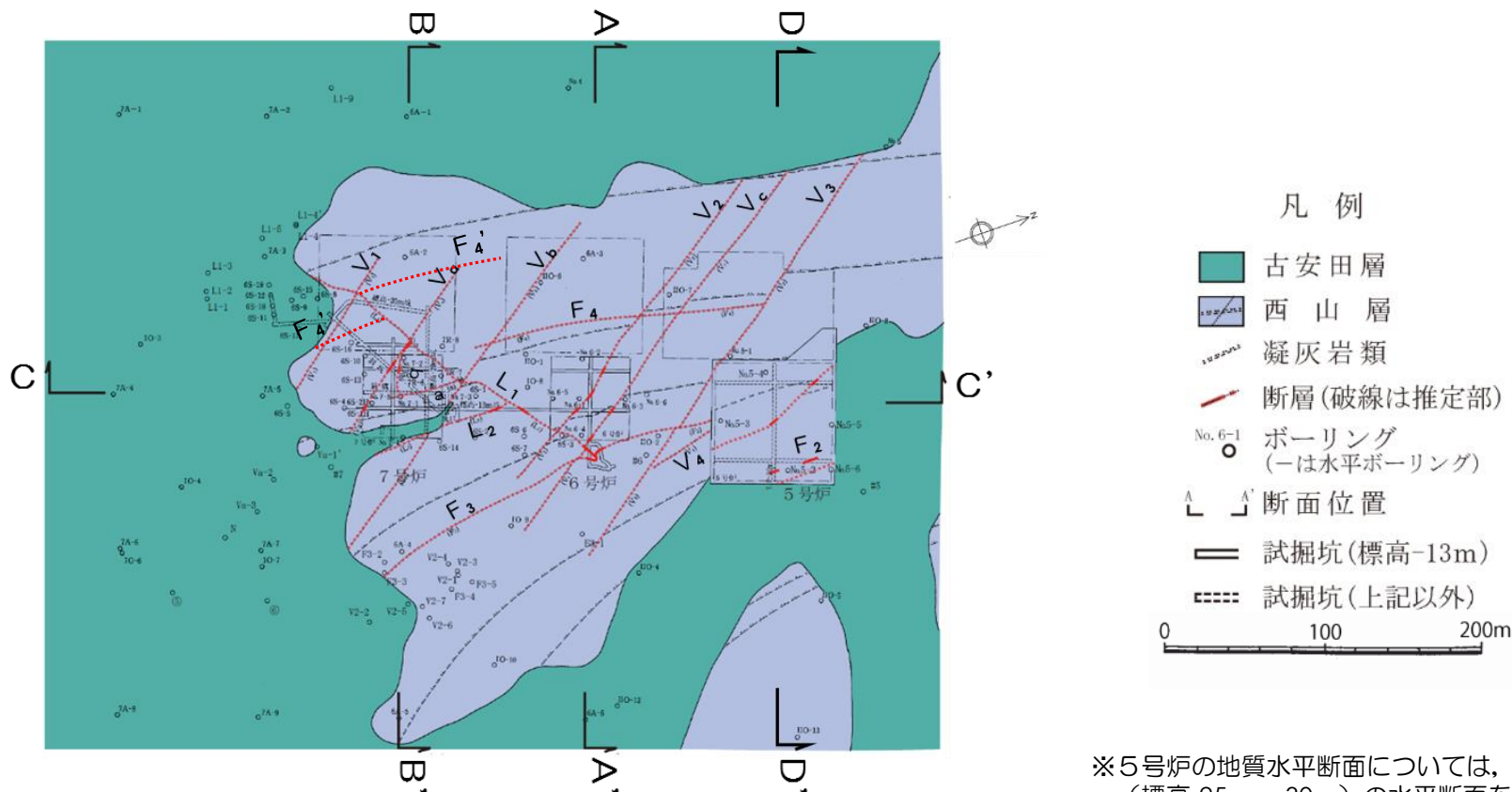
5号、6号及び7号炉付近(標高約-13m ** )の地質水平断面図
