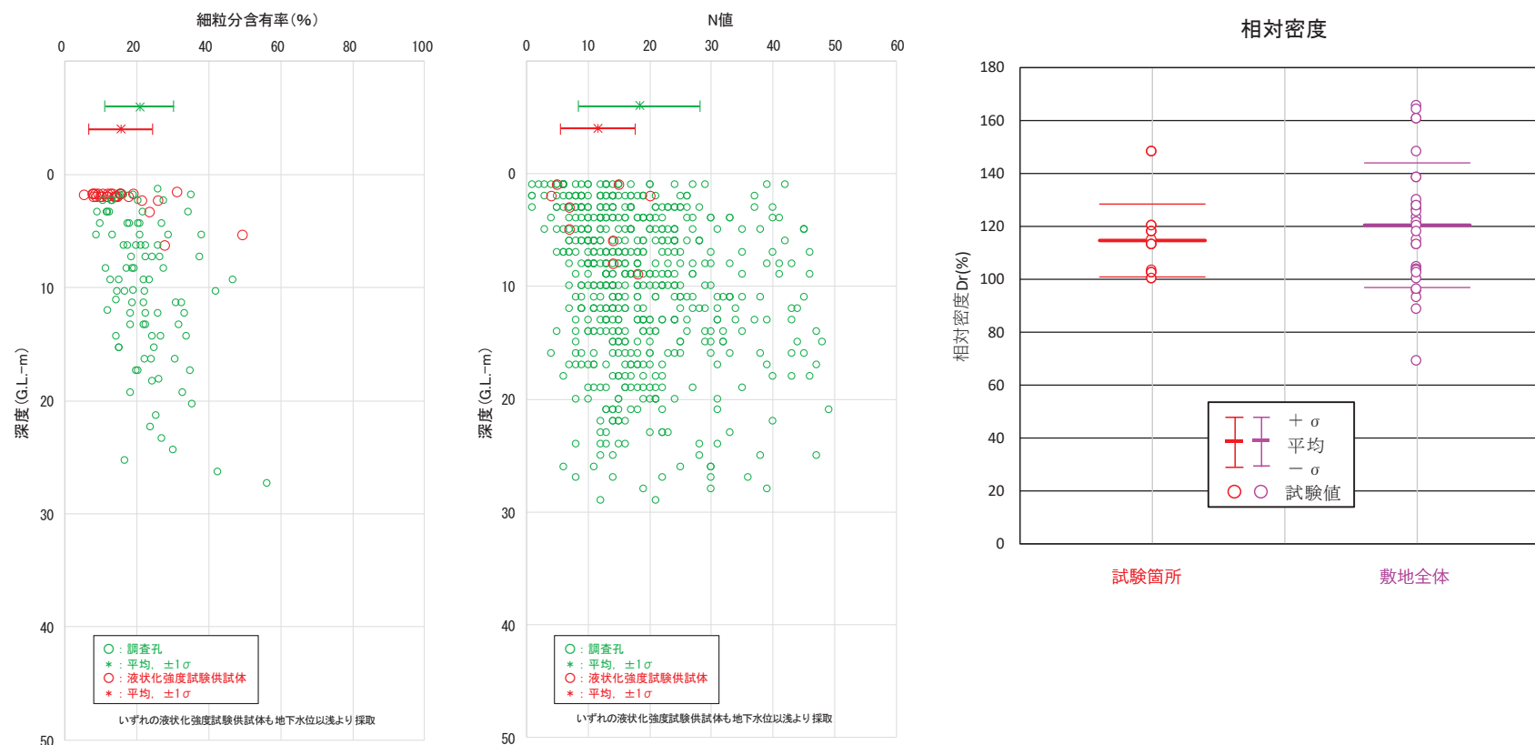
細粒分含有率, N値及び相対密度の確認結果
