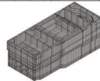
海水ポンプ室の解析モデル
