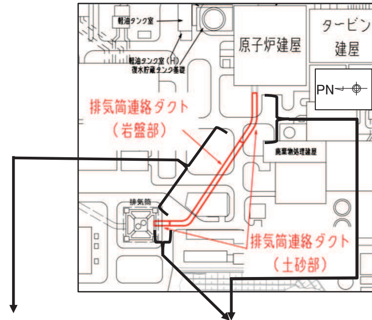
排気筒連絡ダクト配置平面図
