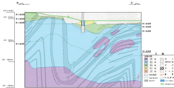
(No.1揚水井戸, A-A)
