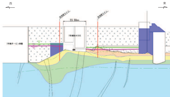
防潮壁(第3号機放水立坑) 断面⑥-⑥' (EW方向)
