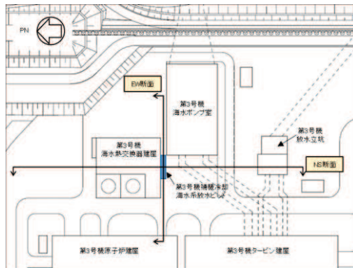
(第3号機補機冷却海水系放水ピット)
