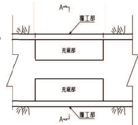
縦断面図(B-B断面)
