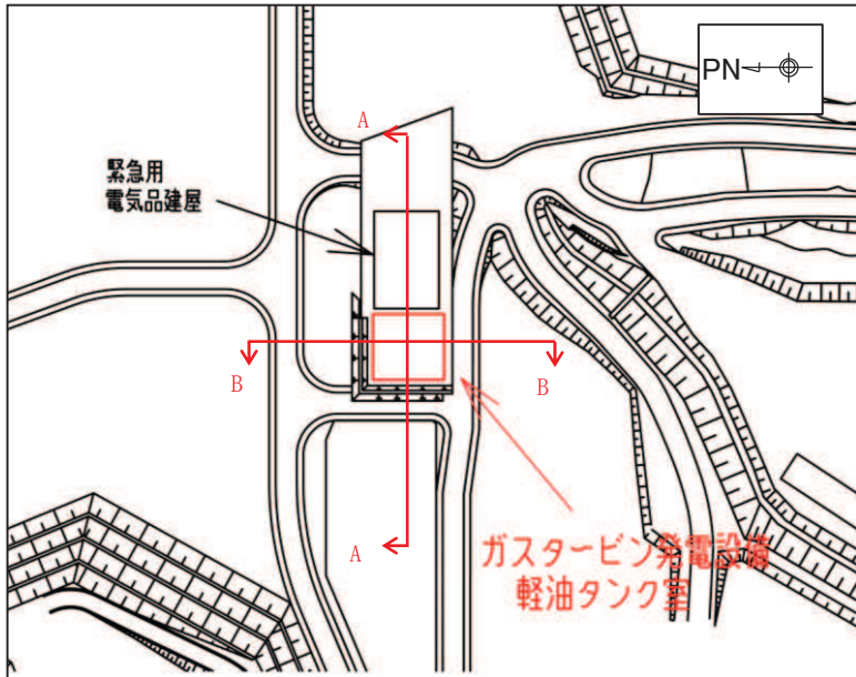
掘削図
