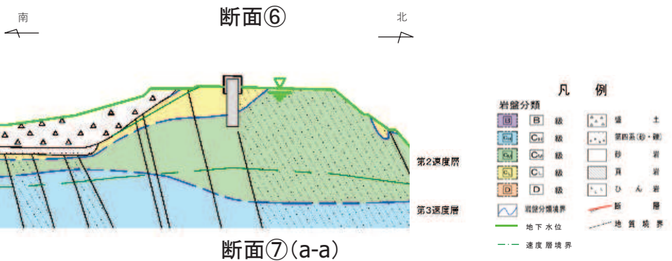
評価対象地質断面図
