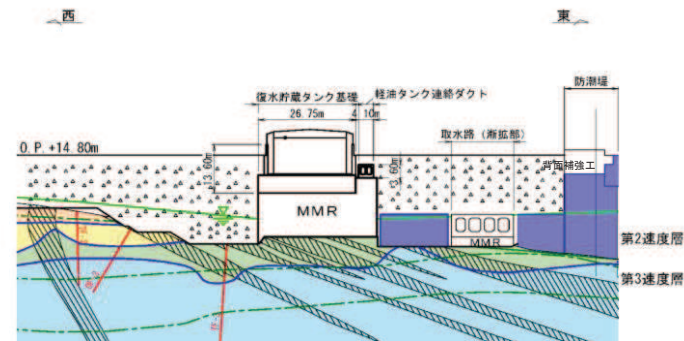
評価対象地質断面図(B-B)
