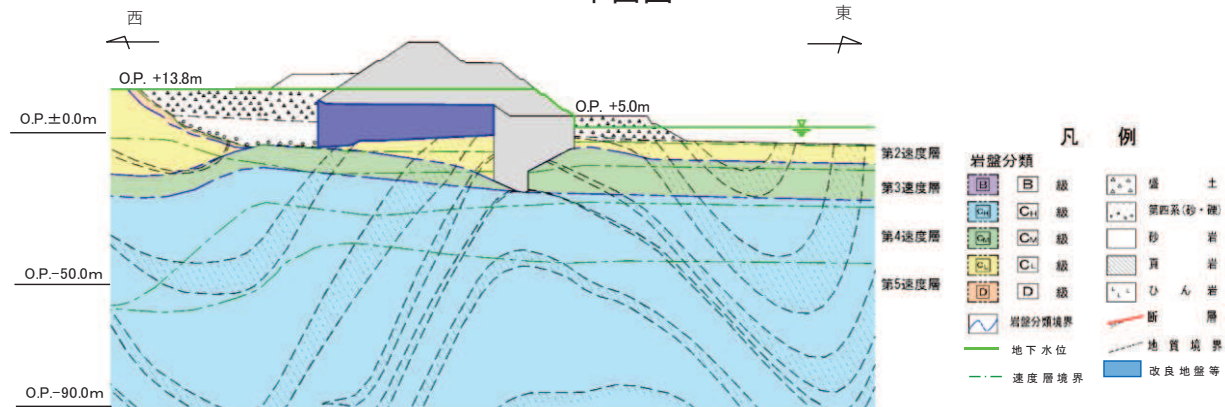
評価対象断面図(断面①)
