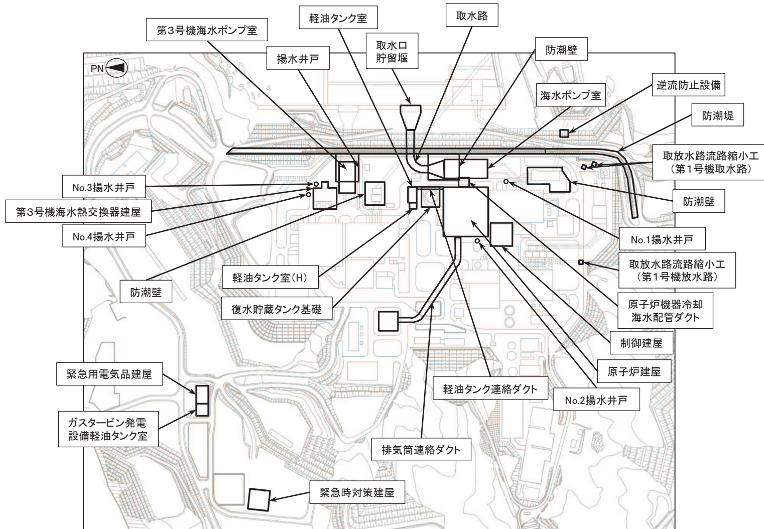
評価対象施設の全体配置図
