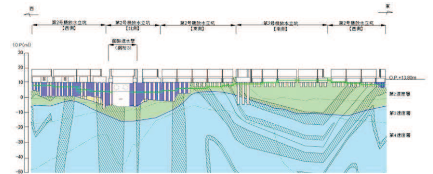
防潮壁(第2号機放水立坑)
