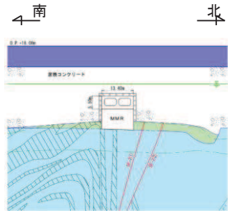
断面④
