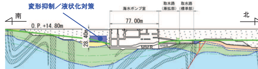
海水ポンプ室(縦断面)
