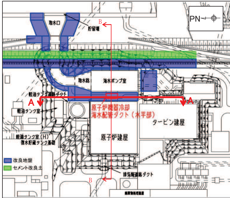
掘削図
