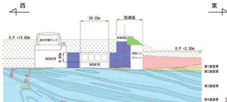
取水路(漸拡部)地質断面図(A-A)
