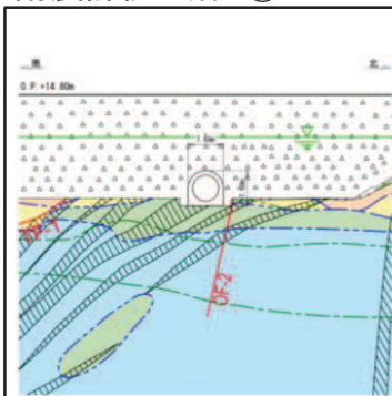
断面①
