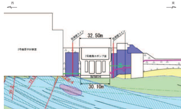
防潮壁(第2号機海水ポンプ室) 断面①-①'(EW方向)
