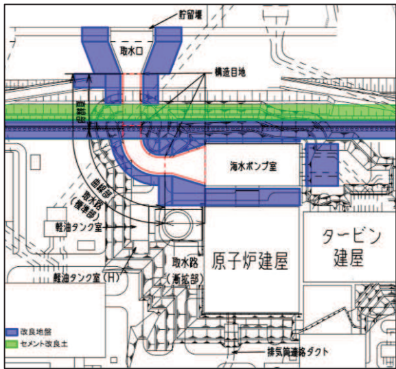
掘削図
