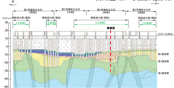
防潮壁(第3号機放水立坑)
