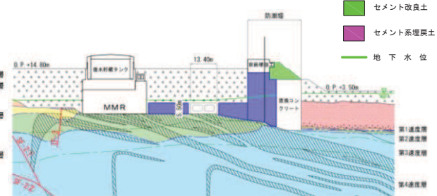
断面⑦
