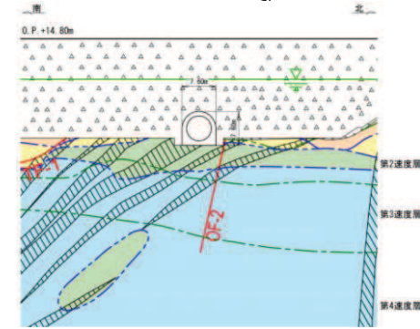
排気筒連絡ダクト(土砂部)
