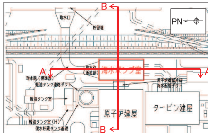
海水ポンプ室の掘削図と地盤改良範囲
