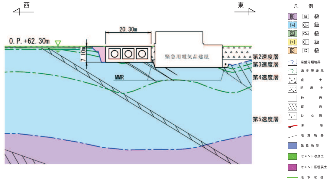
地震時荷重用地質断面図(A-A)
