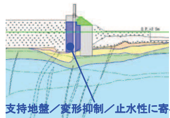
断面①
