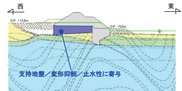
盛土堤防(断面①)
