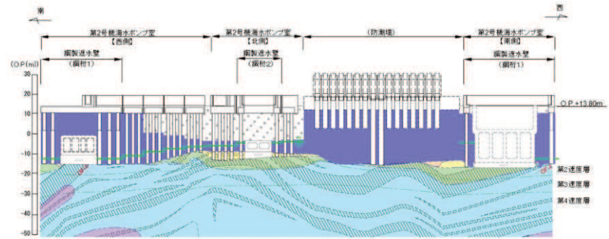
防潮壁(第2号機海水ポンプ室)
