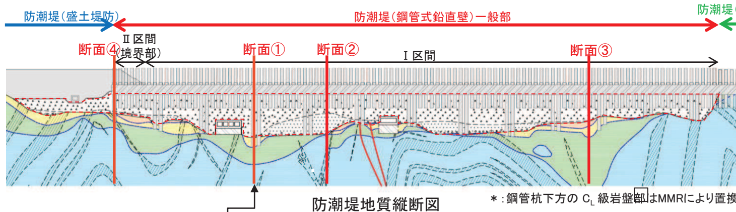
耐震・耐津波評価: 断面①の例
