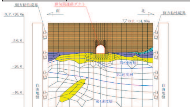
排気筒連絡ダクト(土砂部)の解析モデル
