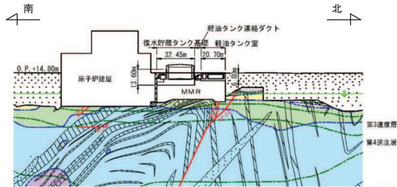
評価対象地質断面図(A-A)
