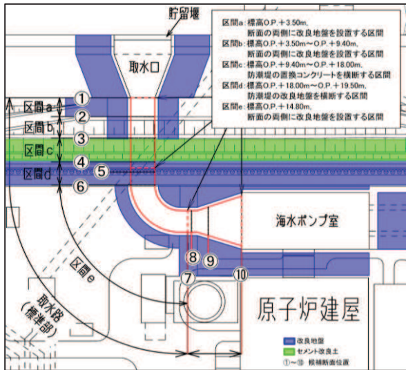
平面図
