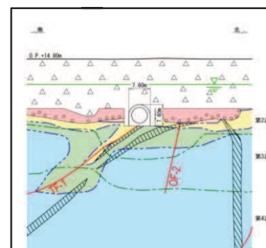
断面②
