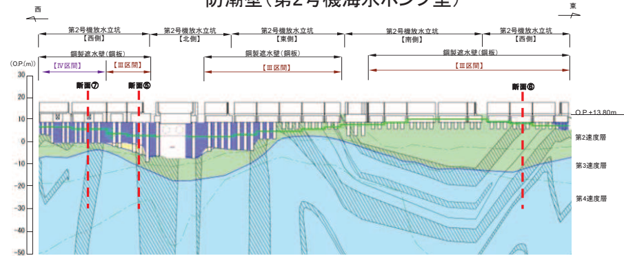
防潮壁(第2号機放水立坑)
