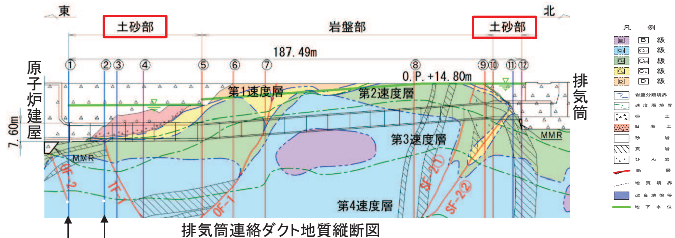
断層影響評価: 断面②
