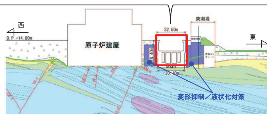
横断面(B-B断面)
