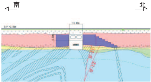
断面②
