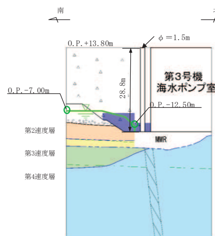
(揚水井戸(第3号機海水ポンプ室防潮壁区画内))
