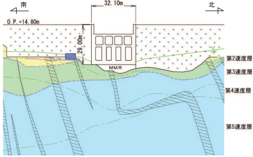
スクリーンエリア(A-A)
