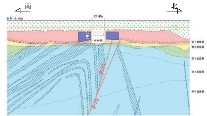
断面③
