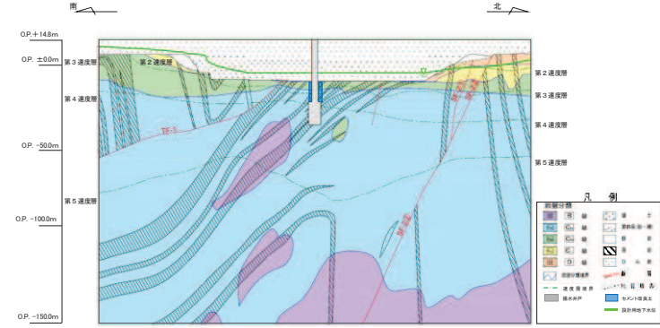
(No.2揚水井戸, B-B)
