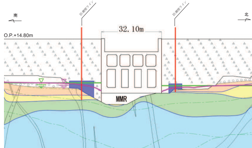
防潮壁(第3号機海水ポンプ室) 断面⑤-⑤' (NS方向)
