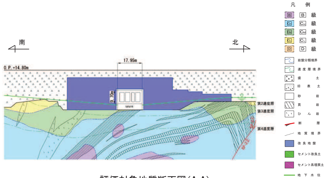
評価対象地質断面図(A-A)
