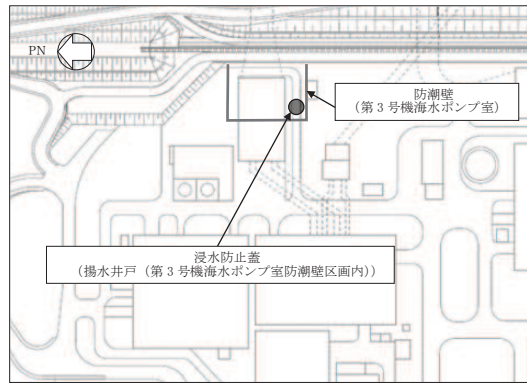
(揚水井戸(第3号機海水ポンプ室防潮壁区画内))
