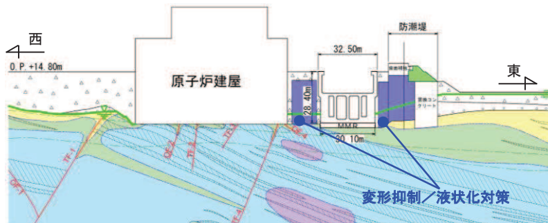
海水ポンプ室(横断面)
