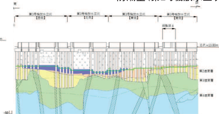
防潮壁(第3号機放水立坑)
