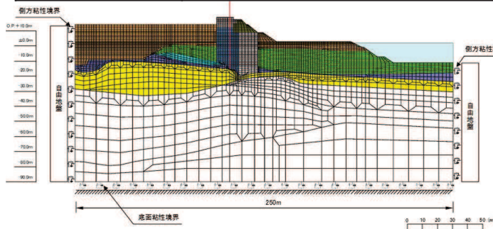
鋼管式鉛直壁(一般部, 断面②)の解析モデル
