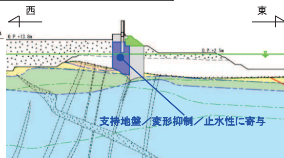
鋼管式鉛直壁(一般部, 断面②)
