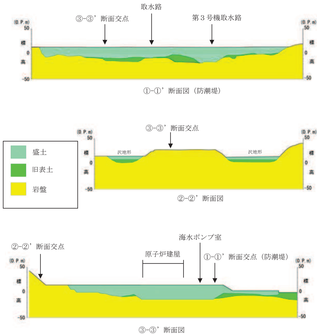
盛土及び旧表土の分布断面図
