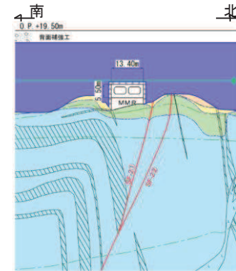
断面⑤
