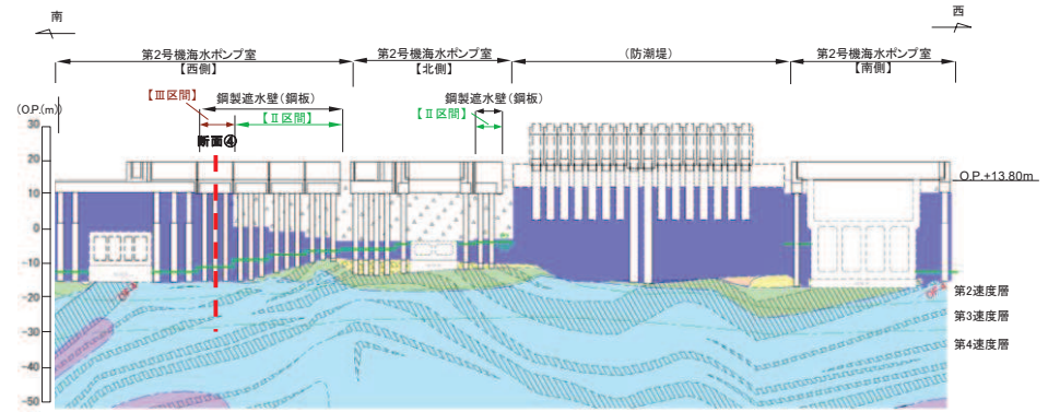
防潮壁(第2号機海水ポンプ室)
