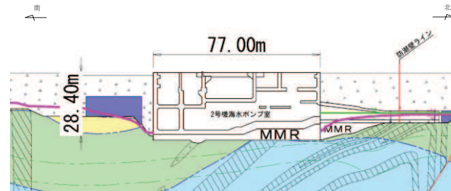
防潮壁(第2号機海水ポンプ室) 断面②-②'(NS方向)
