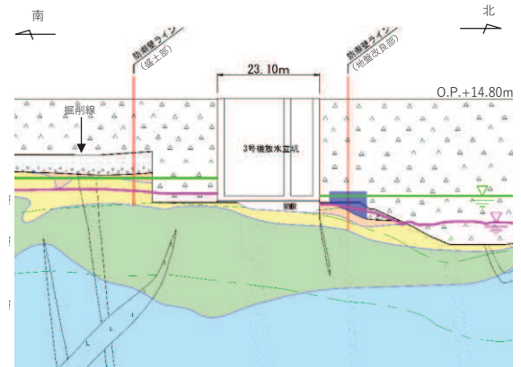
防潮壁(第3号機放水立坑) 断面⑦-⑦' (NS方向)
