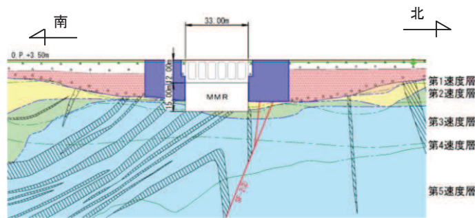
取水口(標準部)地質断面図(B-B)
