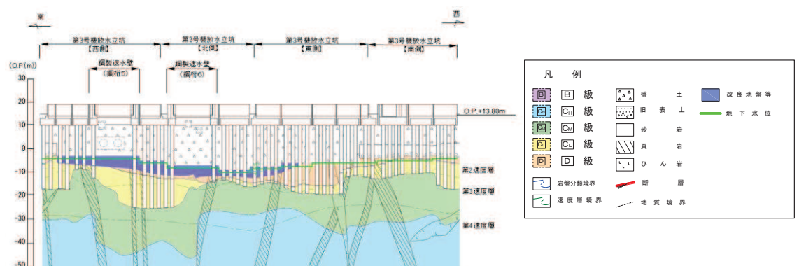
防潮壁(第3号機放水立坑)
