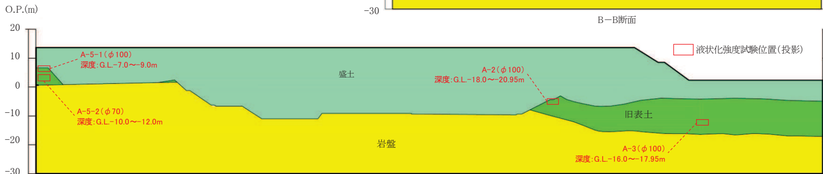
C-C断面
