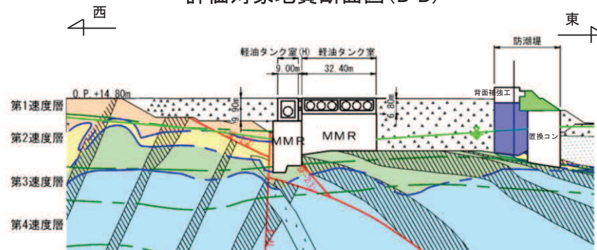
評価対象地質断面図(C-C)
