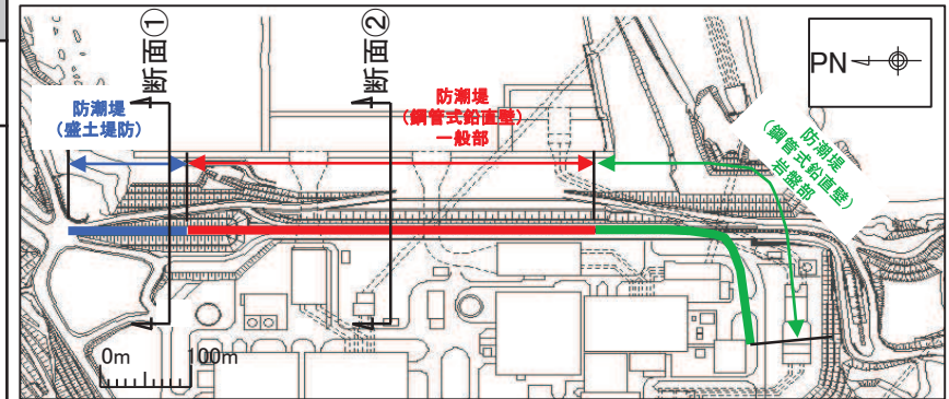
防潮堤配置平面図
