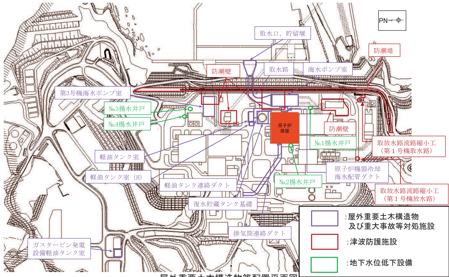
屋外重要土木構造物等配置平面図
