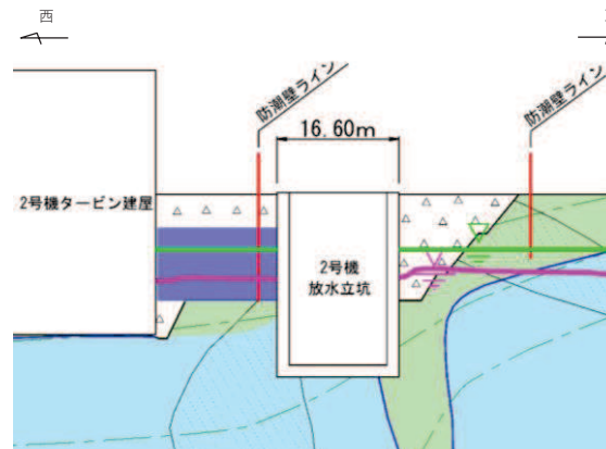
防潮壁(第2号機放水立坑) 断面③-③'(EW方向)
