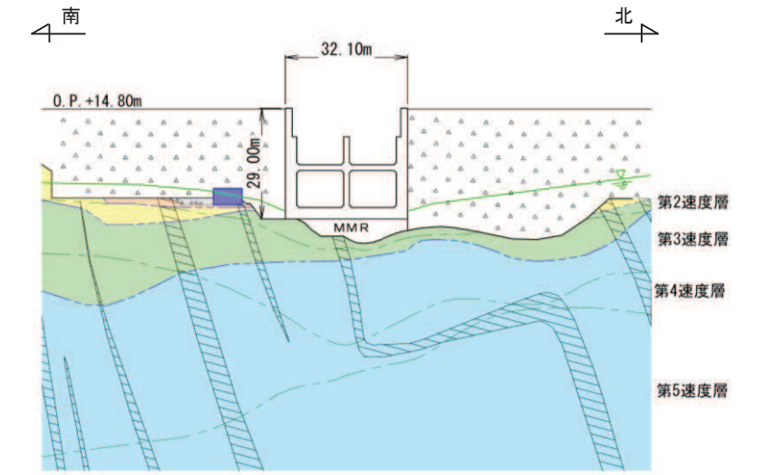
循環水ポンプエリア(B-B)
