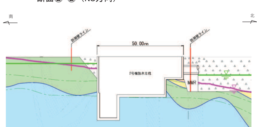
防潮壁(第2号機放水立坑) 断面④-④'(NS方向)
