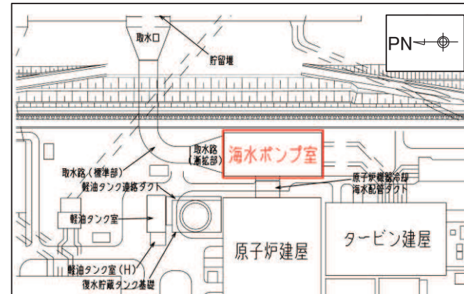
海水ポンプ室配置平面図
