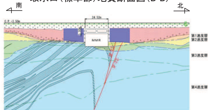
取水口(漸縮部)地質断面図(C-C)
