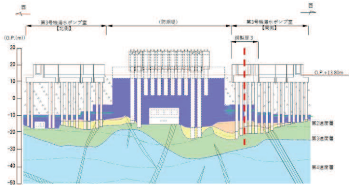
防潮壁(第3号機海水ポンプ室)
