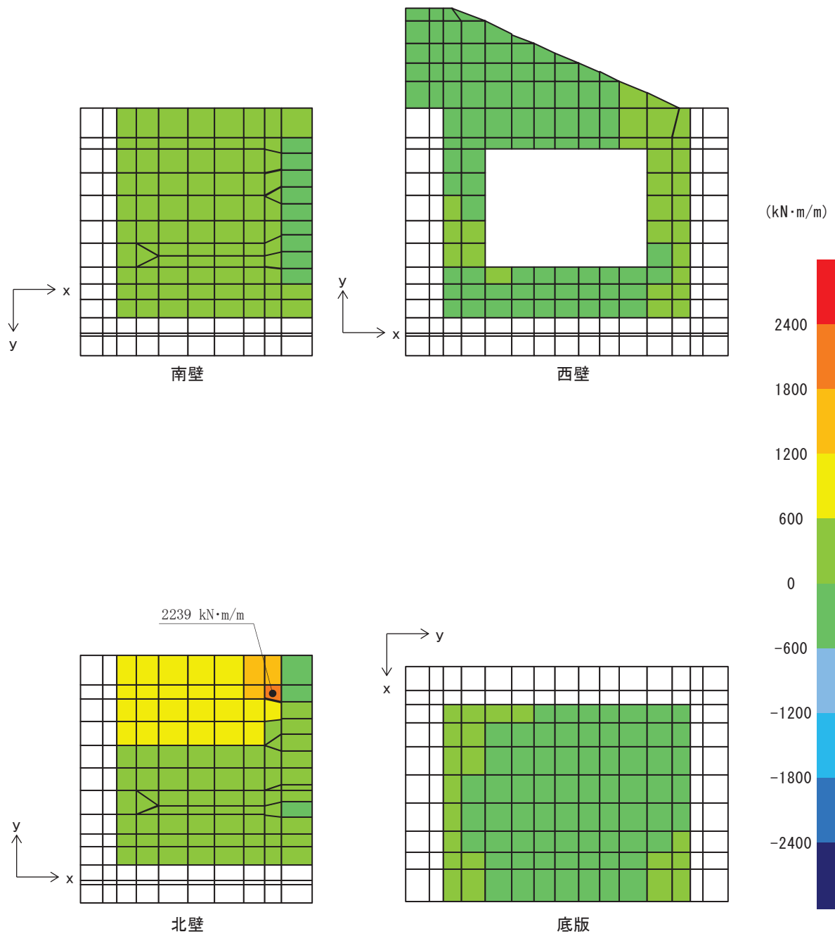
図 8-10 曲げ・軸力系の破壊に対する照査値最大時の断面力分布図 (曲げモーメント( \text{kN}\cdot\text{m}/\text{m} ) : M_x ) (北壁, 解析ケース③, 衝突荷重作用位置 : 北端部)
