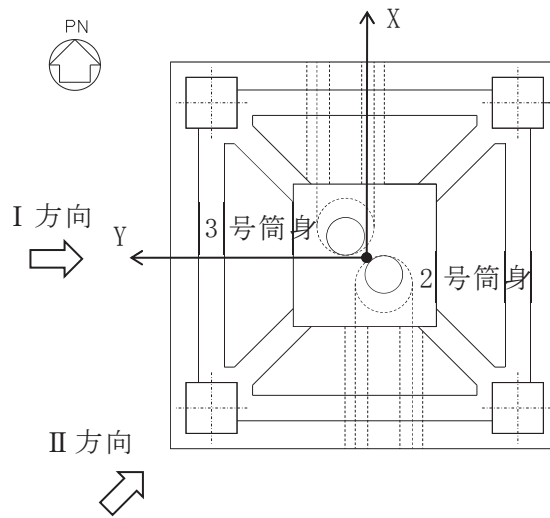
図 2-1 風荷重作用方向の説明
