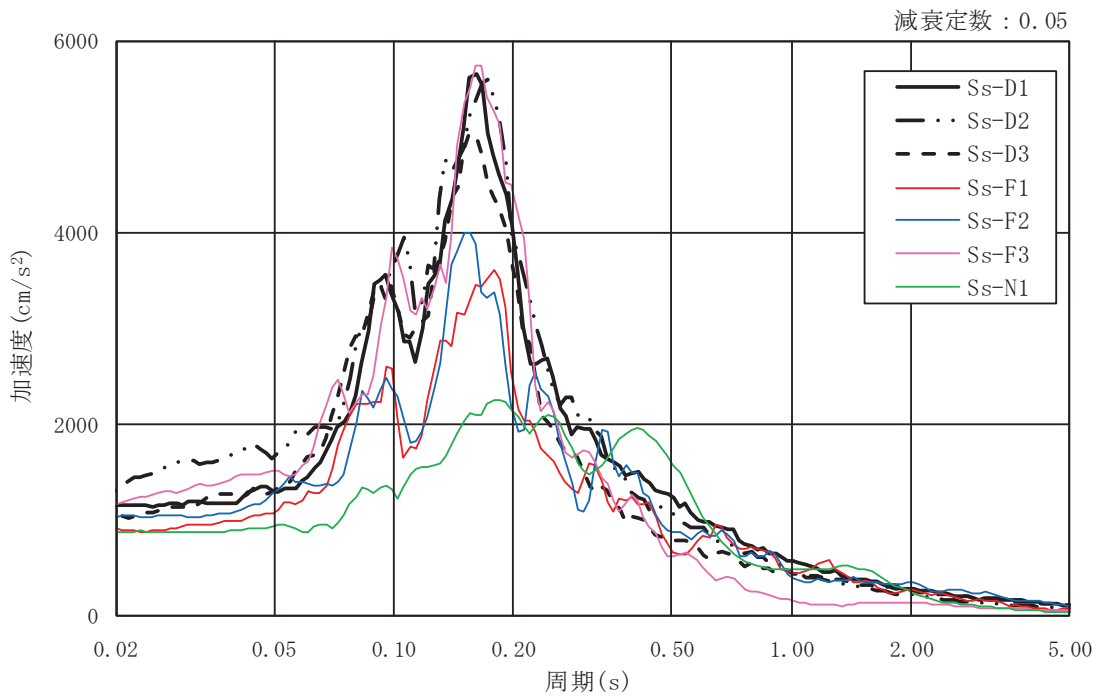
図 3-5(4) 入力地震動の加速度応答スペクトル (基準地震動 S_s , EW 断面 並進成分)
