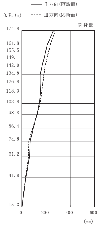
(i) S s - F 2 (直交方向)
