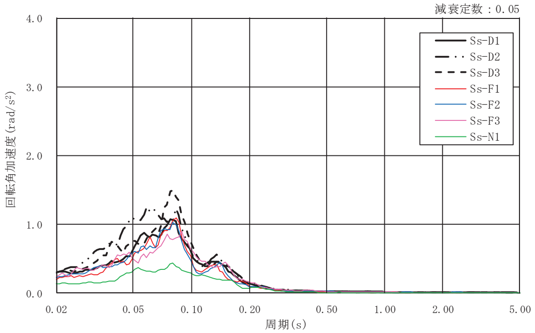
図 3-5(3) 入力地震動の加速度応答スペクトル (基準地震動 S_s , NS 断面 回転成分)
