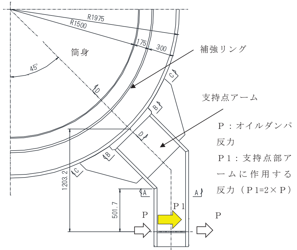
図 4-1(2) 制震オイルダンパ支持点平面図及び支持点荷重 (2/2)
