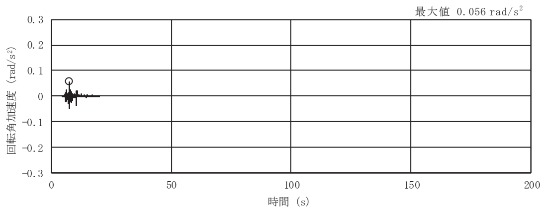
図 3-4(9) 入力地震動の加速度時刻歴波形 (弾性設計用地震動 S d, NS 断面 回転成分) (3/3)
