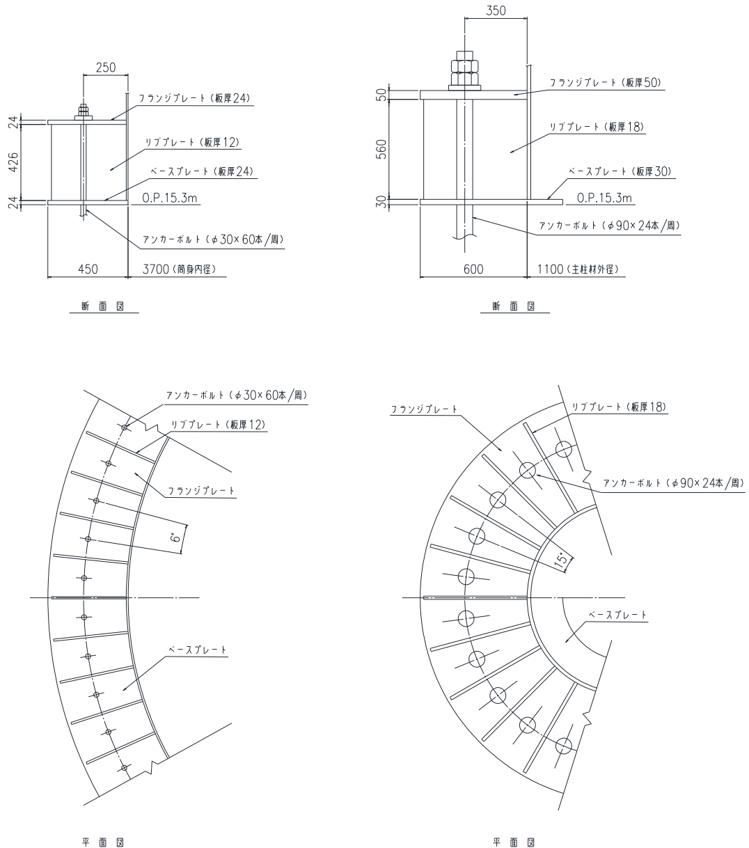
(a) 筒身脚部
