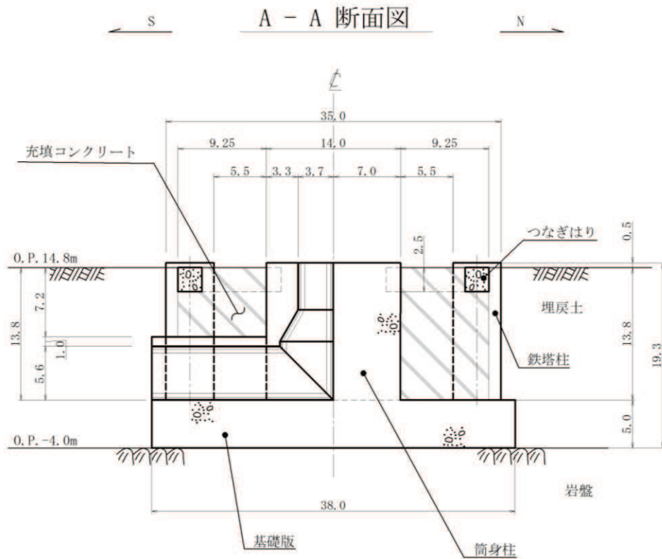
図 2-5 排気筒基礎断面図 (A-A 断面, NS 断面) (単位 : m)
