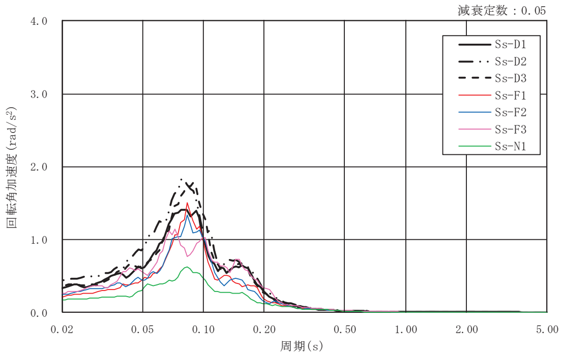
図 3-5(6) 入力地震動の加速度応答スペクトル (基準地震動 S_s , EW 断面 回転成分)
