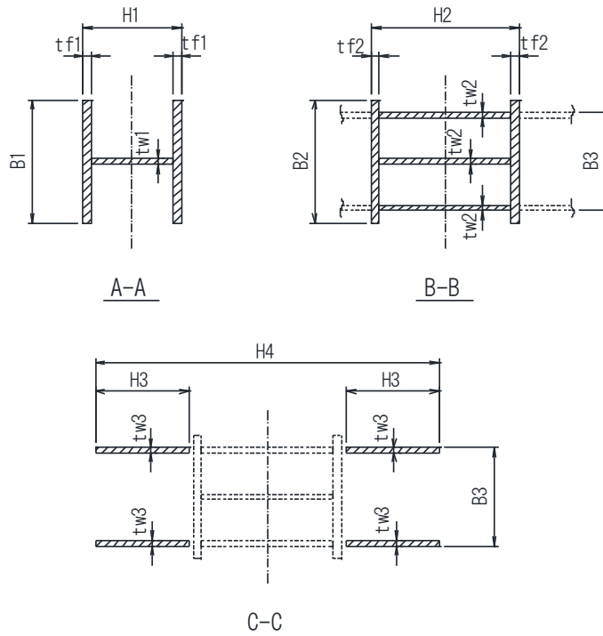
図 4-2(1) 支持点アームの構成断面 (単位: mm) (1/2)
