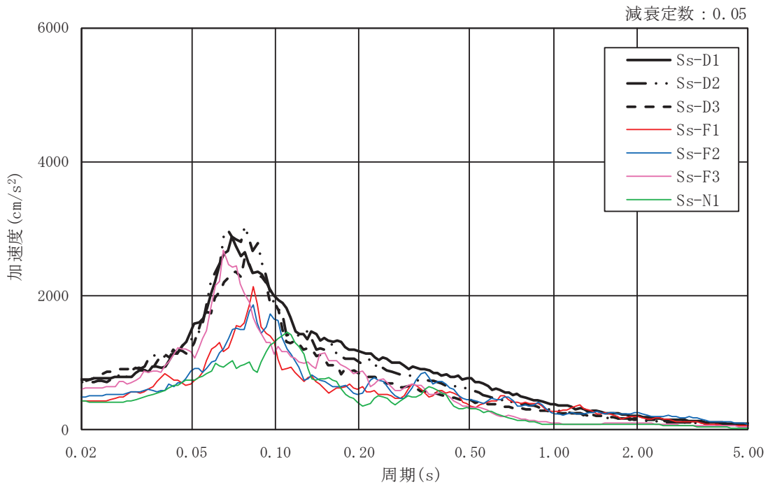
図 3-5(5) 入力地震動の加速度応答スペクトル (基準地震動 S_s , EW 断面 鉛直成分)
