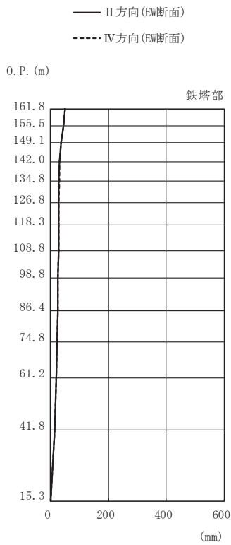
図 4-7(6) 最大応答変位 (弾性設計用地震動 S d) (6/7)
