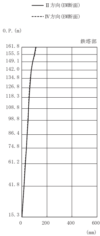
図 4-7(5) 最大応答変位 (弾性設計用地震動 S d) (5/7)
