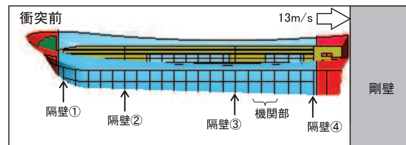
船尾方向からの衝突解析
