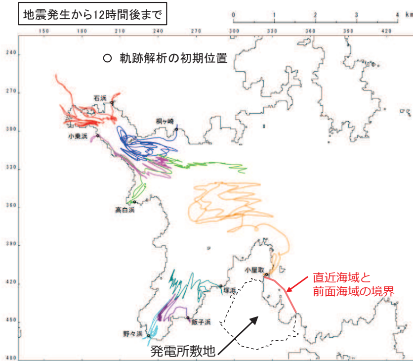
主な漁港を初期位置とした軌跡解析結果
