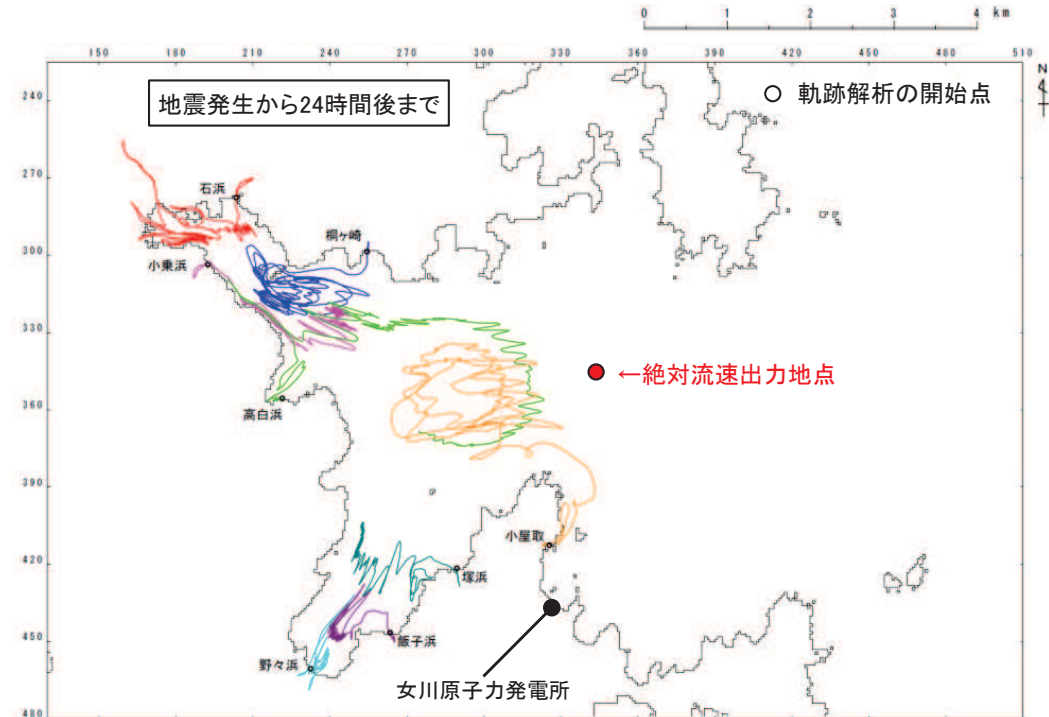
軌跡解析結果(基準津波)
