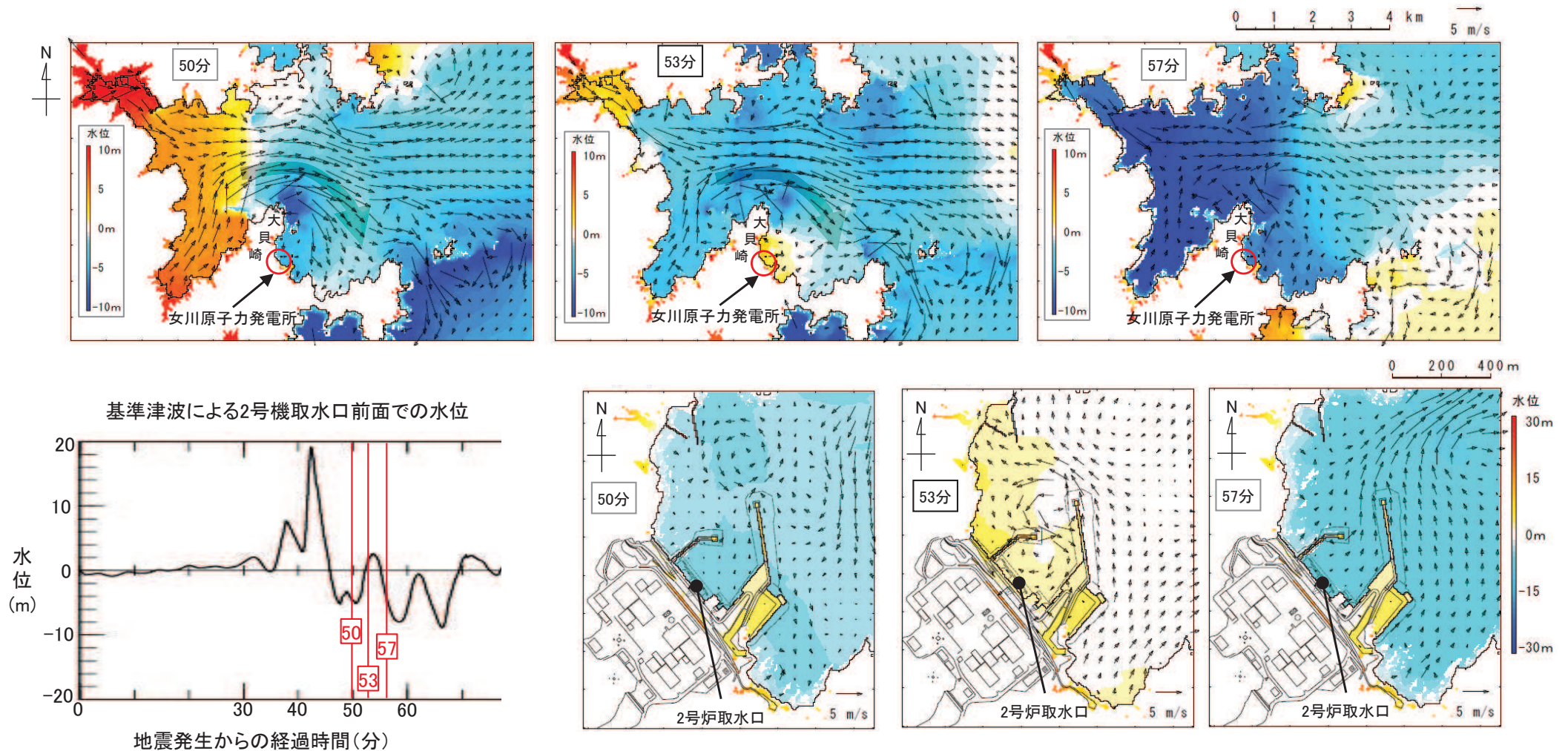
図 発電所周辺海域の水位・流向ベクトル(基準津波)
