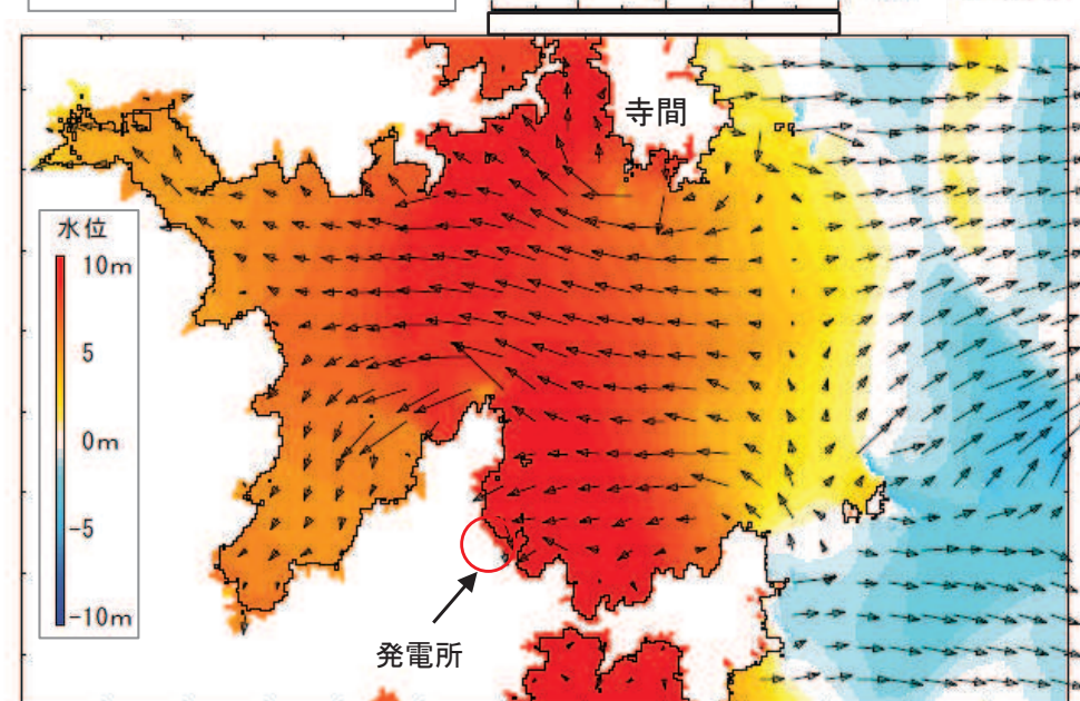
発電所に津波第一波が到達する約42分の流向・流速の分布
