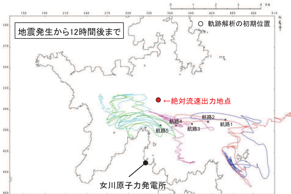
軌跡解析結果
