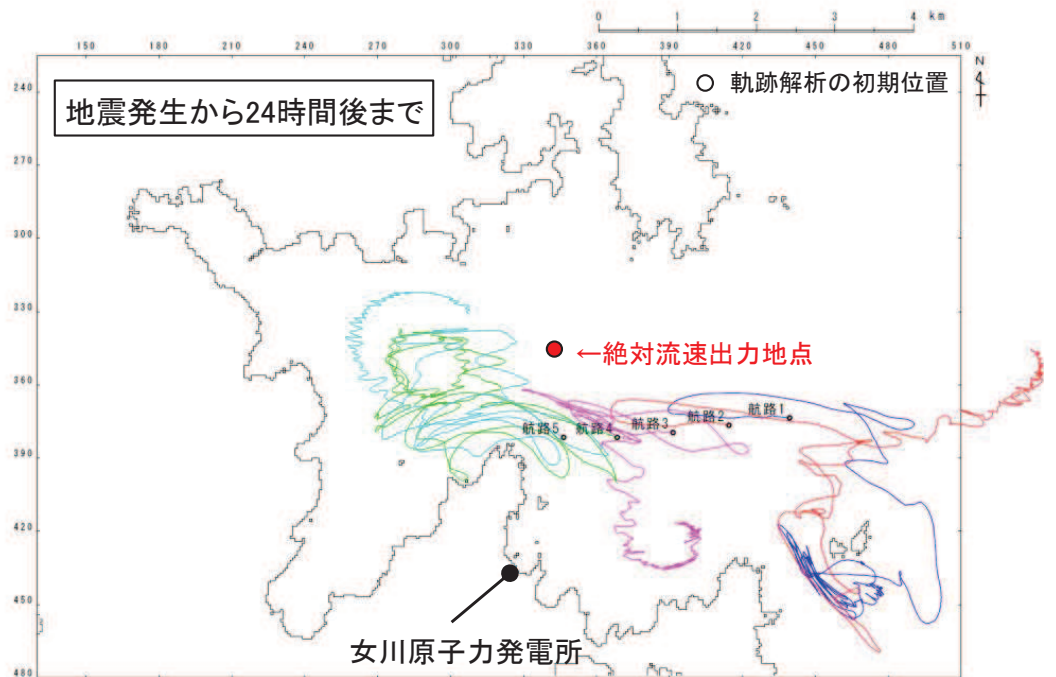
軌跡解析結果
