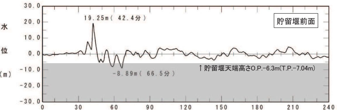
水位時刻歴波形
