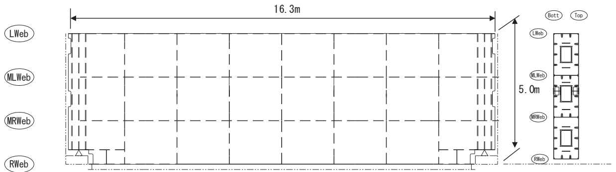
図 2.2-9(3) 鋼製遮水壁（鋼桁 6） 鋼桁構造図
