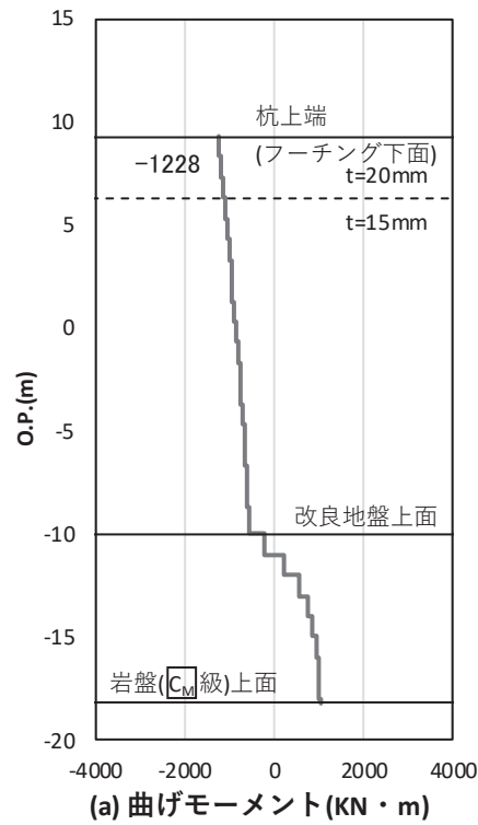
図 4-47(4) 基礎地盤の支持性能照査時刻での軸力（引き抜き） (鋼桁 4：基礎 2, S s - N 1 (-+), 桁軸直交方向加振時, t = 7.90 s)
