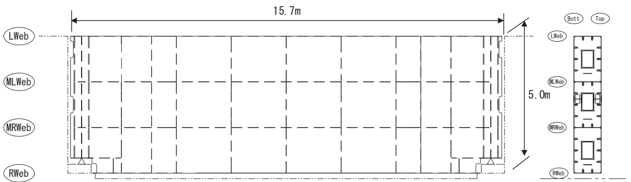
图 2.2—6(3) 鋼製遮水壁（鋼桁 3） 鋼桁詳細図
