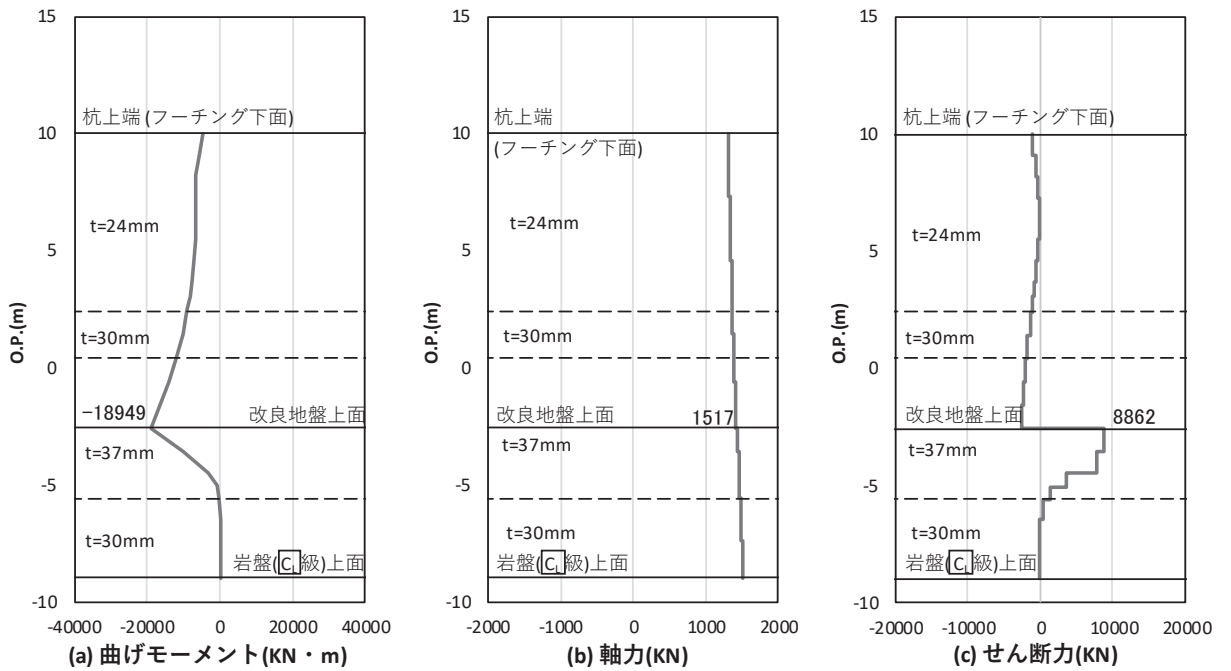
図 4.1-30(1) 鋼管杭のせん断破壊に対する照査における照査時刻での断面力
