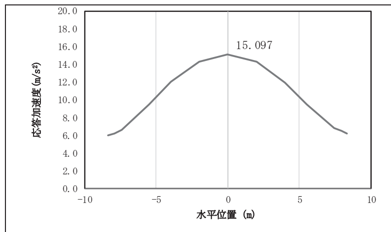
図 4.1-8(17) 鋼桁の応答震度分布 (鋼桁 2, S s-F 3 (++))
