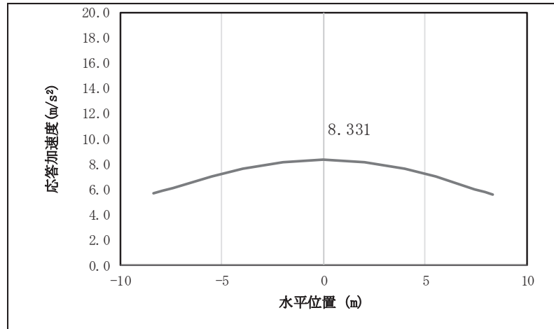
図 4.1-8(19) 鋼桁の応答震度分布 (鋼桁 2, S s -N1 (++) )
