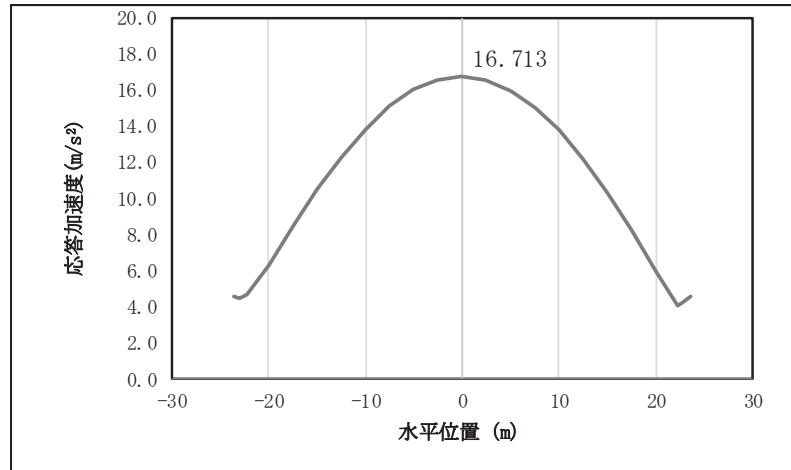
図 4.1-10(19) 鋼桁の応答震度分布 (鋼桁 4, S s -N 1 (++) )
