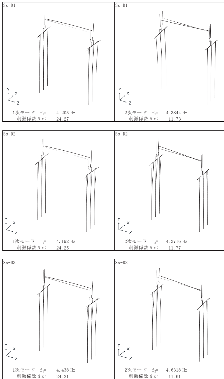
図 3.2-4(1) 固有値解析結果 (鋼桁 2 : モード図) 鋼桁軸直交方向
