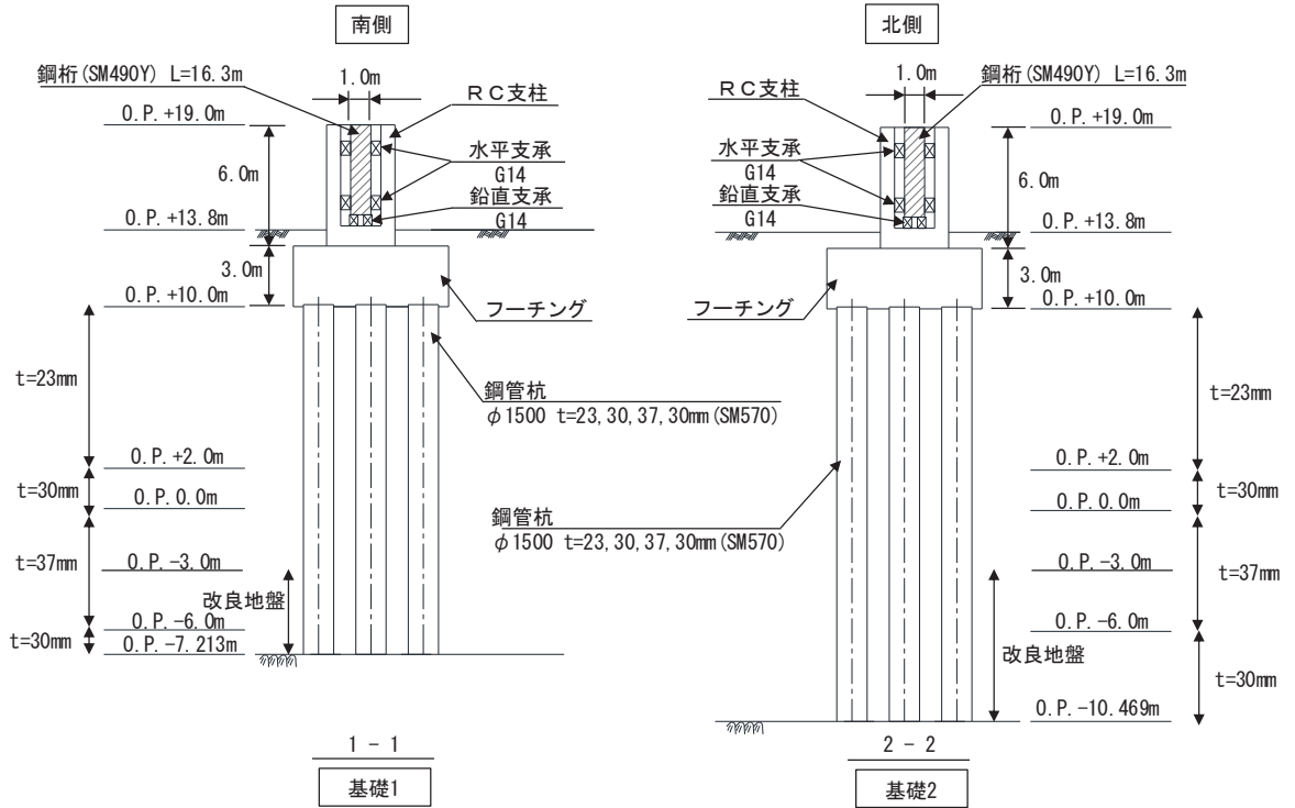
(断面図)
