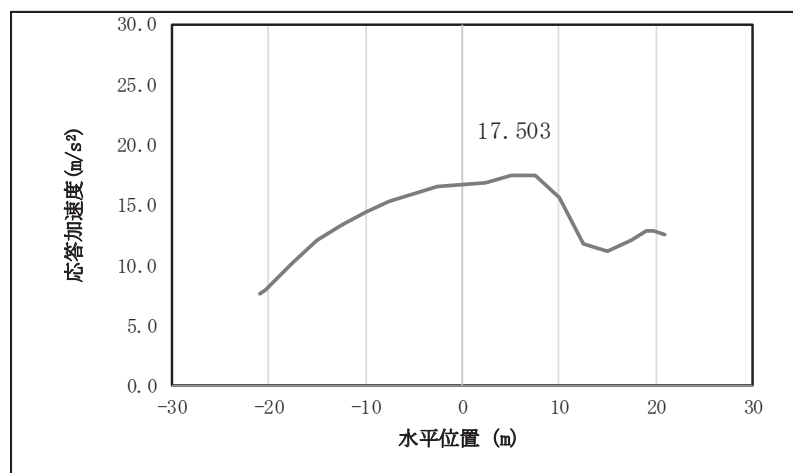
図 4.1-7(12) 鋼桁の応答震度分布 (鋼桁 1, S s-D 3 (--))
