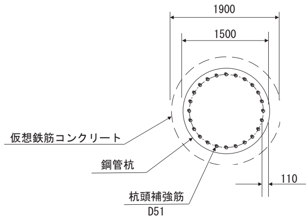
図 4.5-1 杭頭配筋概要図（鋼製扉 2 の例）
