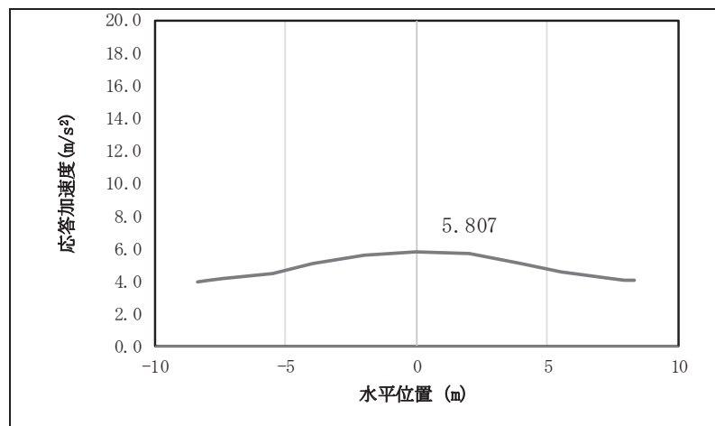
図 4.1-8(14) 鋼桁の応答震度分布 (鋼桁 2, S s - F 1 (-+) )
