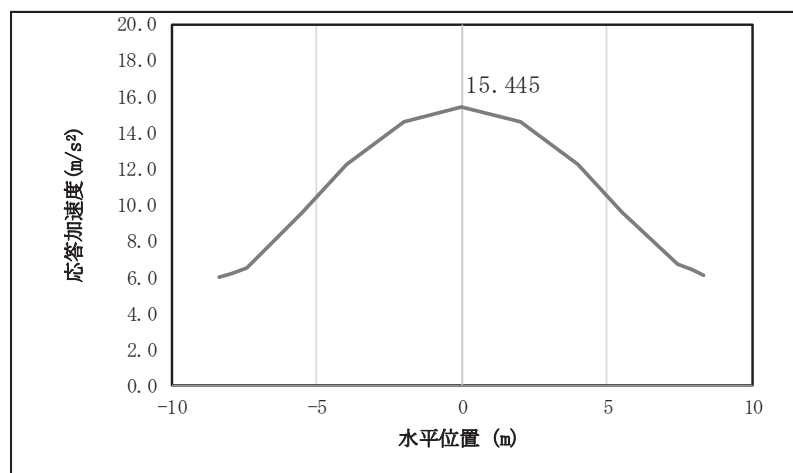
図 4.1-8(18) 鋼桁の応答震度分布 (鋼桁 2, S s-F 3 (-+))
