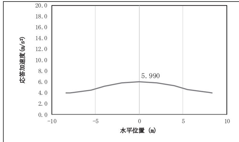
図 4.1-8(13) 鋼桁の応答震度分布 (鋼桁 2, S s - F 1 (++) )
