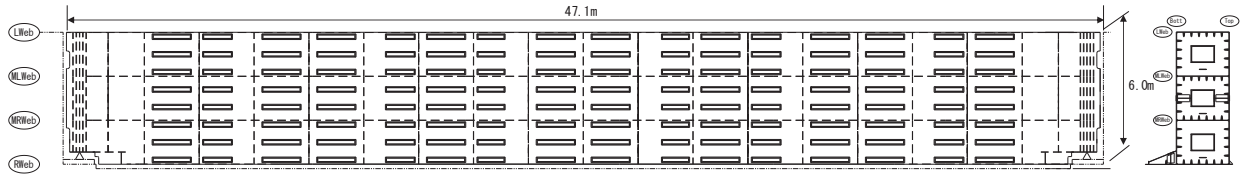
圖 2.2-7(3) 鋼製遮水壁 (鋼桁 4) 鋼桁構造圖
