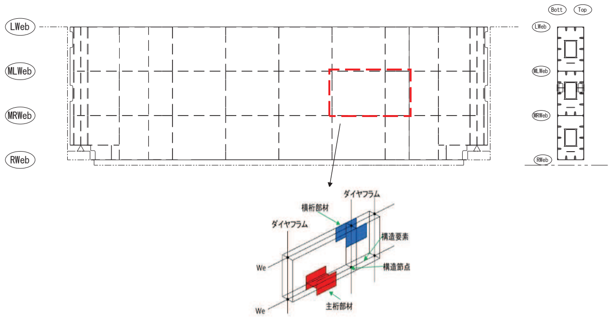
図 3.4-1 鋼桁詳細図
