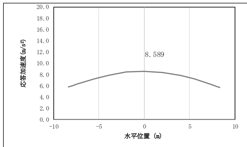
図 4.1-8(20) 鋼桁の応答震度分布 (鋼桁 2, S s -N1 (-+) )
