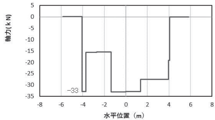
(b) 軸力
