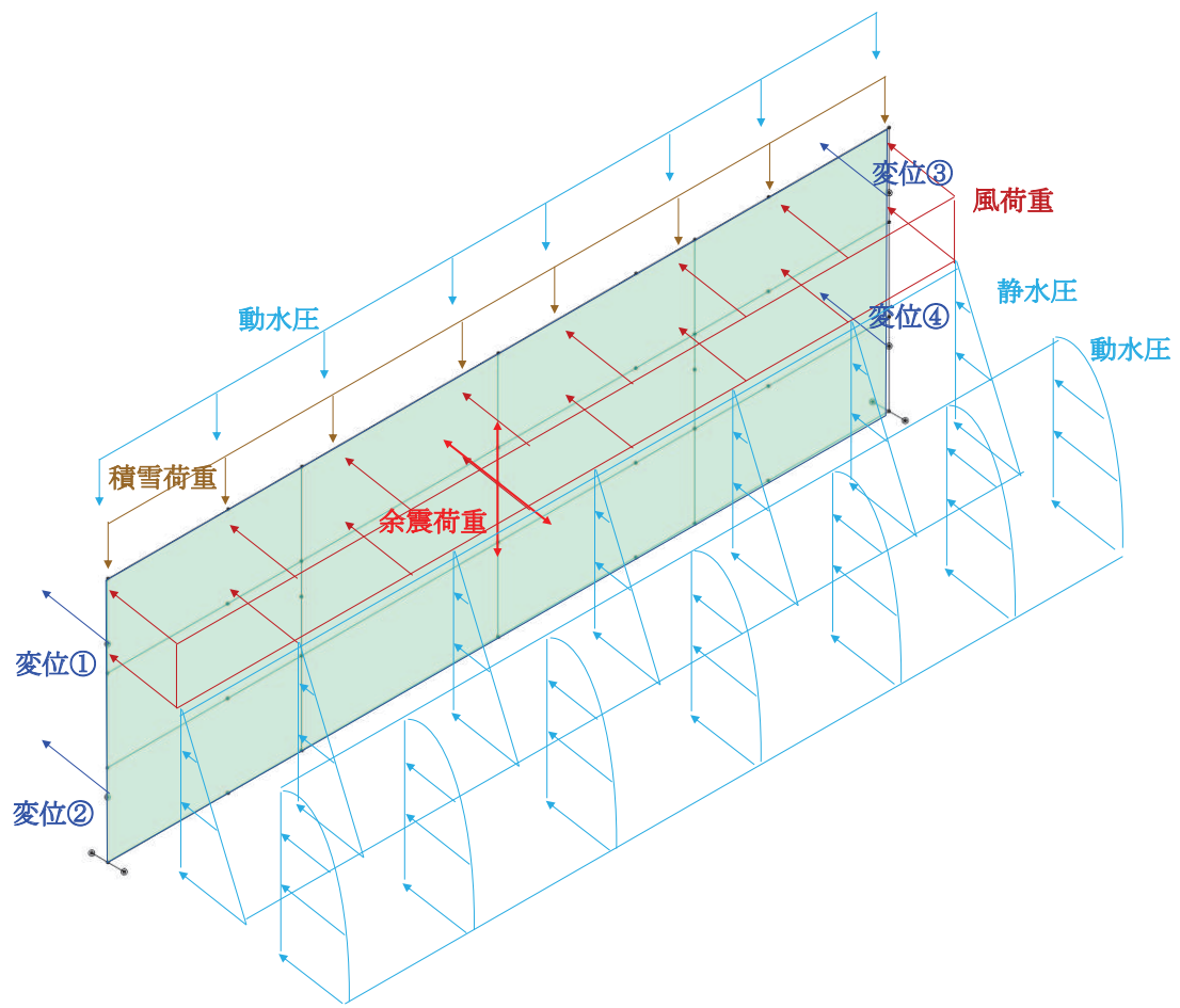
図 3.5-37 作用荷重図
