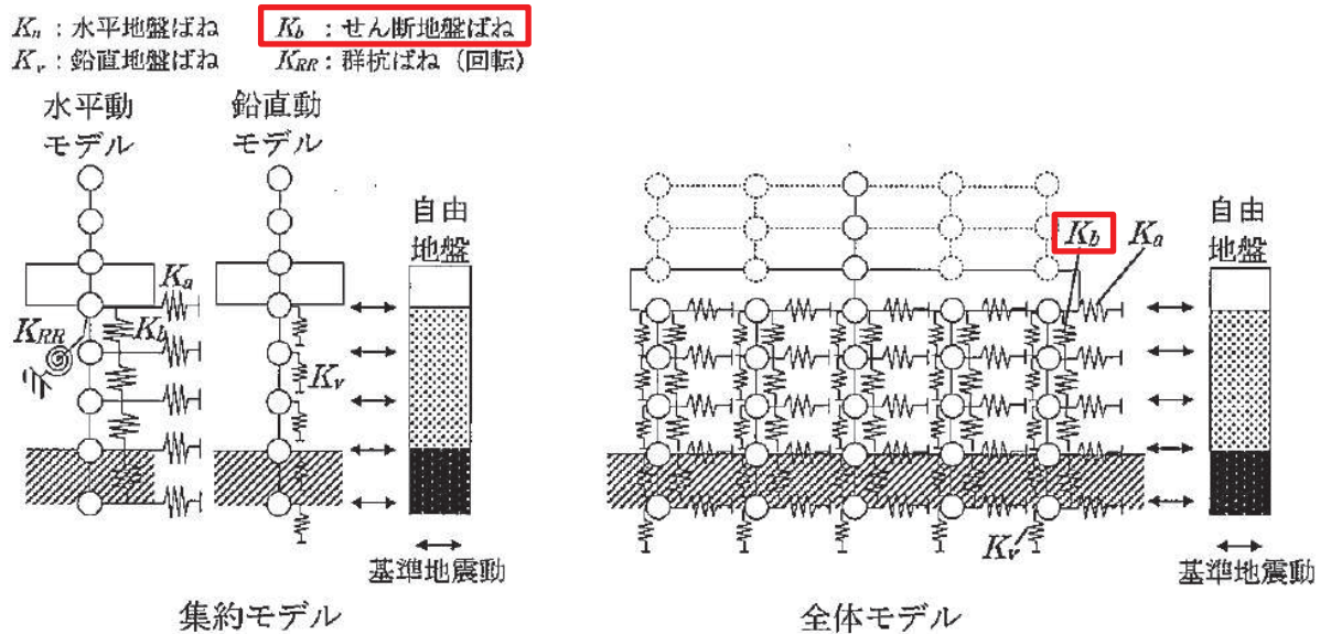
附図2.6-1 質点系モデル
