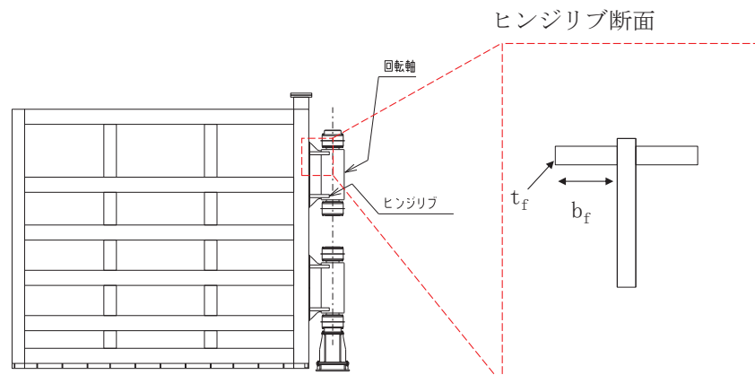
図 3.7-10 扉体詳細図（ヒンジリブ断面の例）
