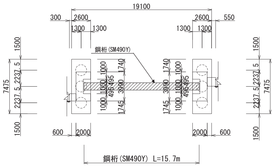
图 2.2—6(2) 鋼製遮水壁（鋼桁 3） 平面図
