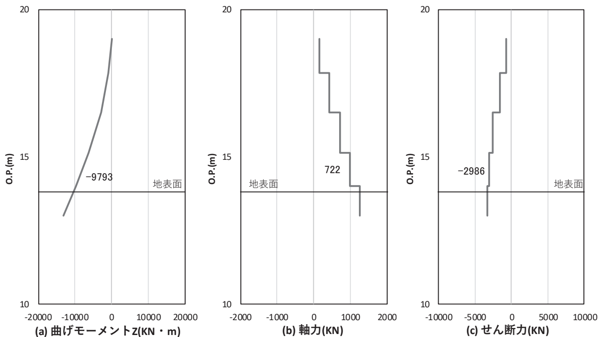
図 4.1-16(2) コンクリート及び鉄筋のせん断破壊に対する照査における照査時刻での断面力 (鋼桁 3 : 基礎 2, S s - D 2 ( + + ), 桁軸直交方向加振時, t = 17.75s )
