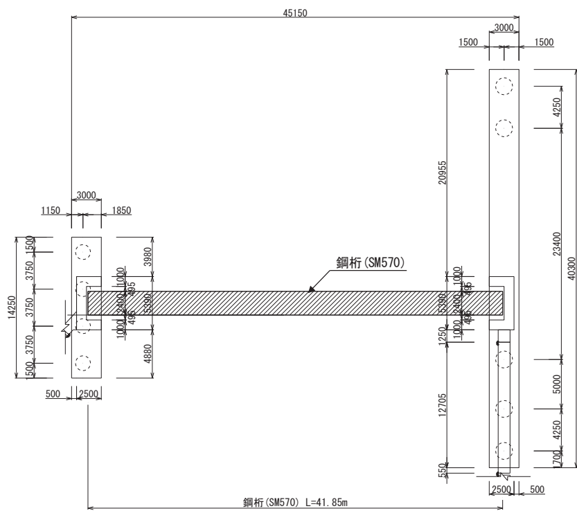
图 2.2-4(2) 鋼製遮水壁 (鋼桁 1) 平面图
