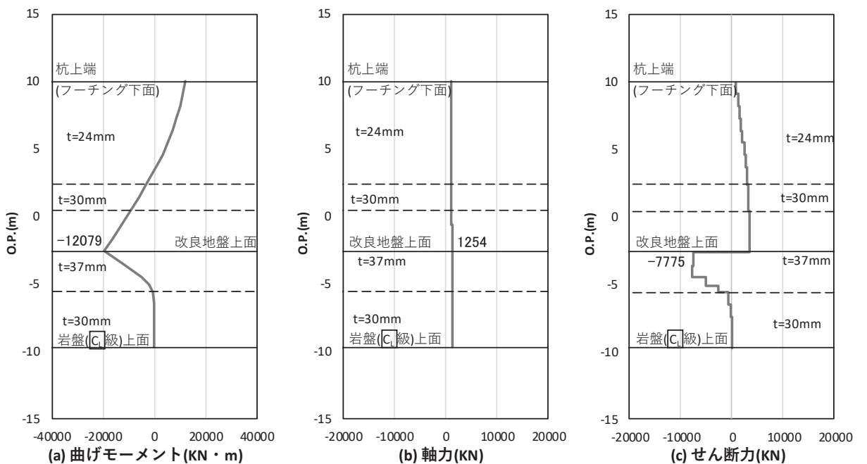
図 4.1-30(2) 鋼管杭のせん断破壊に対する照査における照査時刻での断面力
