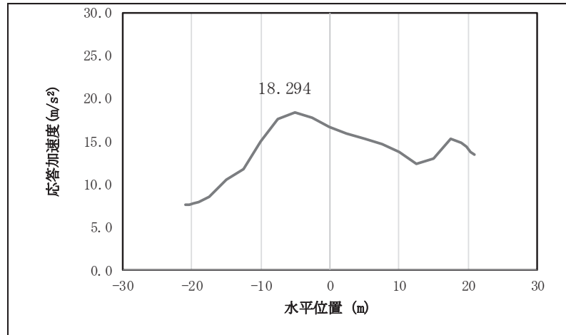
図 4.1-7(10) 鋼桁の応答震度分布 (鋼桁 1, S s-D 3 (-+))
