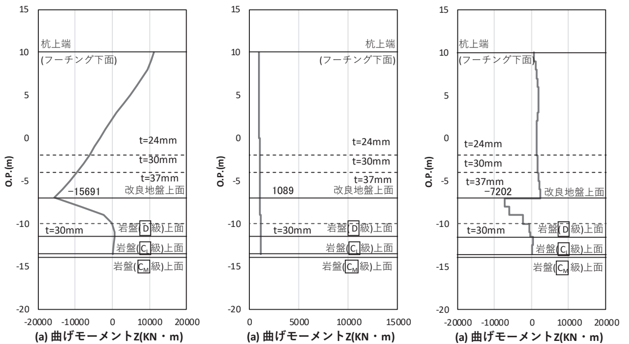
図 4.1-38(2) 鋼管杭のせん断破壊に対する照査における照査時刻での断面力
