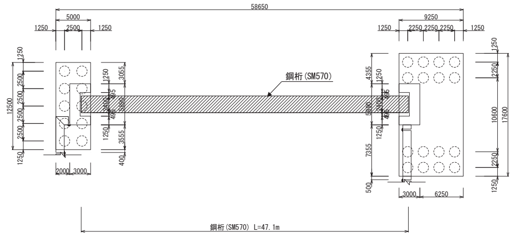
圖 2.2-7(2) 鋼製遮水壁 (鋼桁 4) 平面圖
