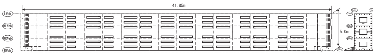
图 2.2-4(3) 鋼製遮水壁 (鋼桁 1) 鋼桁構造图
