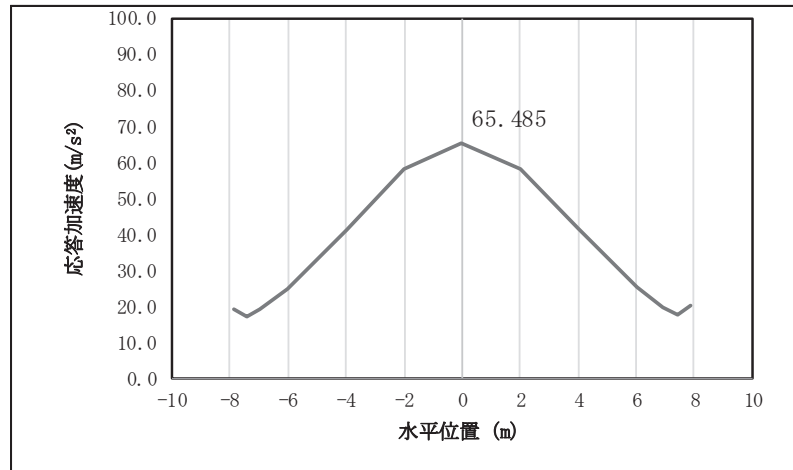
図 4.1-9(4) 鋼桁の応答震度分布 (鋼桁 3, S s-D 1 ( - - ) )
