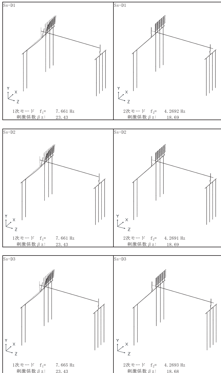
図 3.2-3(3) 固有値解析結果 (鋼桁 1 : モード図) 鋼桁軸方向
