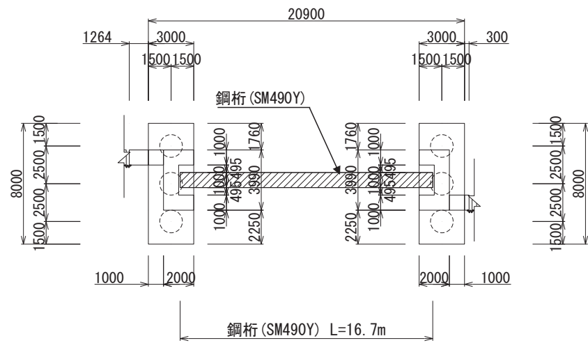
図 2.2-5(2) 鋼製遮水壁 (鋼桁 2) 平面図
