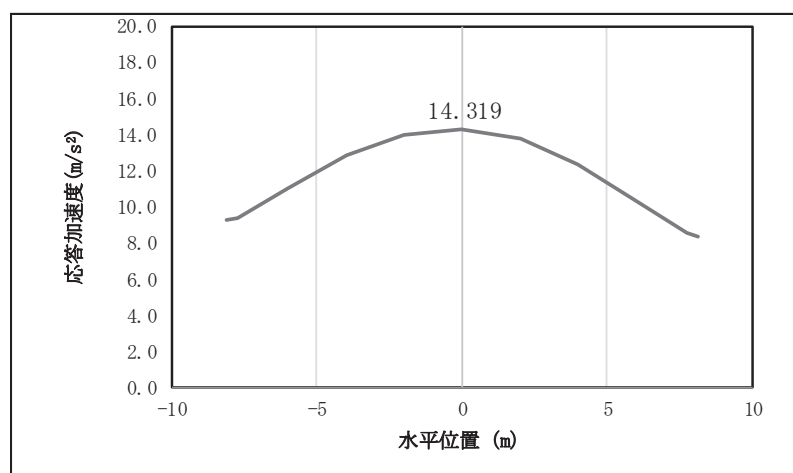
図 4.1-12(12) 鋼桁の応答震度分布 (鋼桁 6, S s-D 3 (--))
