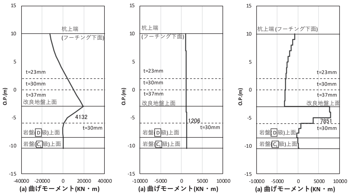
図 4.1-36(2) 鋼管杭のせん断破壊に対する照査における照査時刻での断面力
