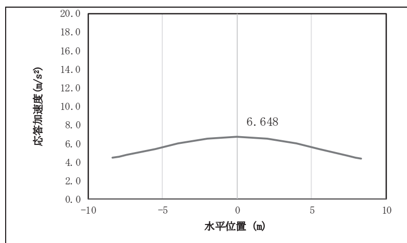
図 4.1-8(15) 鋼桁の応答震度分布 (鋼桁 2, S s - F 2 (++) )
