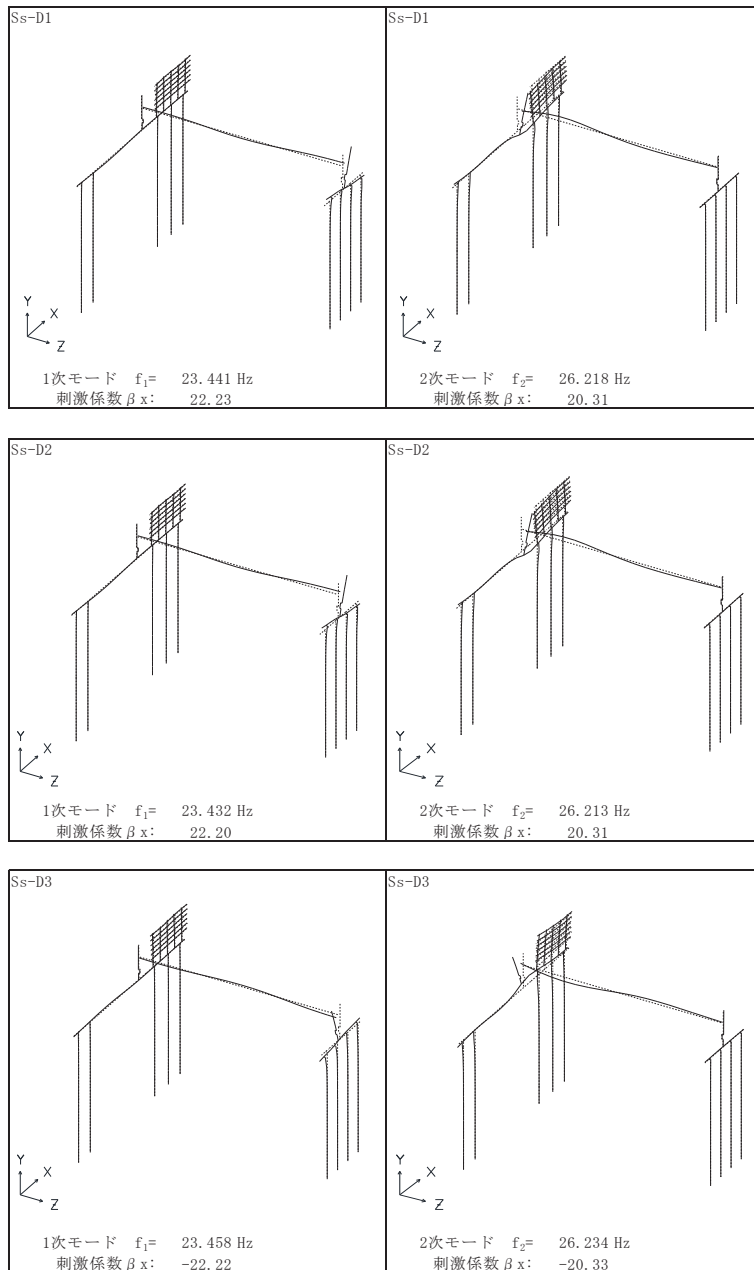
図 3.2-3(1) 固有値解析結果 (鋼桁 1 : モード図) 鋼桁軸直交方向
