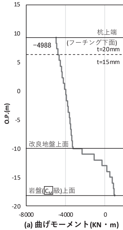
図 4-47(3) 基礎地盤の支持性能照査時刻での軸力（引き抜き） (鋼桁 4：基礎 2, S s - N 1 (-+), 桁軸方向加振時, t = 7.90 s)
