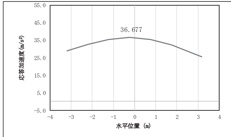
図 4.2-1(4) 扉体の応答震度分布 (鋼製扉 2, S s-D 1 (一一))
