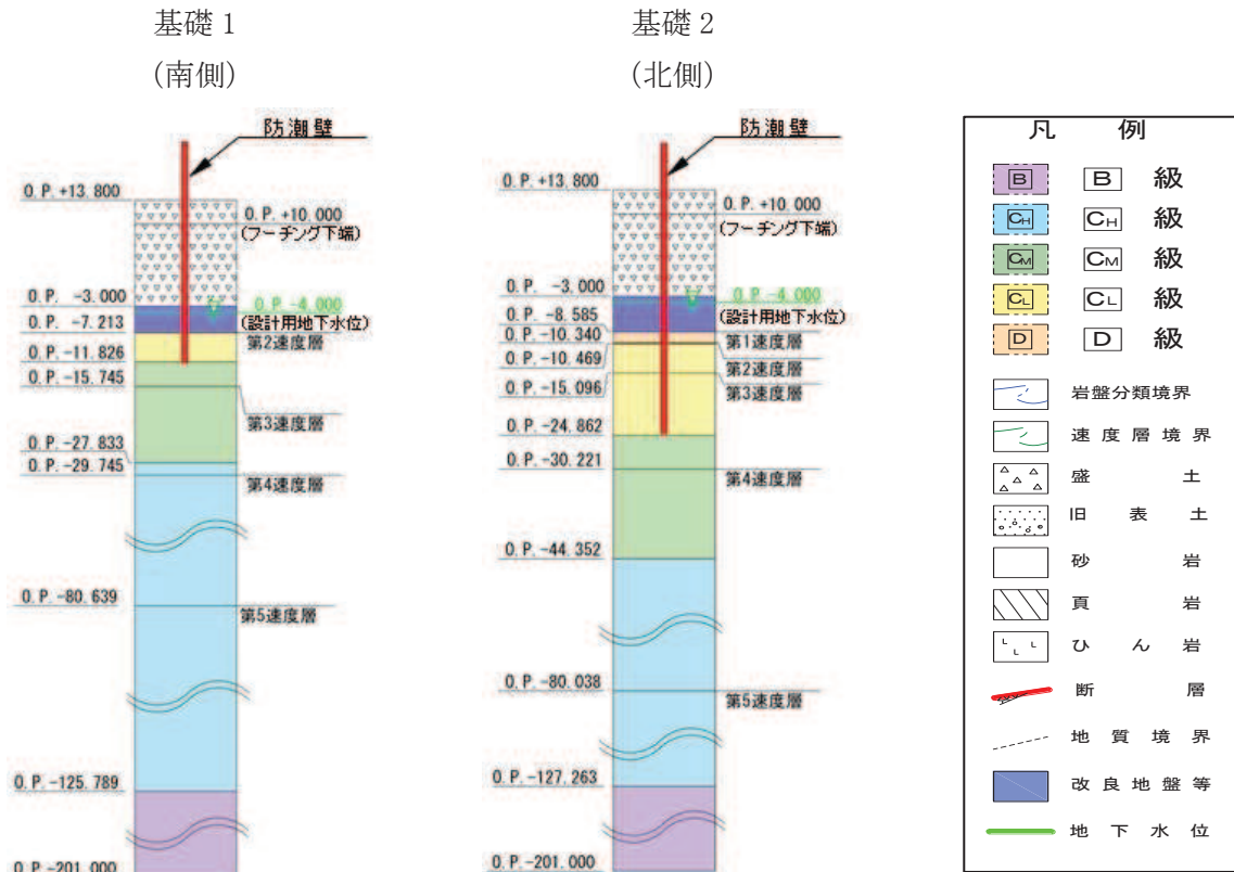
図 3.2-2(5) 評価対象断面の地層構成図 (鋼桁5)
