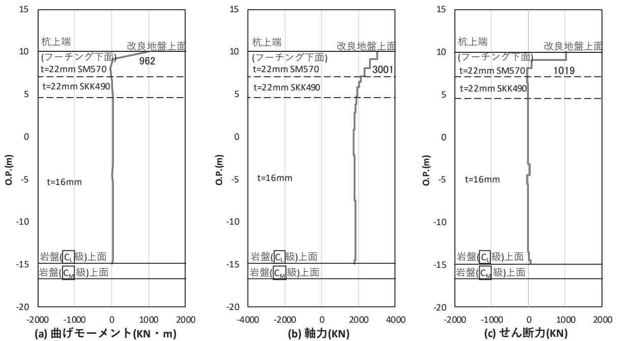
図 4.1-28(2) 鋼管杭のせん断破壊に対する照査における照査時刻での断面力
