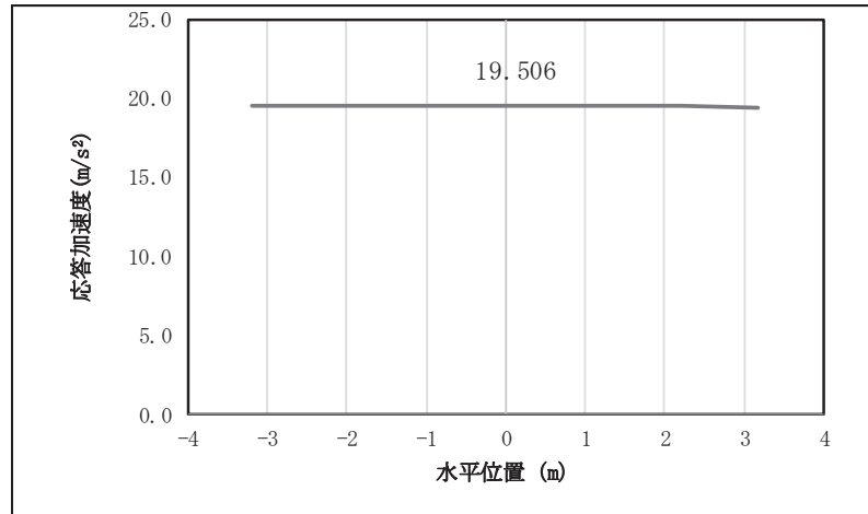
図 4.2-2(4) 扉体の応答震度分布 (鋼製扉 3, S s-D 1 (一一))
