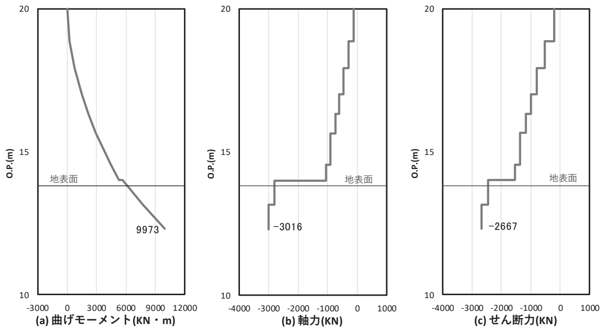
図 4.1-17(1) コンクリートの曲げ・軸力系の破壊に対する照査における
