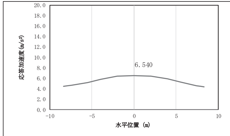
図 4.1-8(16) 鋼桁の応答震度分布 (鋼桁 2, S s-F 2 (-+))
