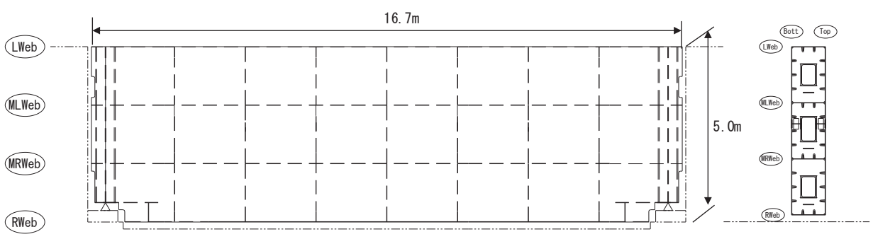
図 2.2-5 (3) 鋼製遮水壁 (鋼桁 2) 鋼桁詳細図
