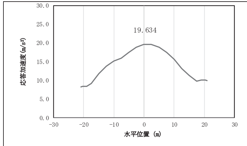
図 4.1-7(19) 鋼桁の応答震度分布 (鋼桁 1, S_s-N1 (++) )
