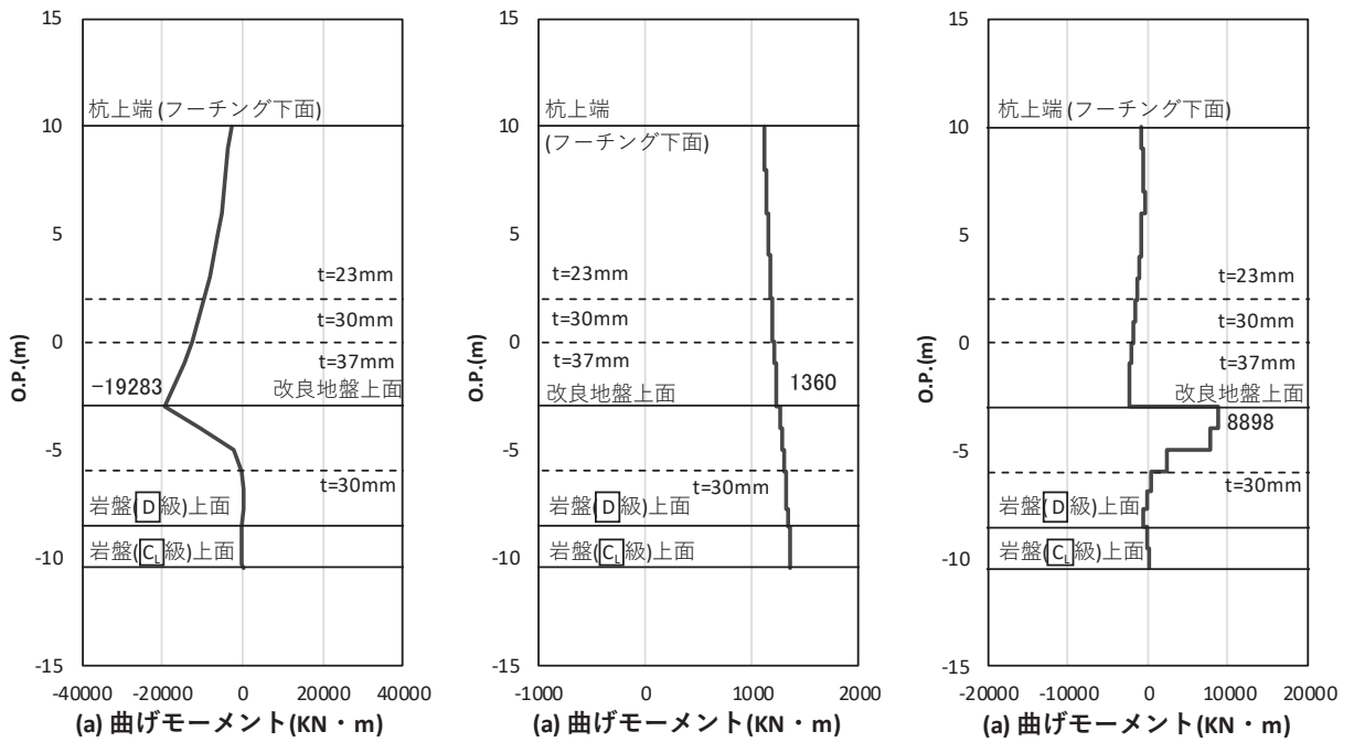
図 4.1-36(1) 鋼管杭のせん断破壊に対する照査における照査時刻での断面力
