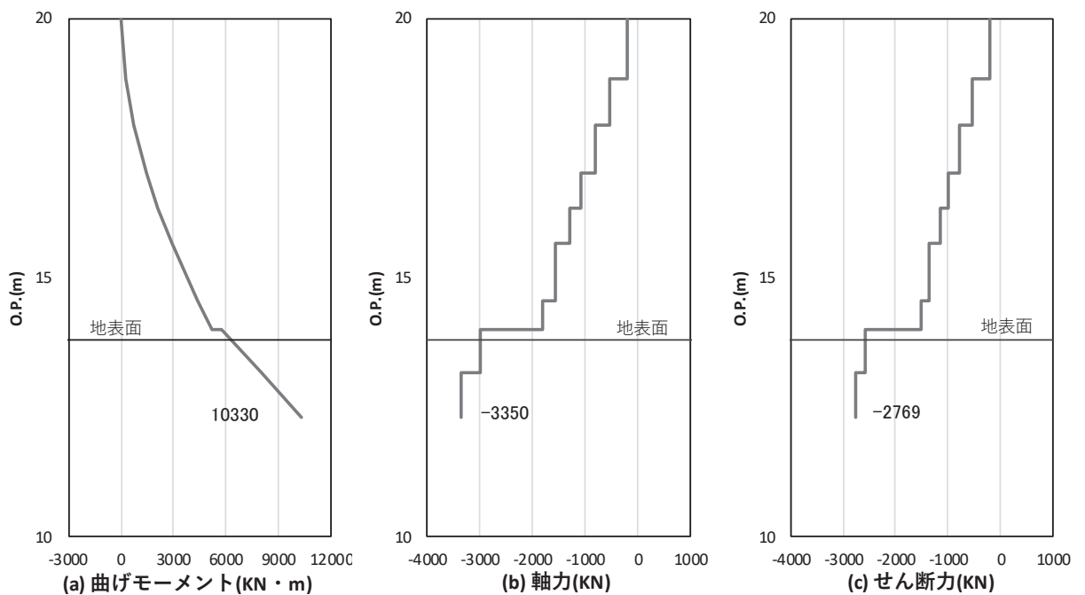
図 4.1-17(2) 鉄筋の曲げ・軸力系の破壊に対する照査における
