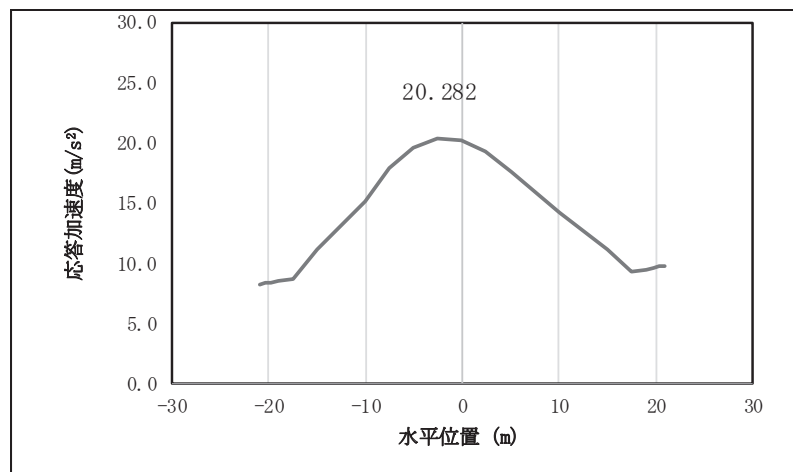
図 4.1-7(20) 鋼桁の応答震度分布 (鋼桁 1, S_s-N1 (-+))
