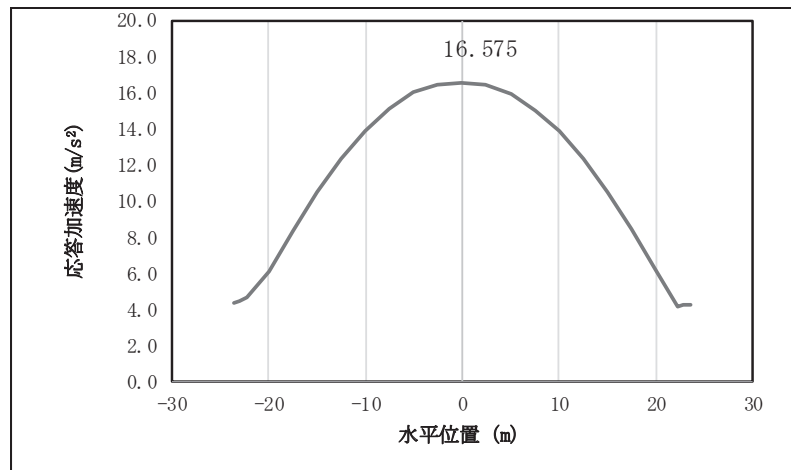
図 4.1-10(20) 鋼桁の応答震度分布 (鋼桁 4, S s -N 1 (-+) )
