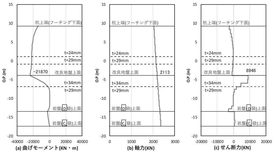
図 4.1-14 鋼管杭の曲げ・軸力系の破壊に対する照査における照査時刻での断面力 (鋼製扉 3, S s - N 1 ( - + ) , t = 7.93s) 解析ケース③：地盤物性のばらつき ( - 1 \sigma ) を考慮した解析ケース
