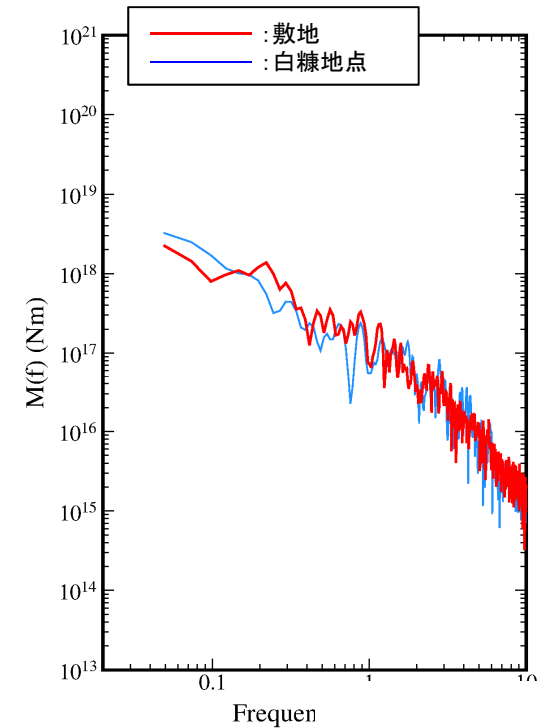
③2001/8/14の地震(M6.4)による観測記録から求めた震源スペクトルの比較
