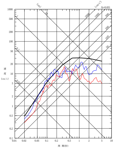
NS成分(PN基準)
