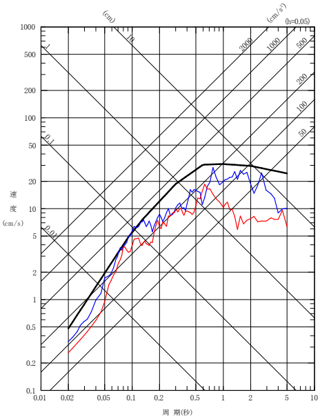
EW成分(PN基準)
