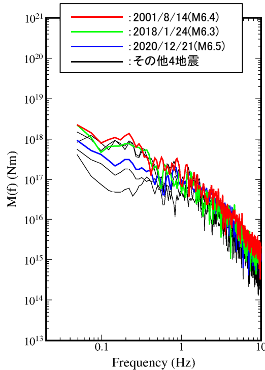
①敷地の観測記録から求めた震源スペクトル
