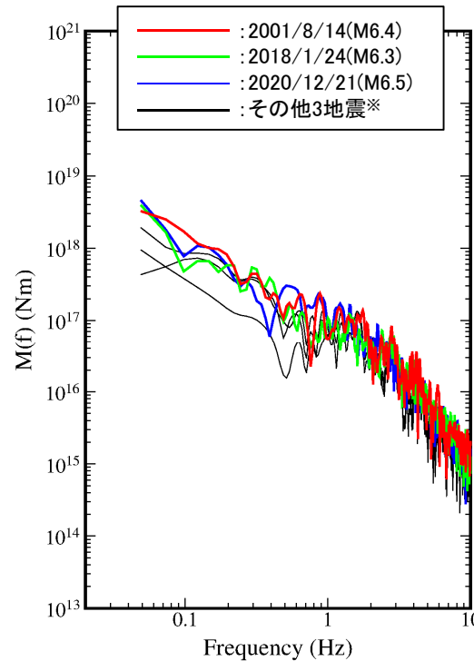
②白糠地点の観測記録から求めた震源スペクトル
