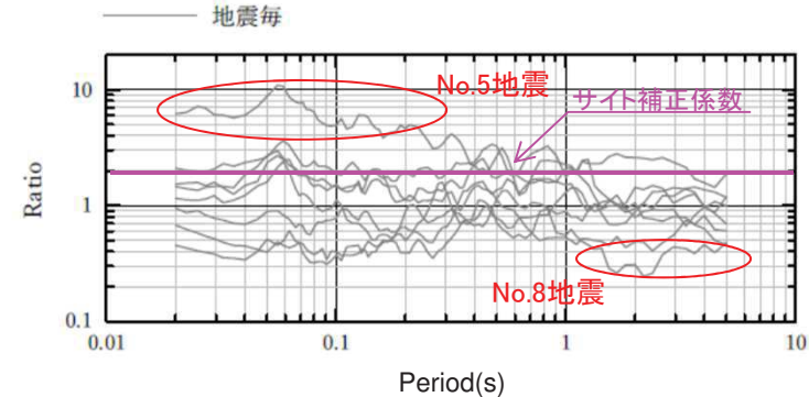
海洋プレート内地震のNoda et al.(2002)に対するサイト補正係数(本資料p.108に一部加筆)
