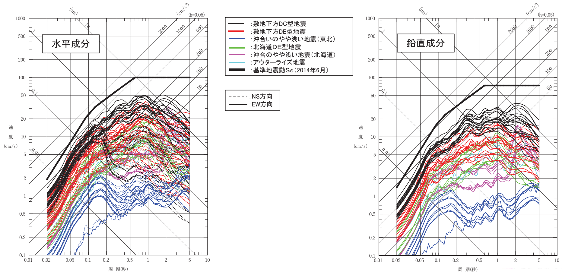
検討対象地震の平均応答スペクトルと申請時の基準地震動Ss
