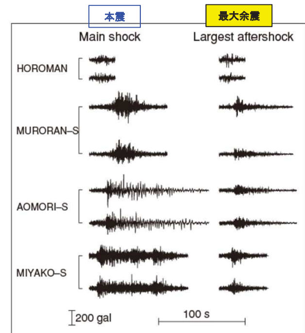
強震記録
