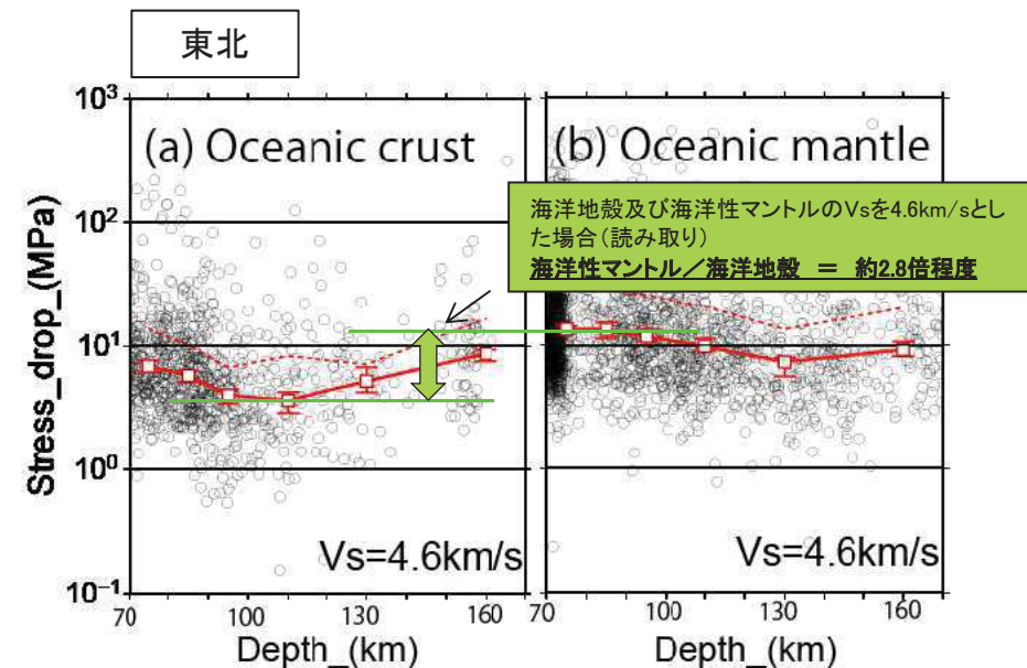
東北日本の海洋プレート内地震の応力降下量 〔北(2016) 一部加筆〕
