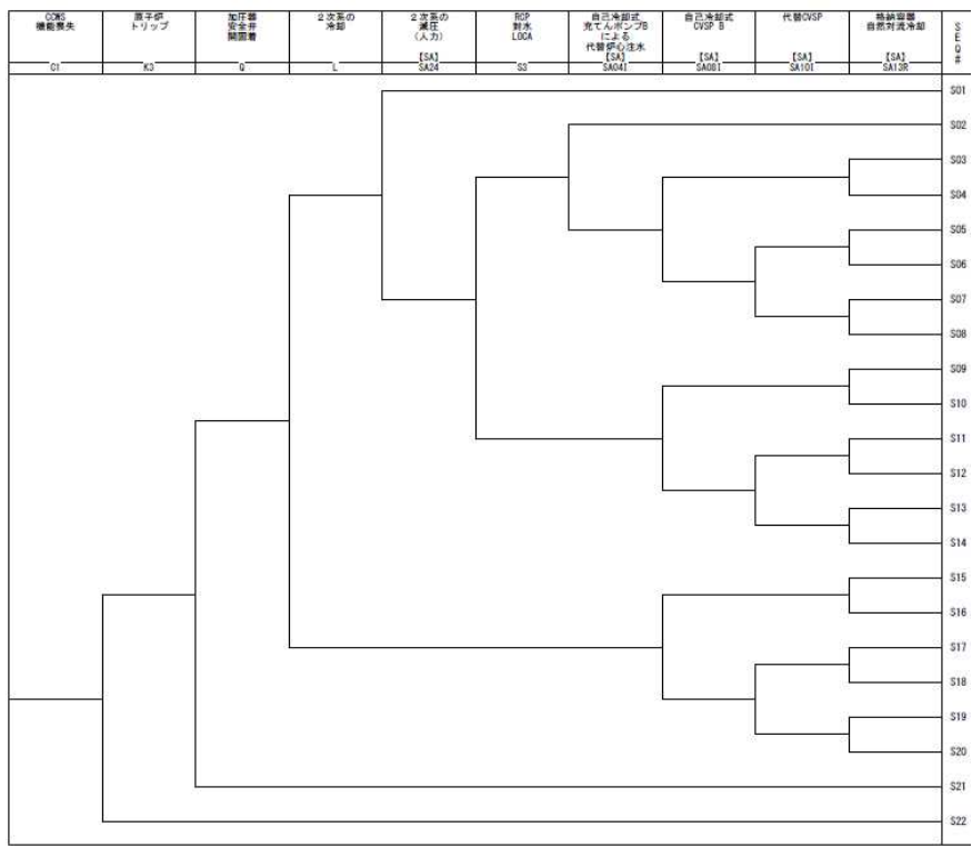
図 3 イベントツリーのイメージ
