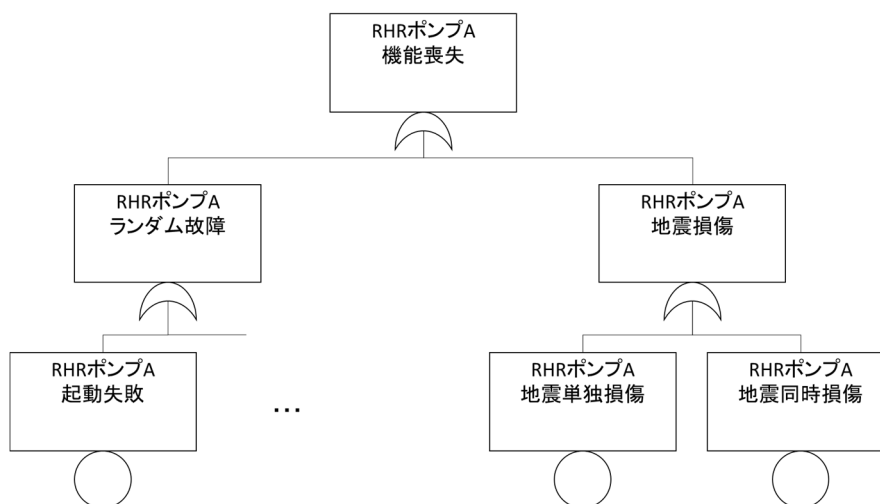
図 1 機器毎のゲート構造
