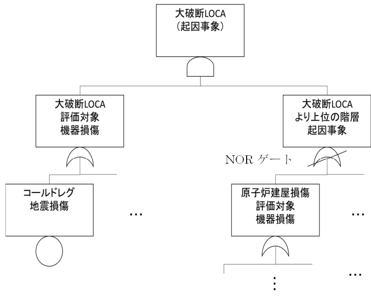
図 2 フォールトツリーのイメージ
