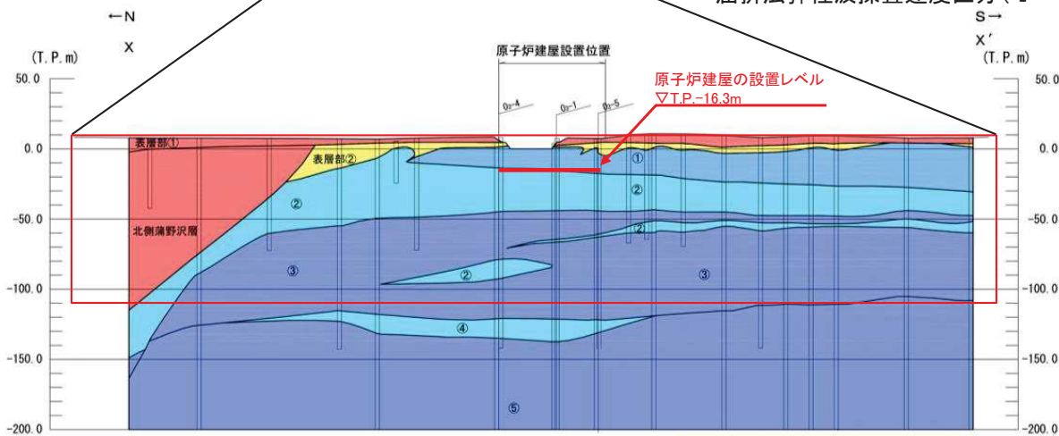
PS検層による速度層断面 (X-X')
