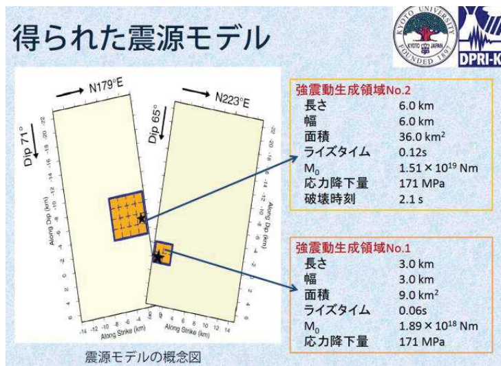
震源モデル
