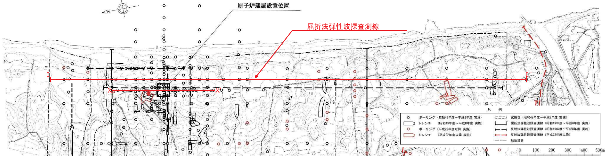
断面位置図
