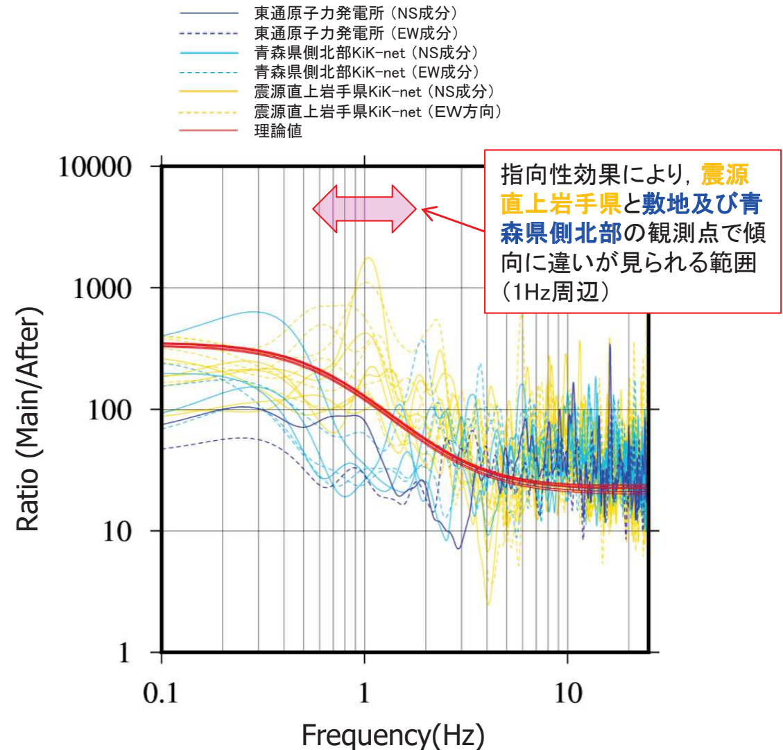
フーリエスペクトル比(スムージング)
