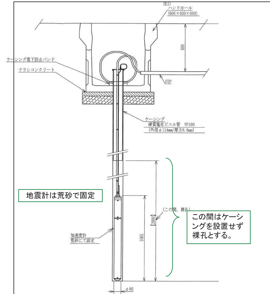
増設地震計[T.P.+2.0m]の設置概要図
