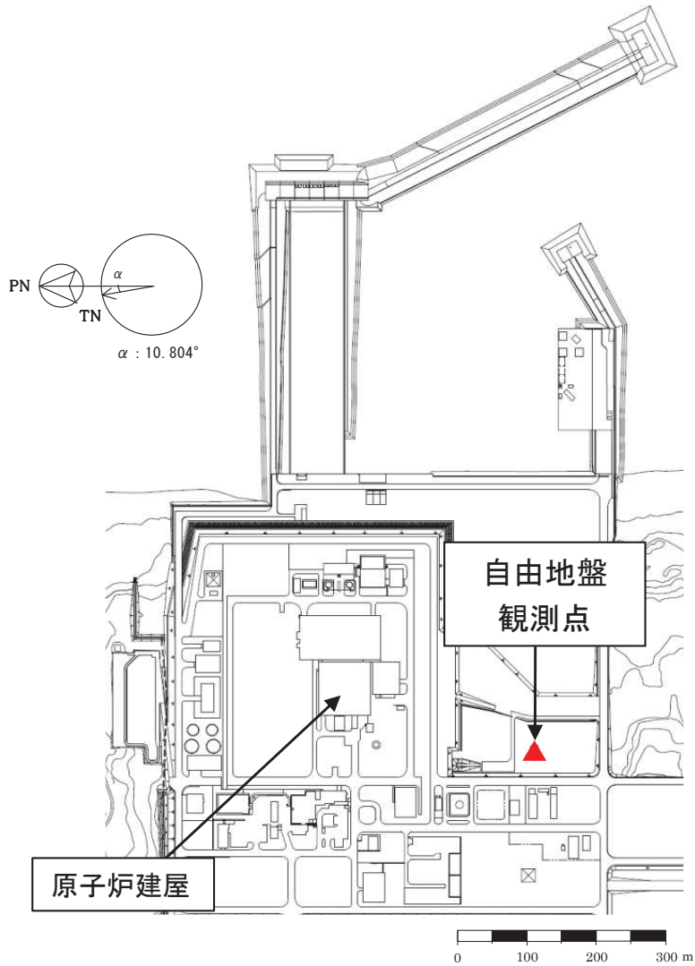
平面配置図
