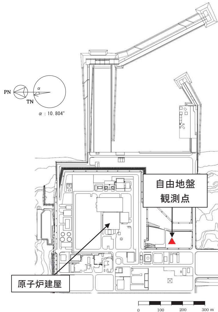
平面配置図
