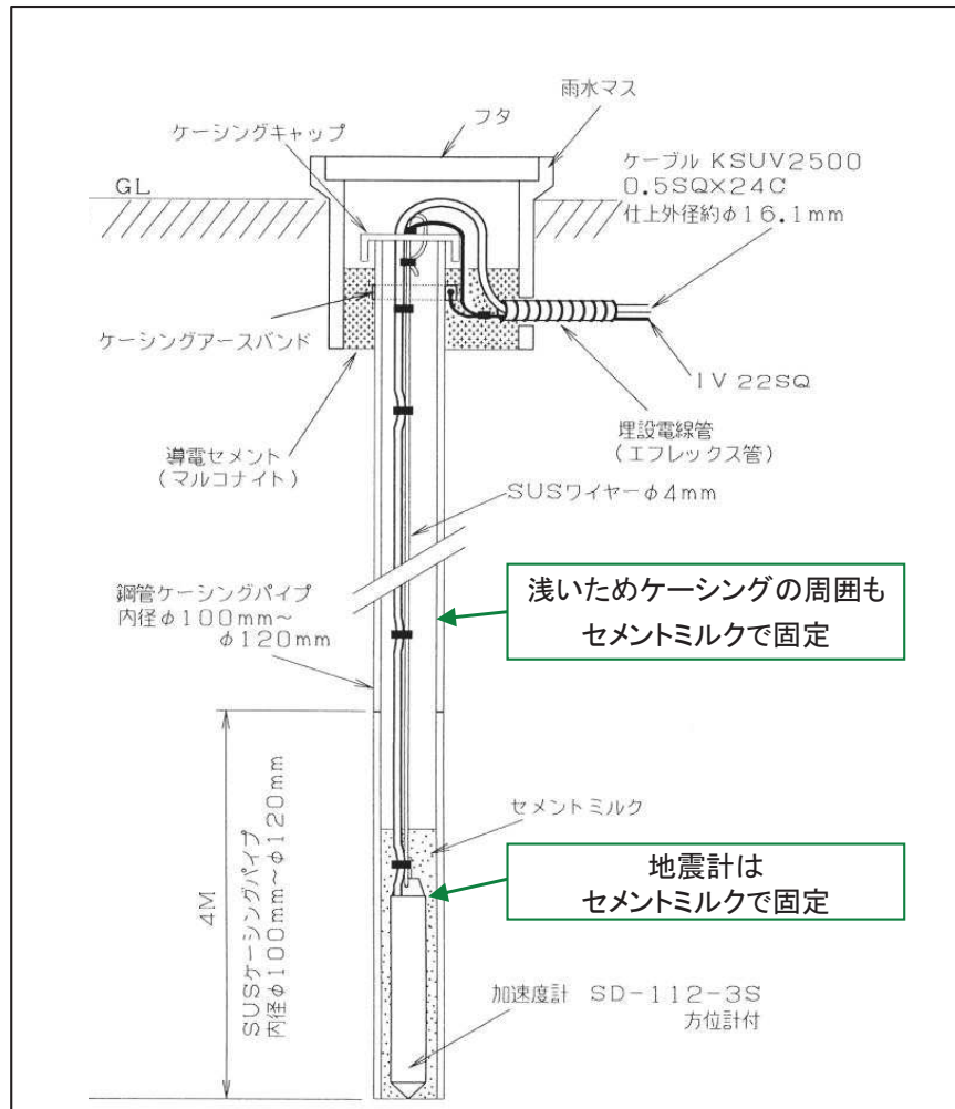
既設地震計[T.P.+2.0m]の設置概要図
