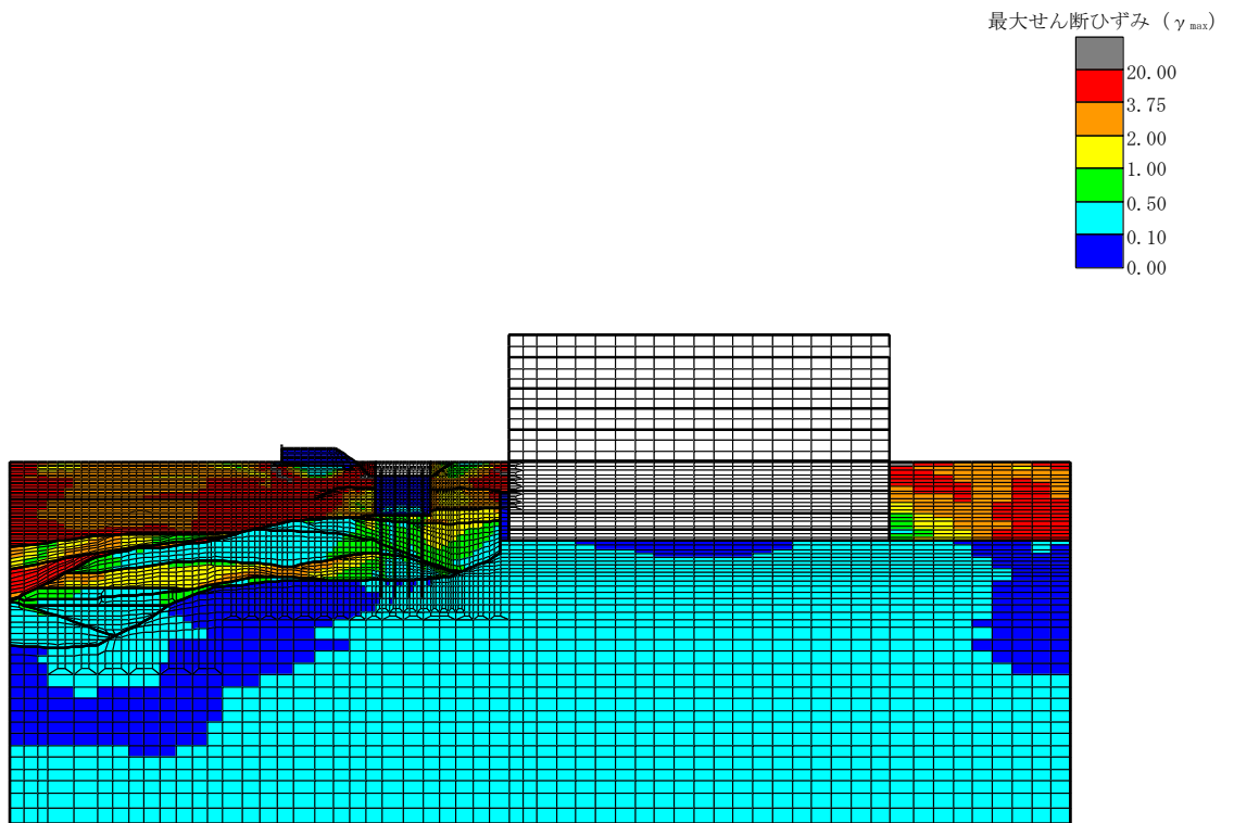
全体図
