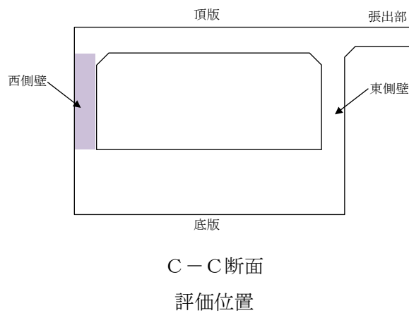
図 6-2 鉄筋コンクリート部材の曲げ軸力照査が最も厳しくなるケースでのひずみ分布図 (第一ガスタービン発電機用燃料タンク基礎(側壁④), 解析ケース①, 地震動 Ss-1-1, t=5.96s)
