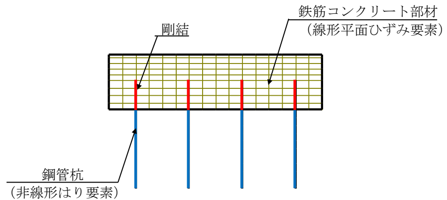
(a) 第一ガスタービン発電機基礎 (A-A断面, 構造物部分拡大部)
