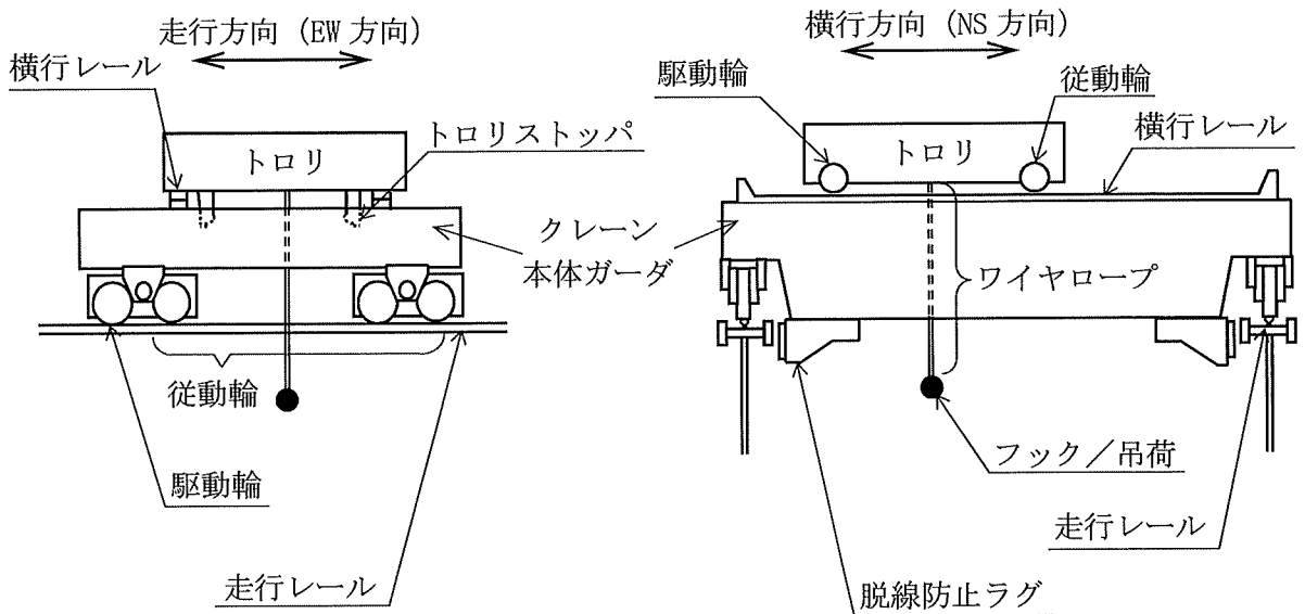
図4-1 構造概要図
