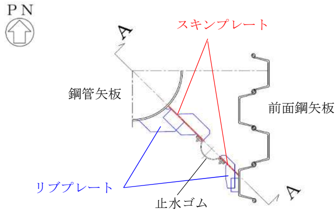
(a) 平面図
