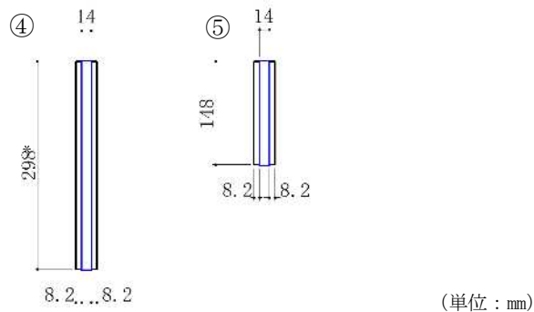
図3-18 照査モデル図（リブプレートと鋼管矢板又は前面鋼矢板接合部）
