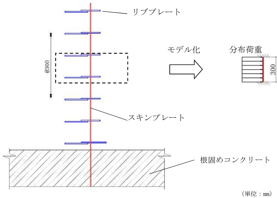
図 3-14 スキンプレート照査モデル図
