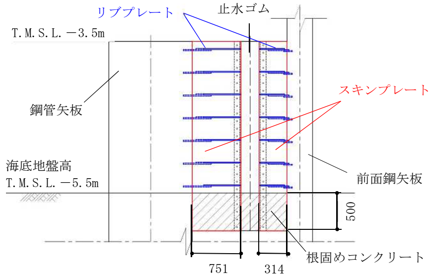
(b) A-A断面図
