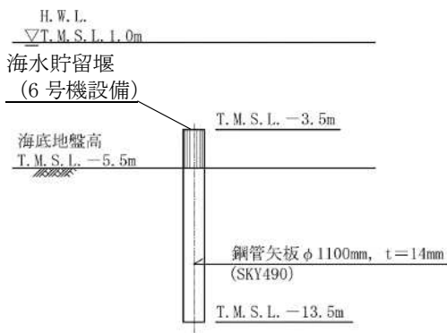
(a) A-A断面図
