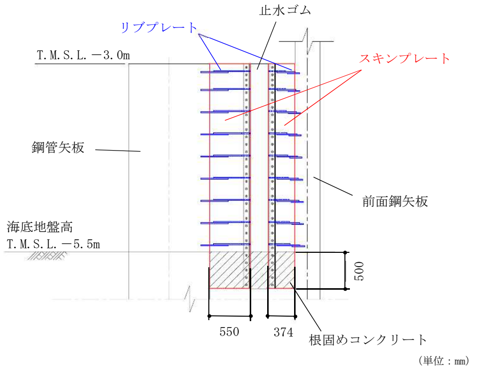
(b) A-A断面図
