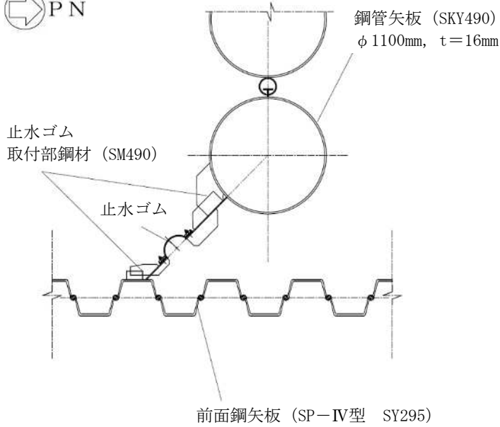
図 2-2 (2) 海水貯留堰 (6号機設備) の平面図 (A部拡大)
