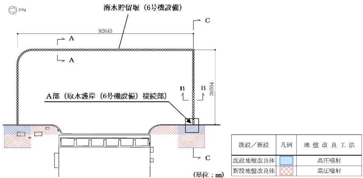
図2-2 (1) 海水貯留堰（6号機設備）の平面図
