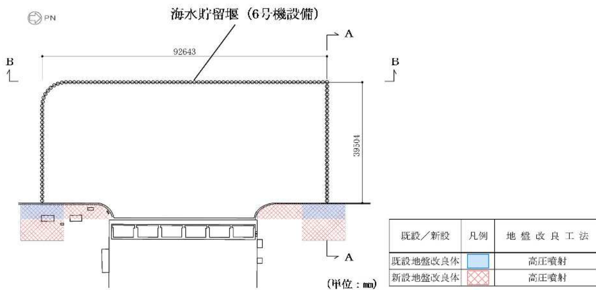
図3-1 海水貯留堰（6号機設備）の評価対象断面位置図
