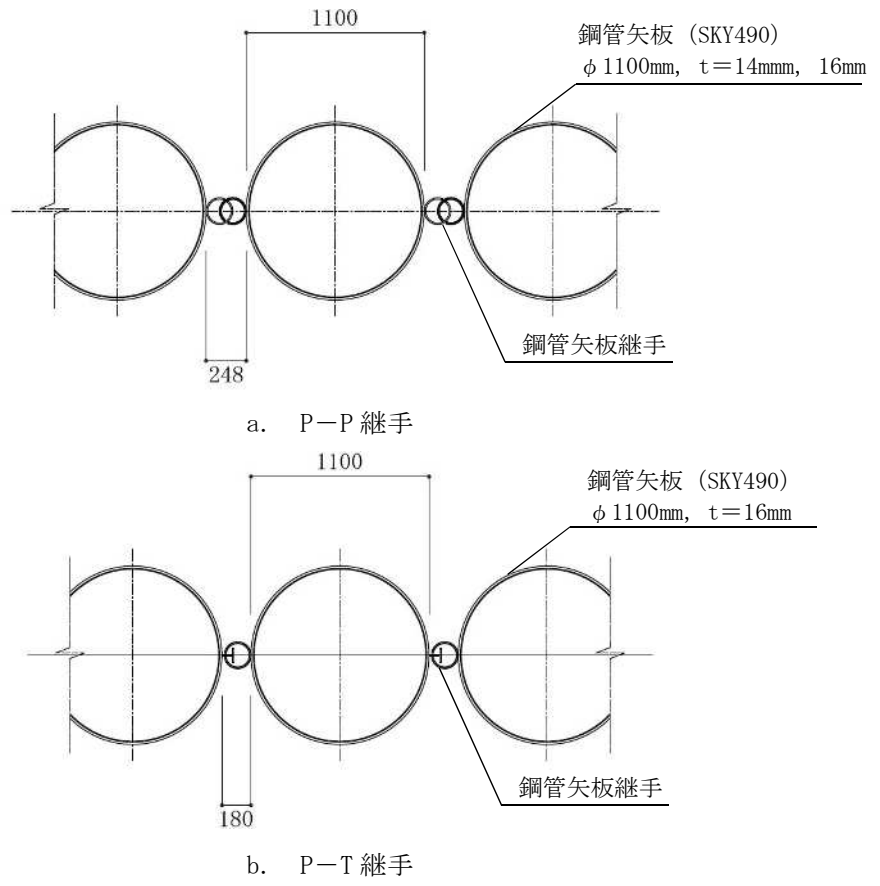
(d) 鋼管矢板継手部平面図
