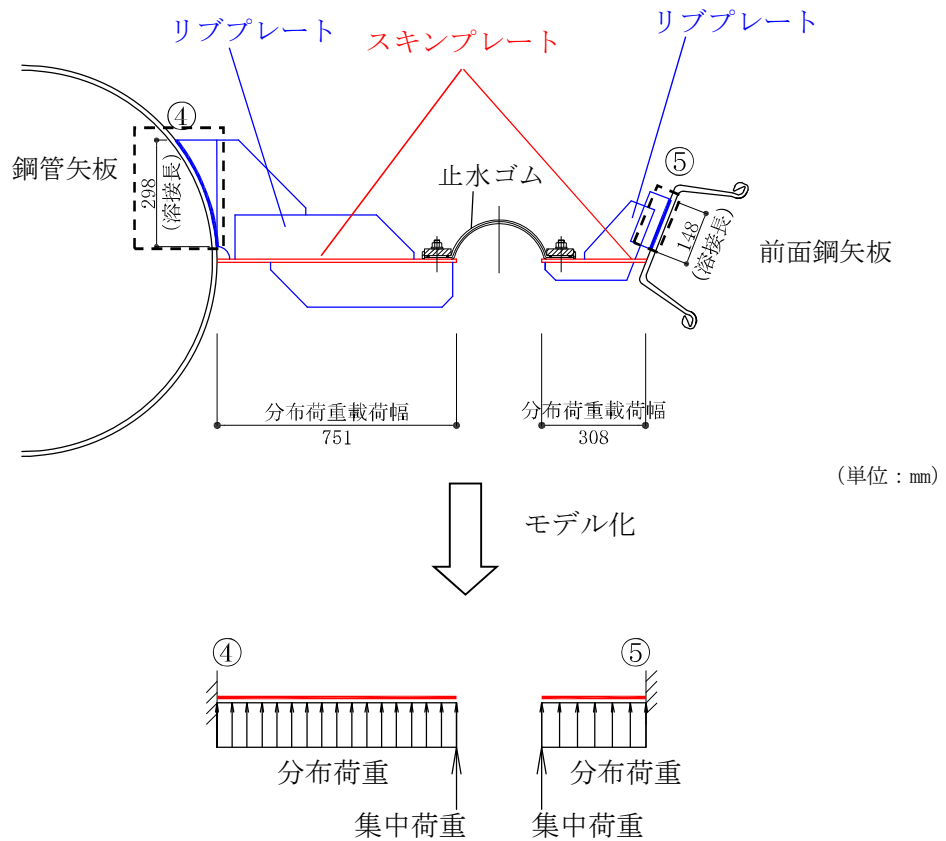
図3-18 照査モデル図（リブプレートと鋼管矢板又は前面鋼矢板接合部）
