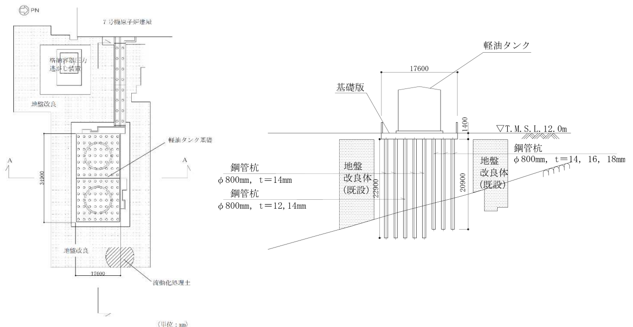
図 2-1 軽油タンク基礎の断面図（A-A断面）
