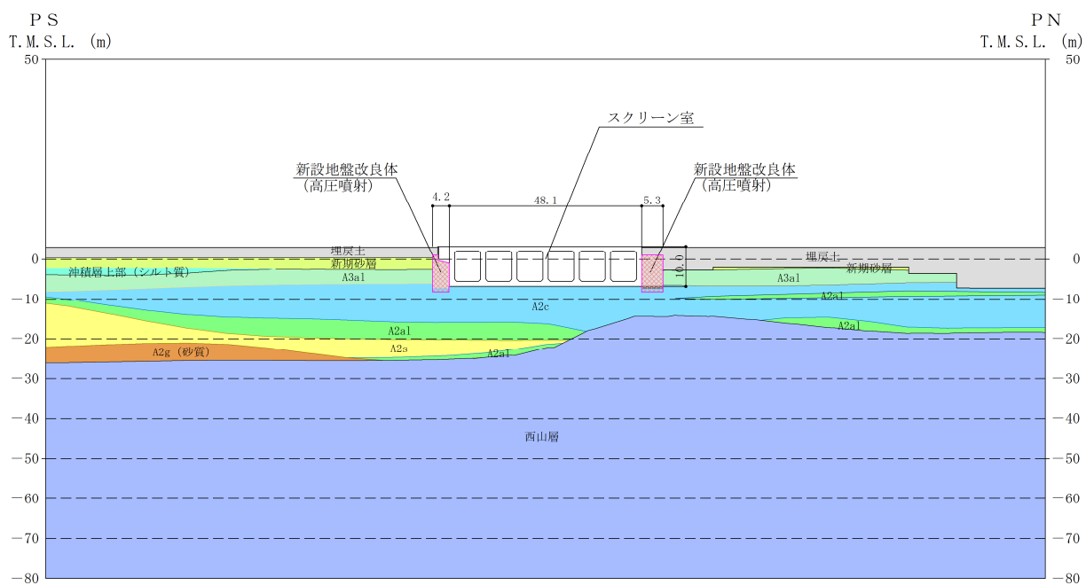
図 4-5 スクリーン室の周辺地質断面図 (A-A断面 ブロック①)
