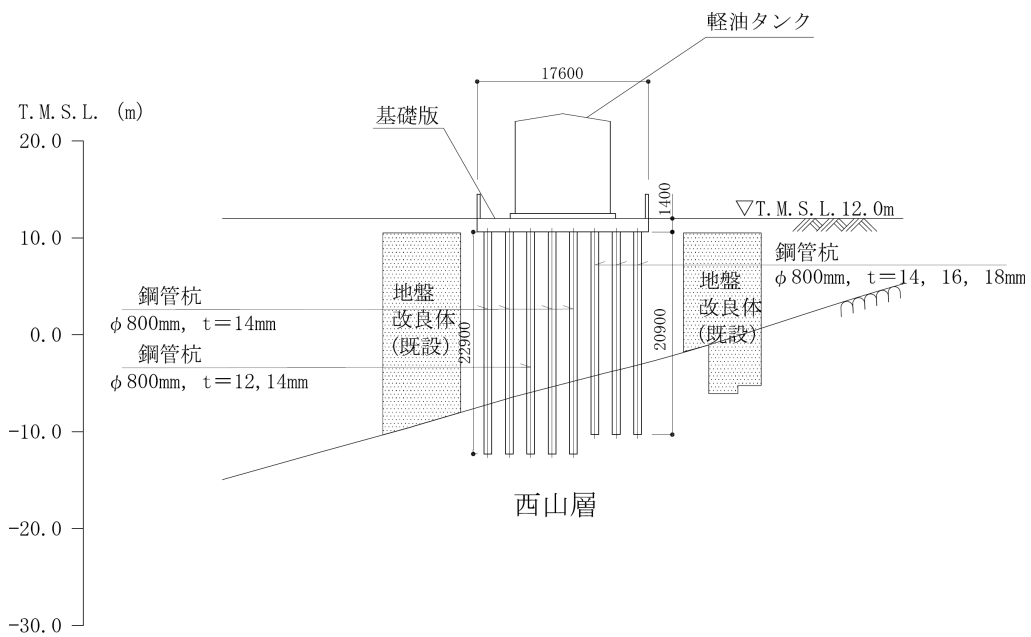
図 4-20 (1) 軽油タンク基礎の断面図 (A-A断面)
