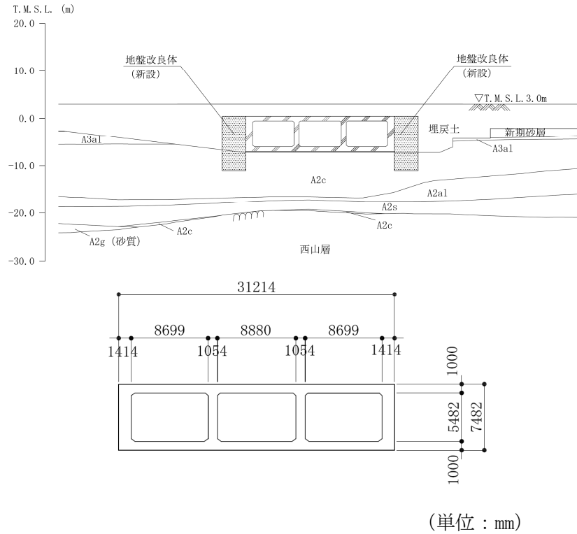
図 4-37 (1) 取水路 (6 号機設備) の断面図 (漸縮部 A-A 断面 ②ブロック)
