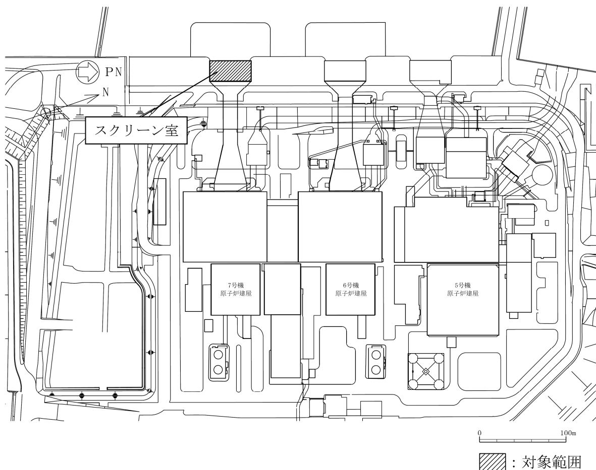
図 4-2 スクリーン室の平面配置図
