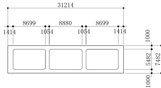
図 4-8 (1) 取水路の断面図 (漸縮部 A-A断面 ブロック②)
