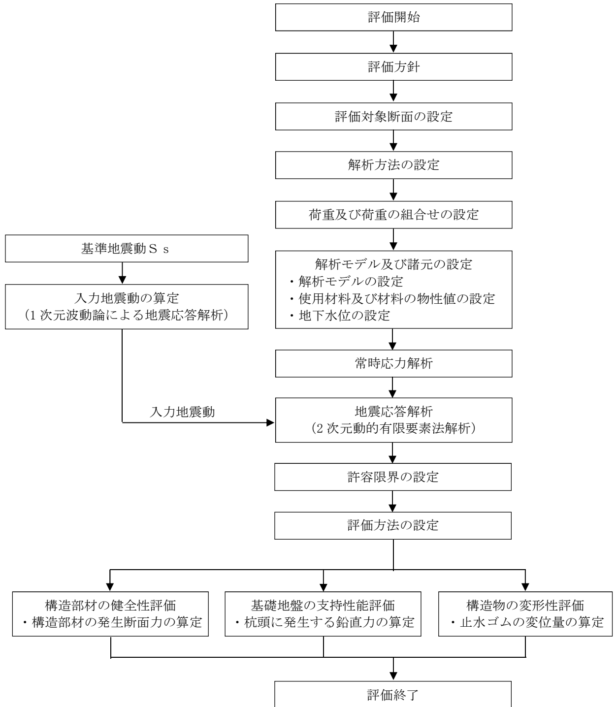
図 2-4 海水貯留堰の耐震評価フロー
