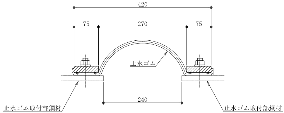
図 3-13 止水ゴムの構造図
