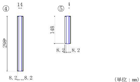
図 3-18 照査モデル図（リッププレートと鋼管矢板又は前面鋼矢板接合部）
