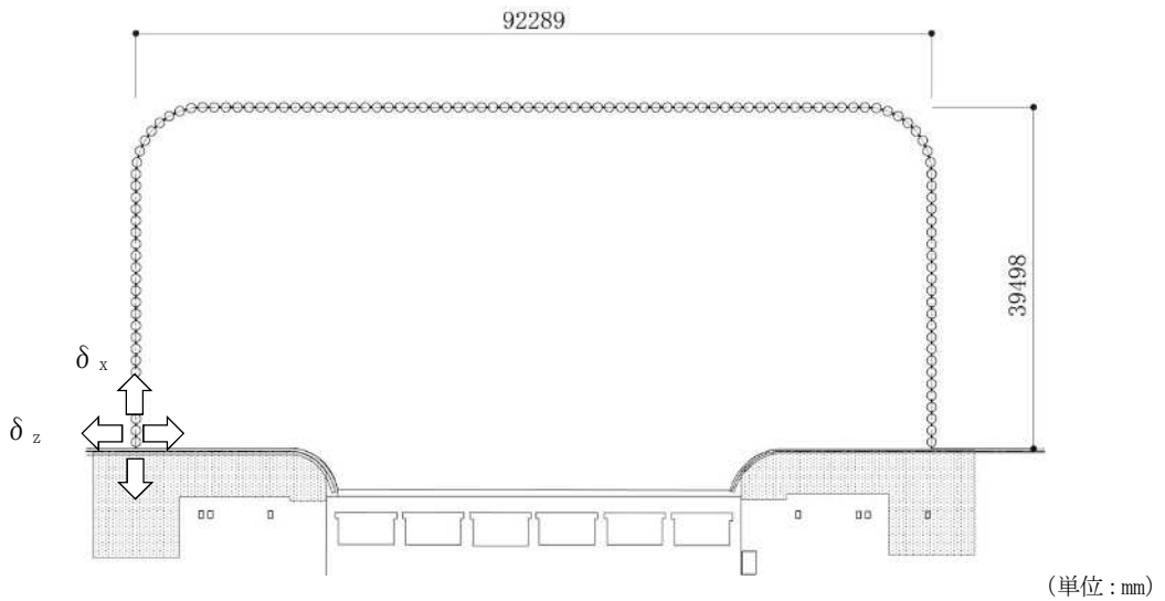
図 3-22 変位方向の定義 ( \delta_x , \delta_z 平面図)
