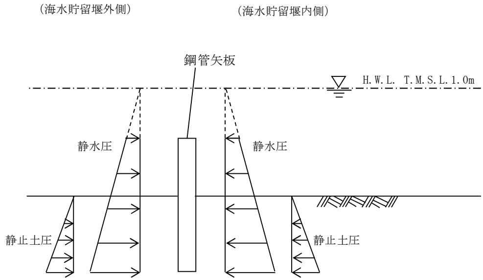
図 3-3 荷重作用図 (鋼管矢板 常時)
