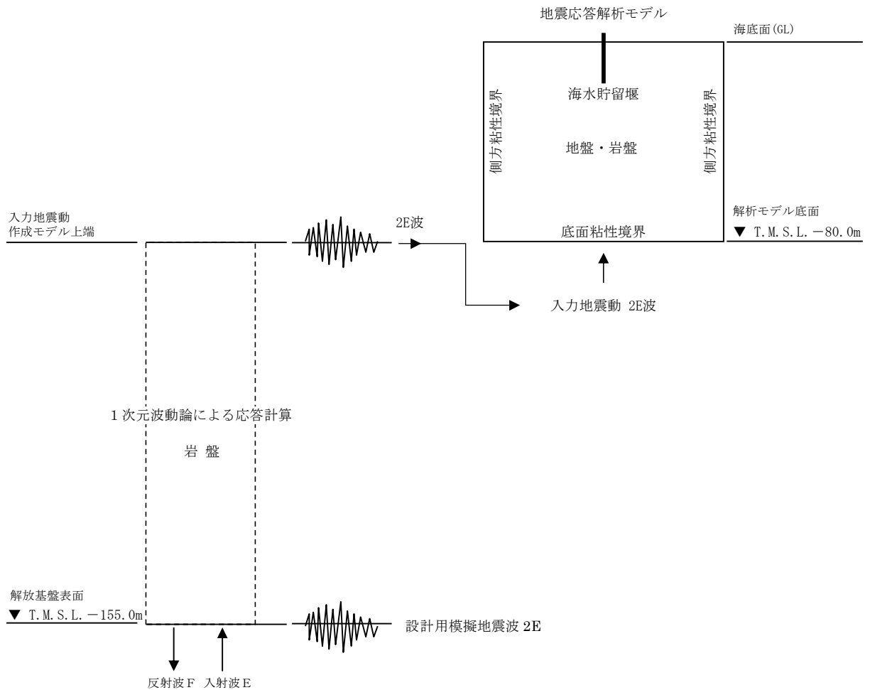
図 3-6 入力地震動算定の概念図
