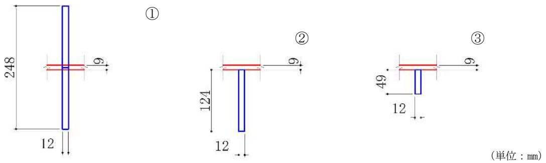
図 3-16 照査モデル図 (リブプレートと鋼管矢板又は前面鋼矢板)
