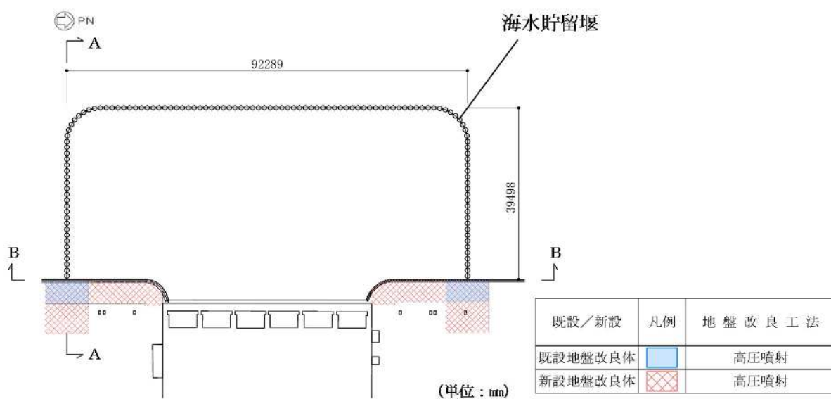
図3-1 海水貯留堰の評価対象断面位置図
