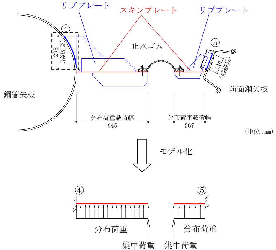
図 3-18 照査モデル図（リッププレートと鋼管矢板又は前面鋼矢板接合部）
