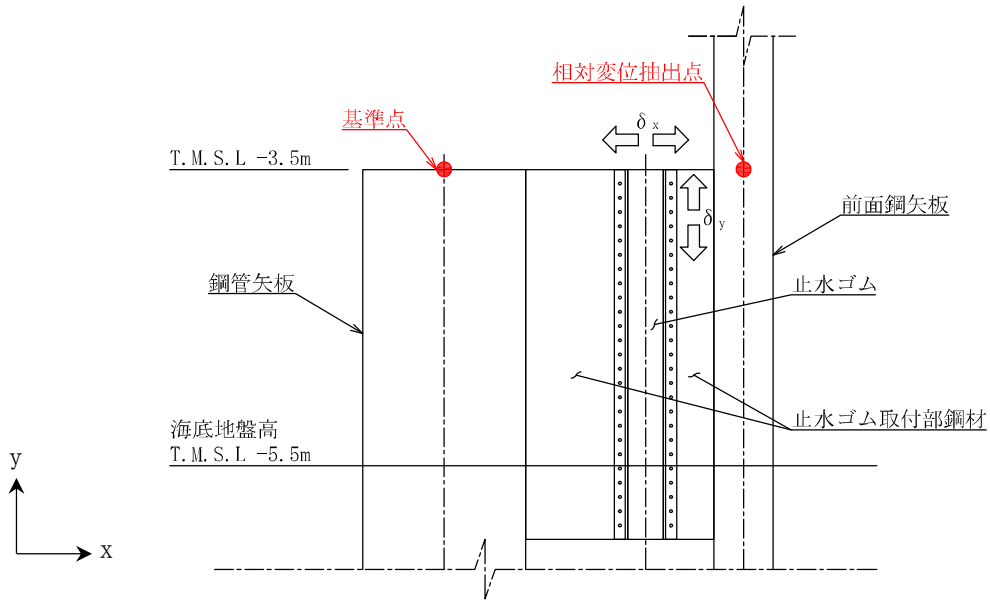
図 3-23 変位方向の定義 ( \delta_x , \delta_y 断面図)
