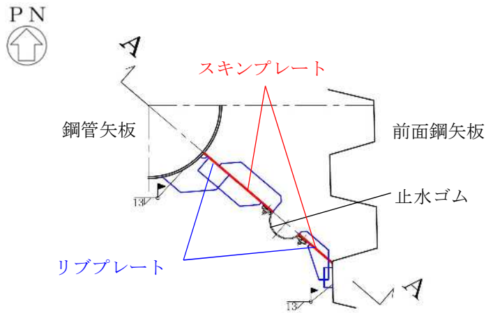
(a) 平面図
