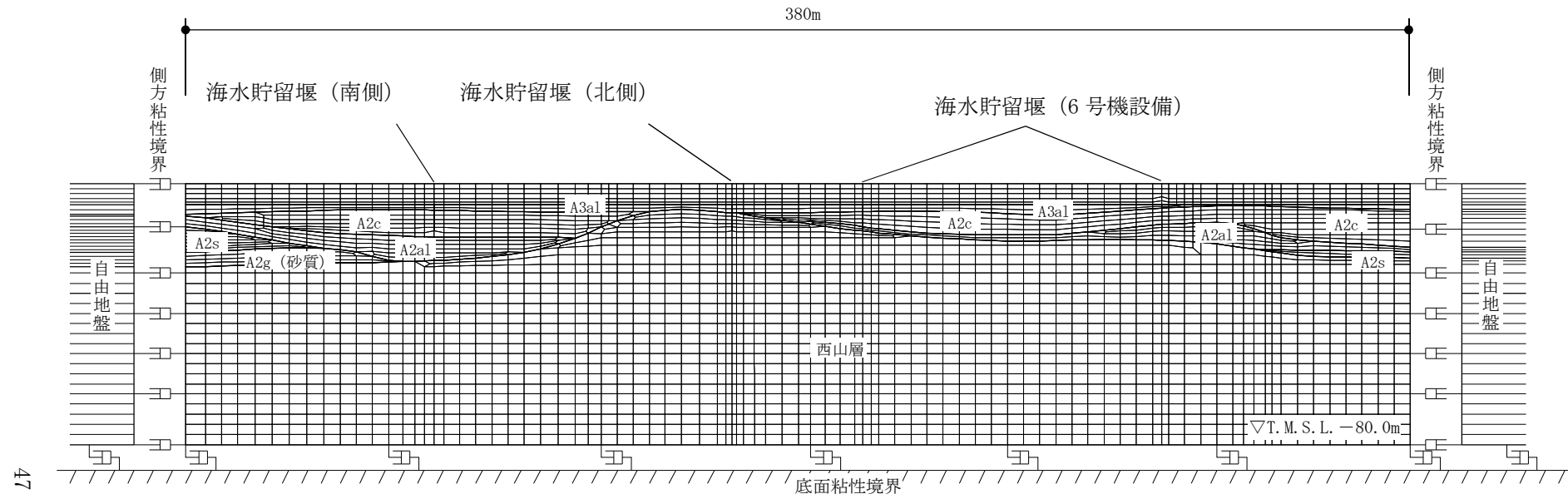
図 3-8 (2) 海水貯留堰の地震応答解析モデル (B-B断面)
