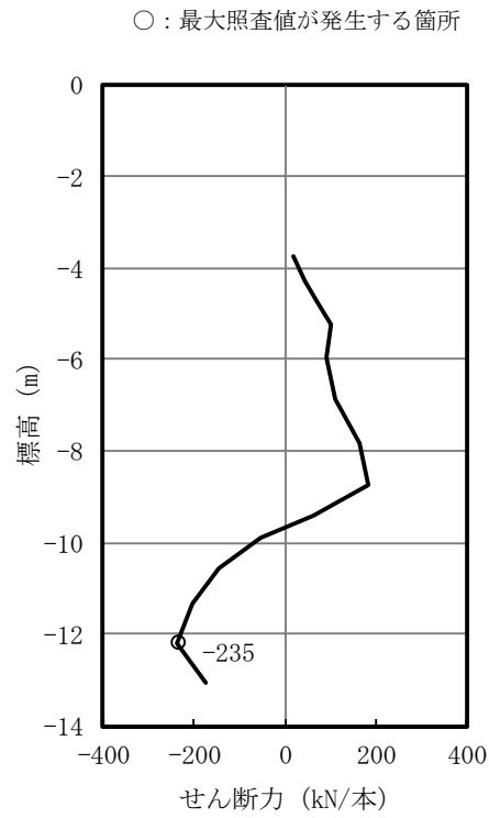
図 3-10 (1) 鋼管矢板のせん断力照査における最大照査値の評価時刻での断面力 (A-A断面 Ss-1++, t=18.66s) (検討ケース③: 地盤物性値のばらつき (-1σ) を考慮した解析ケース)
