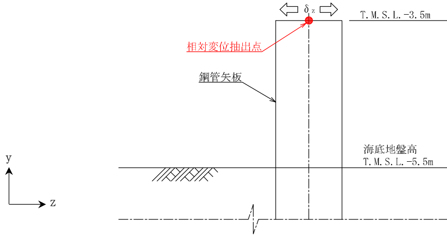
図 3-24 変位方向の定義 ( \delta_z 断面図)
