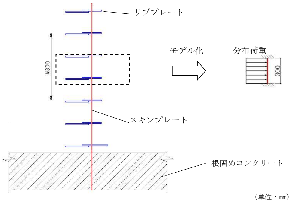
図 3-14 スキンプレート照査モデル図
