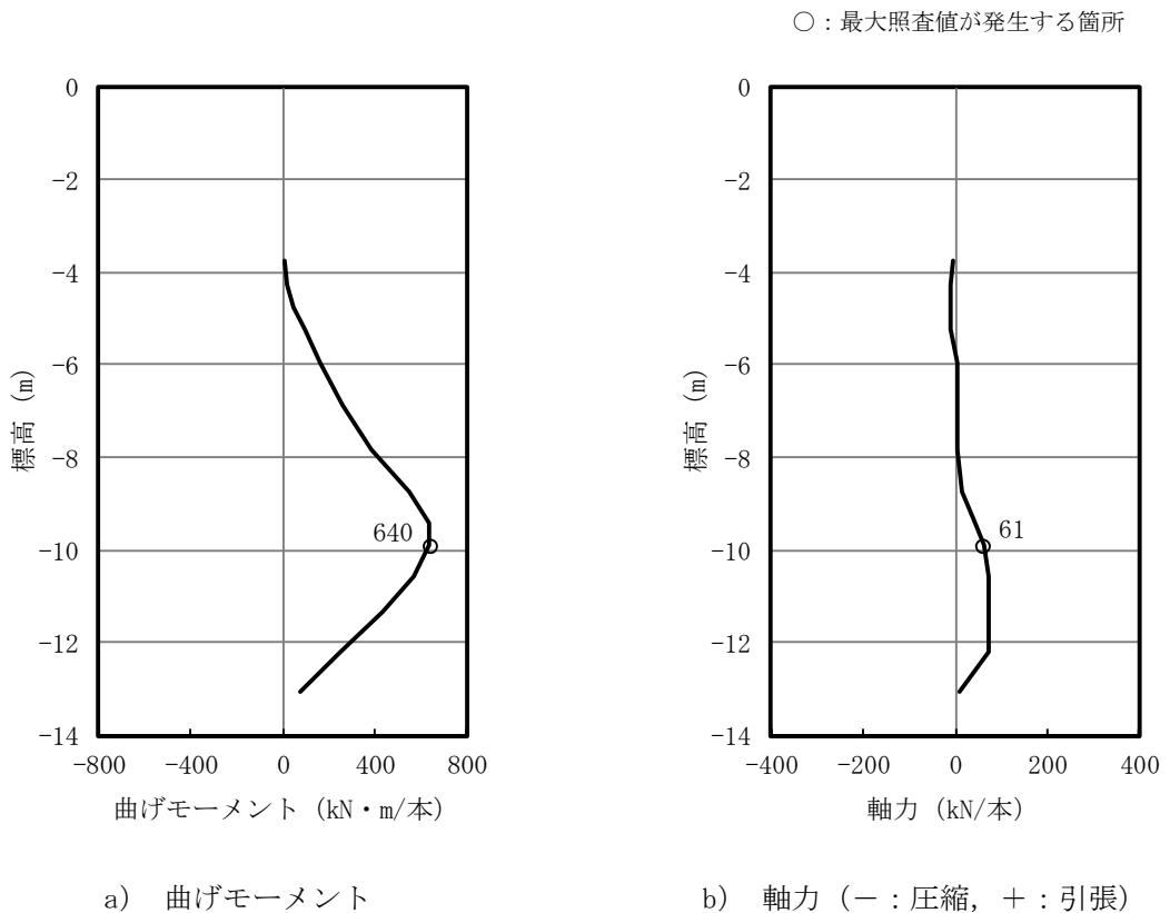
図3-9 (1) 鋼管矢板の曲げ軸力照査における最大照査値の評価時刻での断面力
