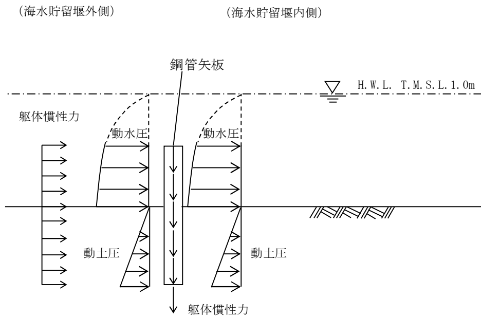
図 3-4 荷重作用図 (鋼管矢板 地震時)
