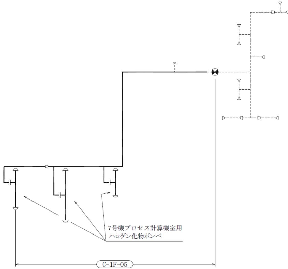
小空間固定式消火設備概略系統図 (その 91)
