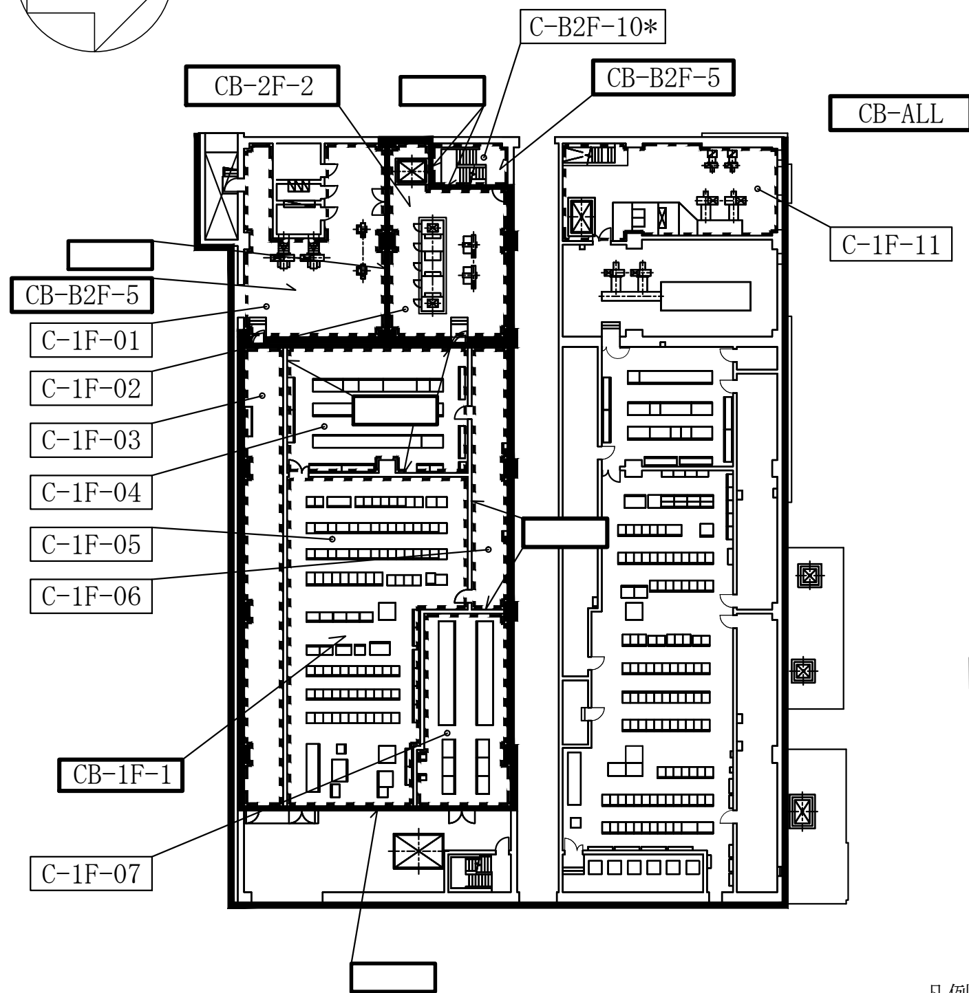
コントロール建屋 T.M.S.L. 12300
