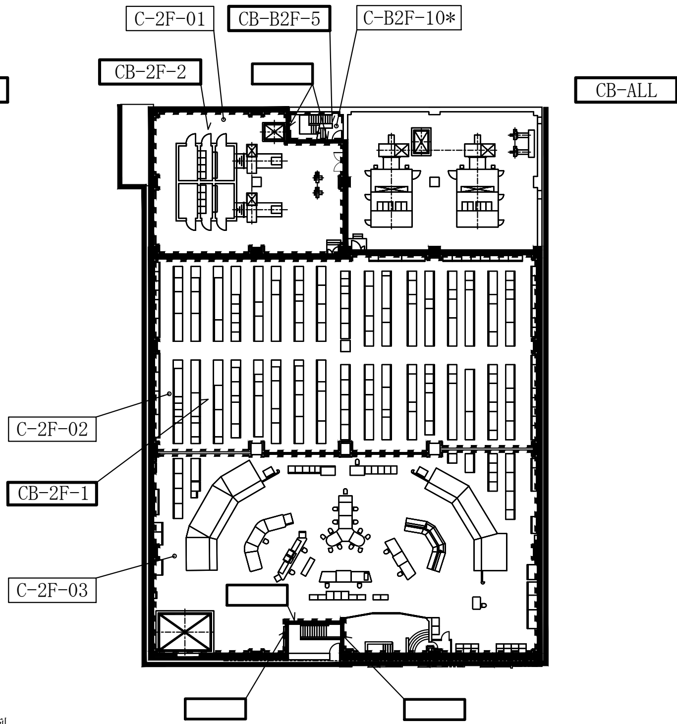
コントロール建屋 T.M.S.L. 17300
