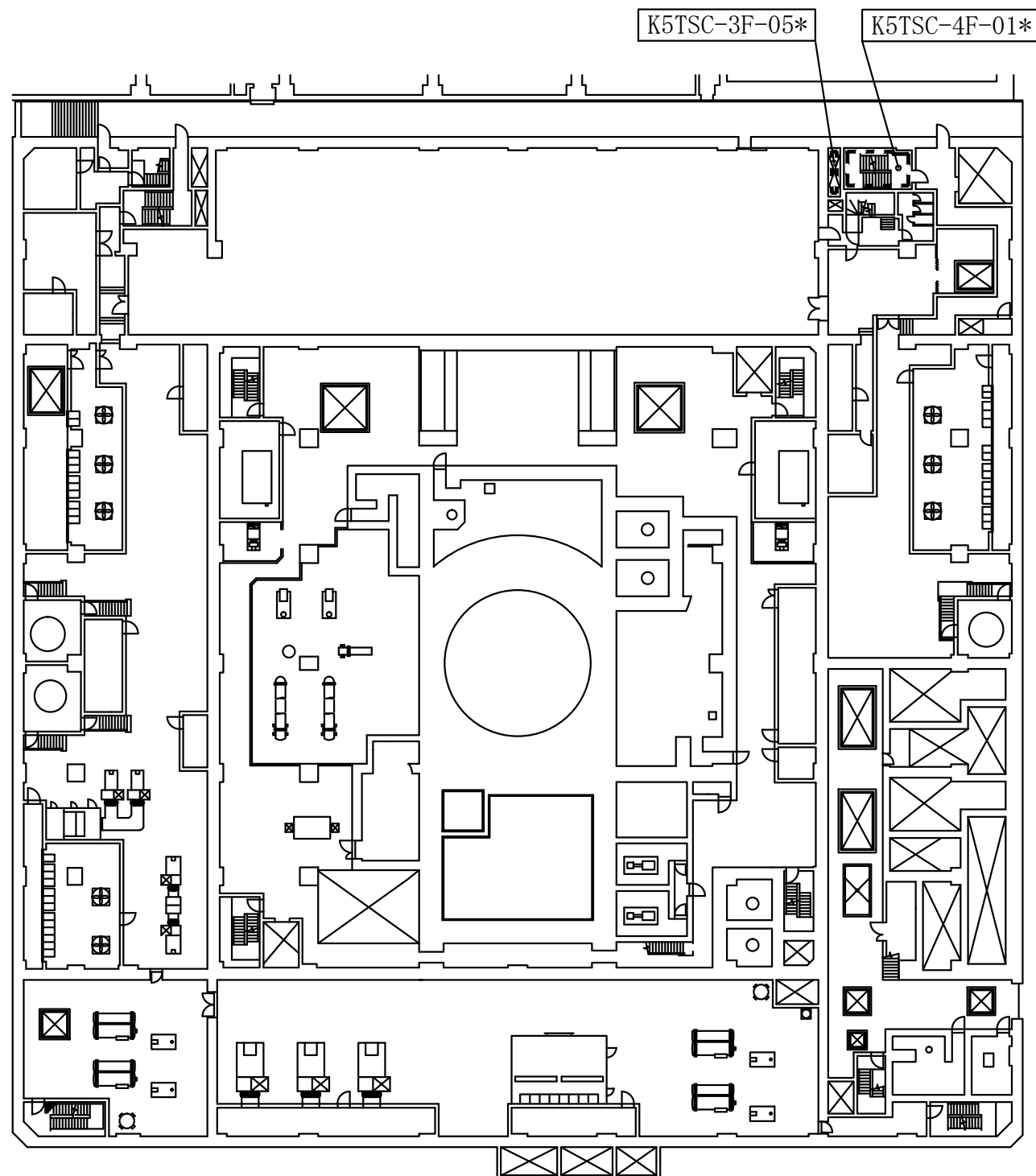
原子炉建屋 T.M.S.L. 20300
