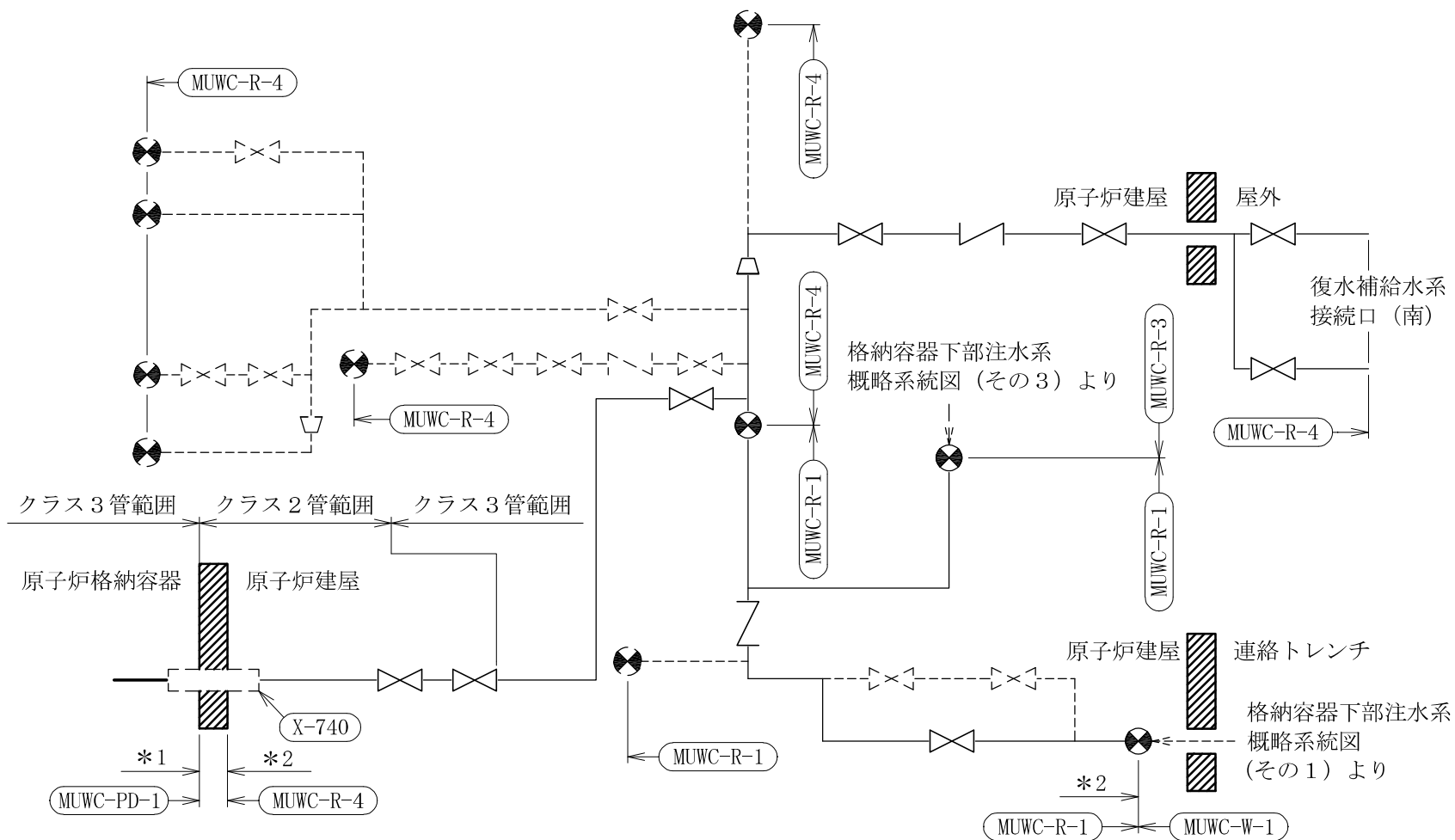
格納容器下部注水系概略系統図 (その2)
