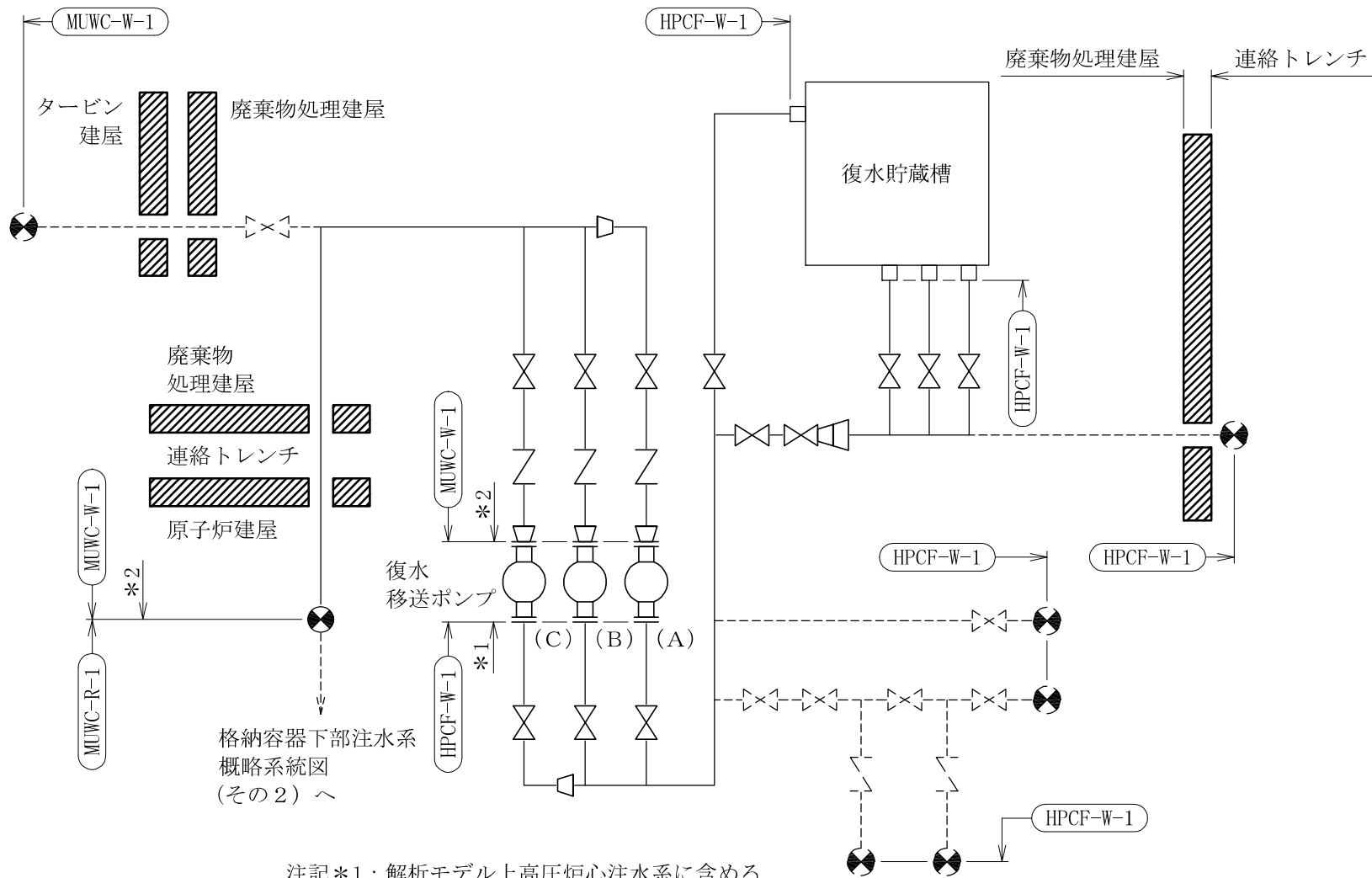
格納容器下部注水系概略系統図 (その1)
