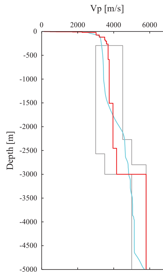
推定された鉛直分布 Vp
