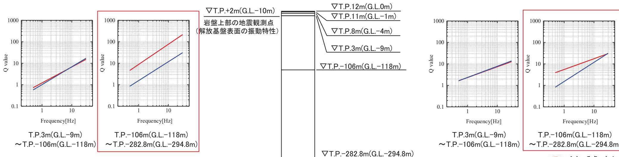
《推定された Q_s 》
