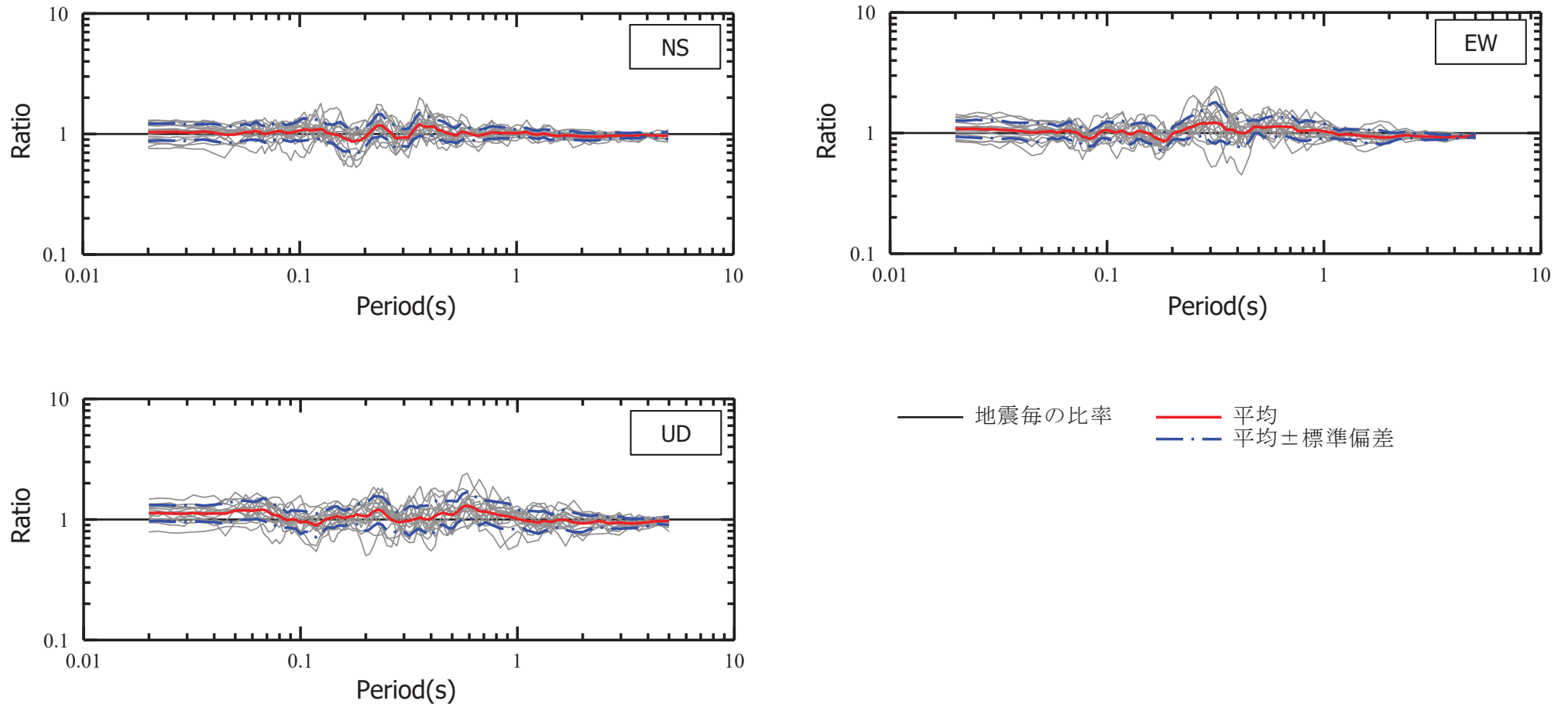
原子炉建屋直下(T.P.-82.8m)に対する自由地盤(T.P.-82.8m)の観測記録の応答スペクトル比(PN基準) 自由地盤(T.P.-82.8m)／原子炉建屋地中(T.P.-82.8m)
