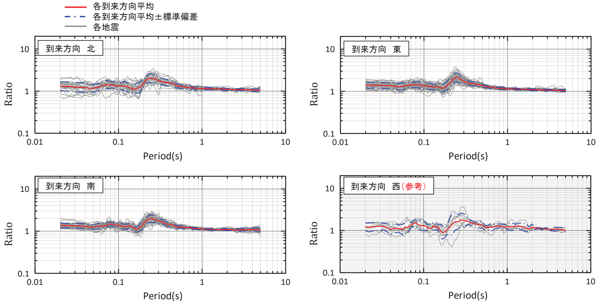
地震波到来方向別の応答スペクトル比 原子炉建屋直下 水平成分 (PN基準)
