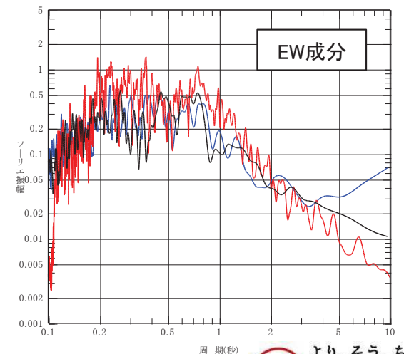
余震(要素地震)のフーリエスペクトル(スムージング)
