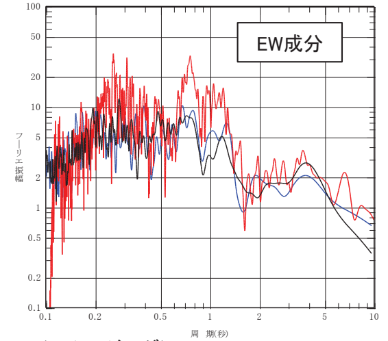
本震のフーリエスペクトル(スムージング)
