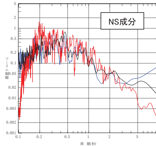
余震(要素地震)のフーリエスペクトル(スムージング)
