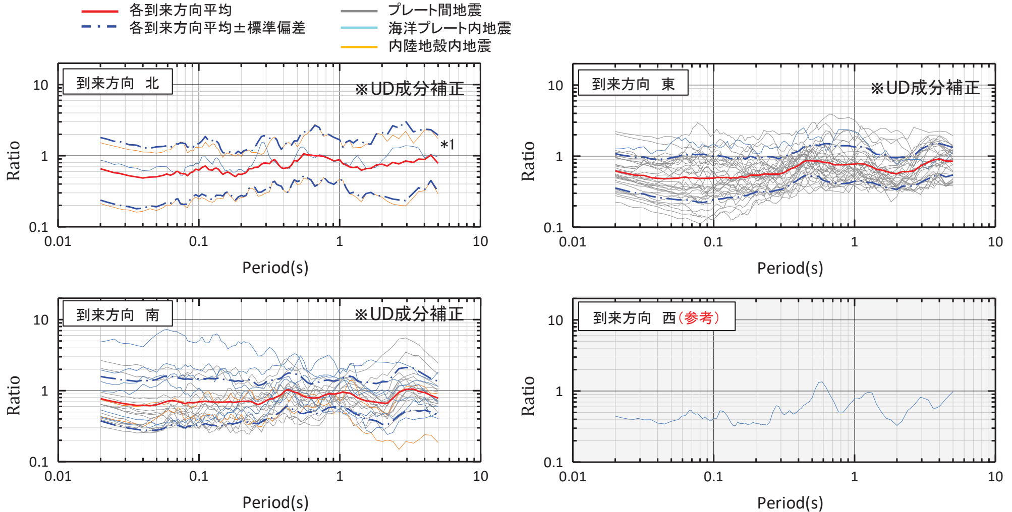
観測記録とNoda et al.(2002)との比較 地震波到来方向別 鉛直成分 自由地盤の岩盤上部地震観測点 (T.P.+2.0m) / Noda et al.(2002)
