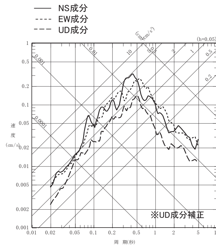
応答スペクトル
