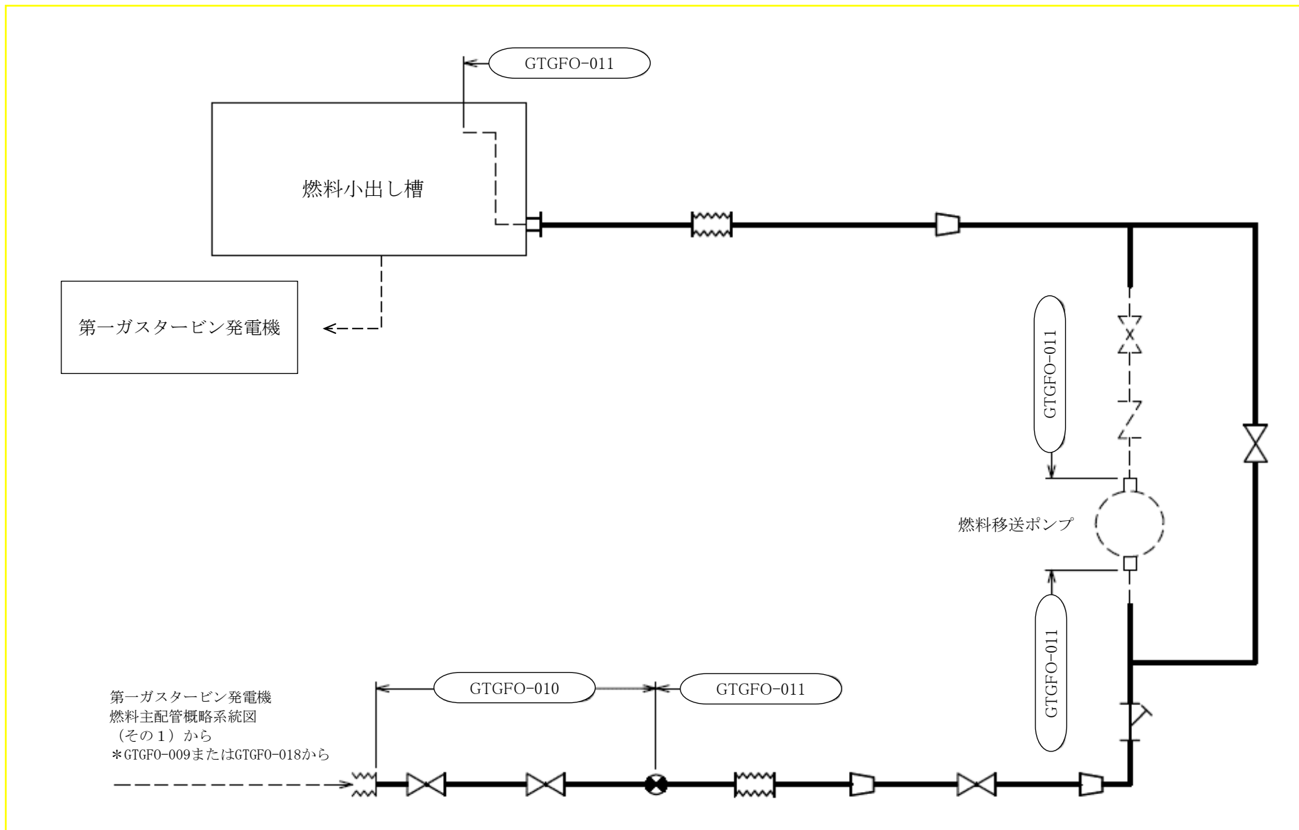
第一ガスタービン発電機 燃料主配管概略系統図 (その2)
