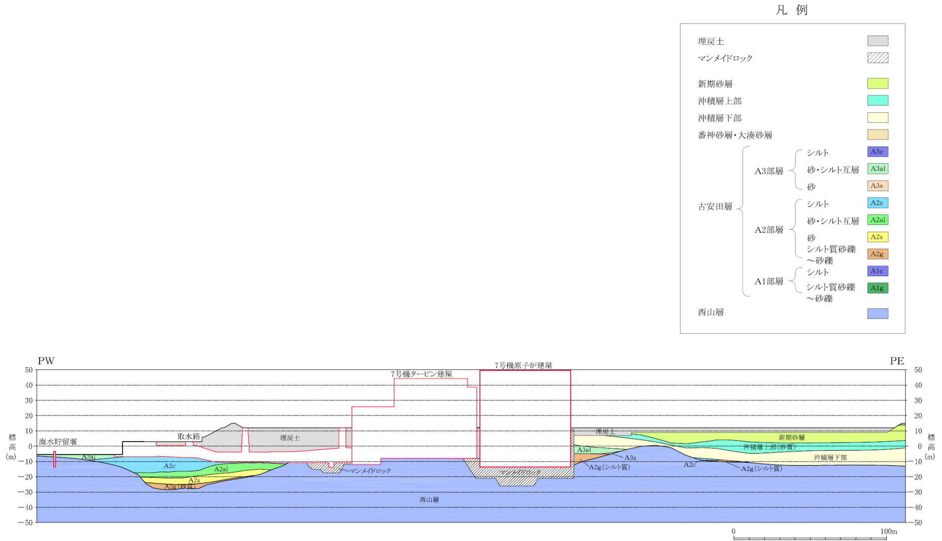
図 6-3 汀線直交 地質断面図 (7号機原子炉建屋炉心中央) (B-B断面)
