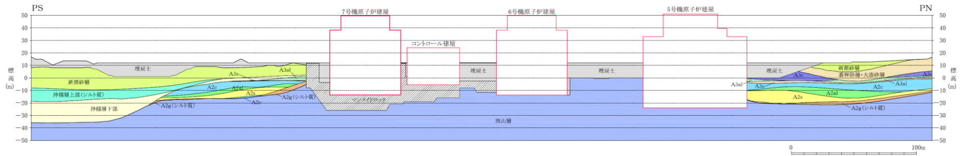
図6-2 汀線平行 地質断面図(7号機原子炉建屋炉心中央)(A-A断面)
