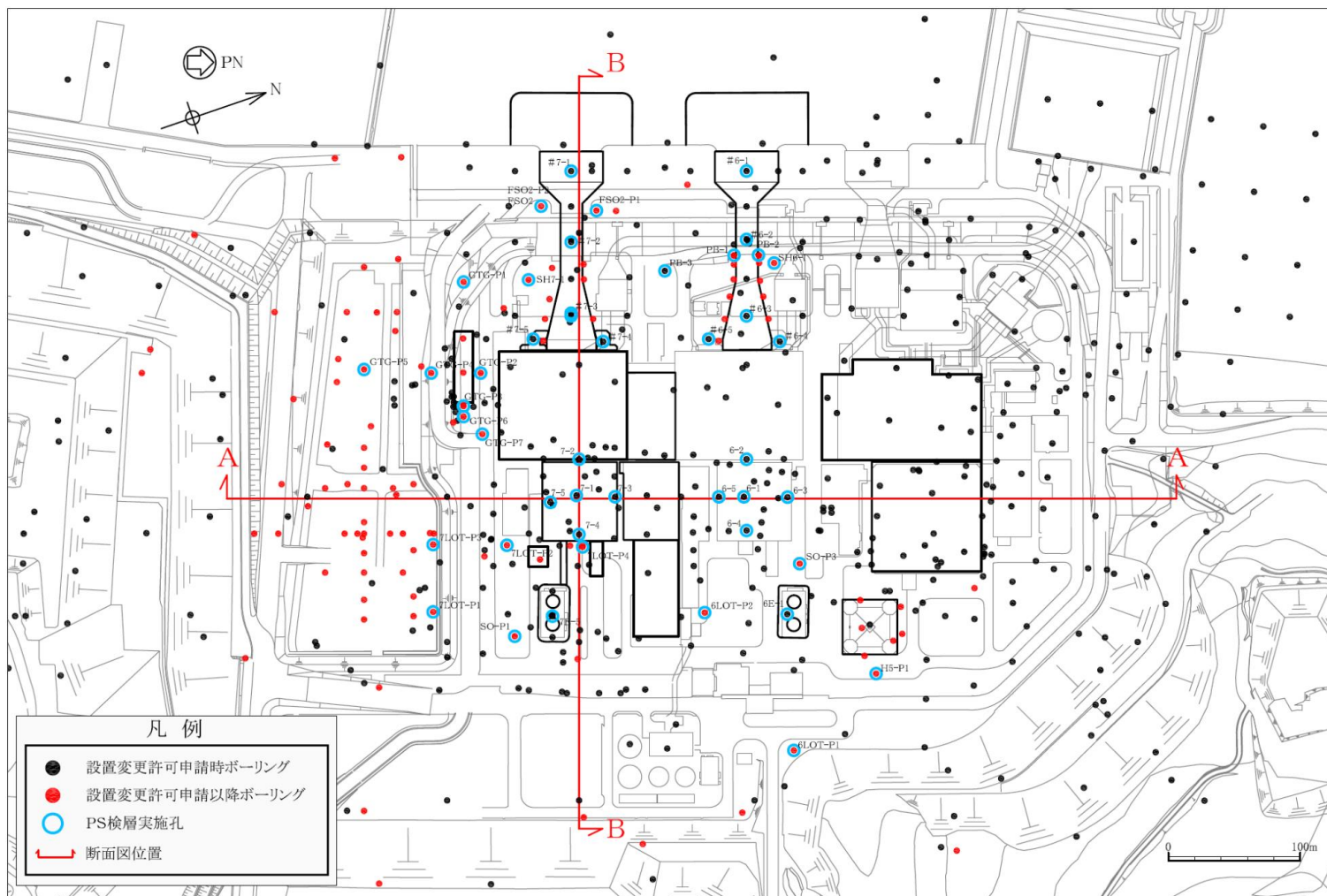
図 6-1 ボーリング調査位置図
