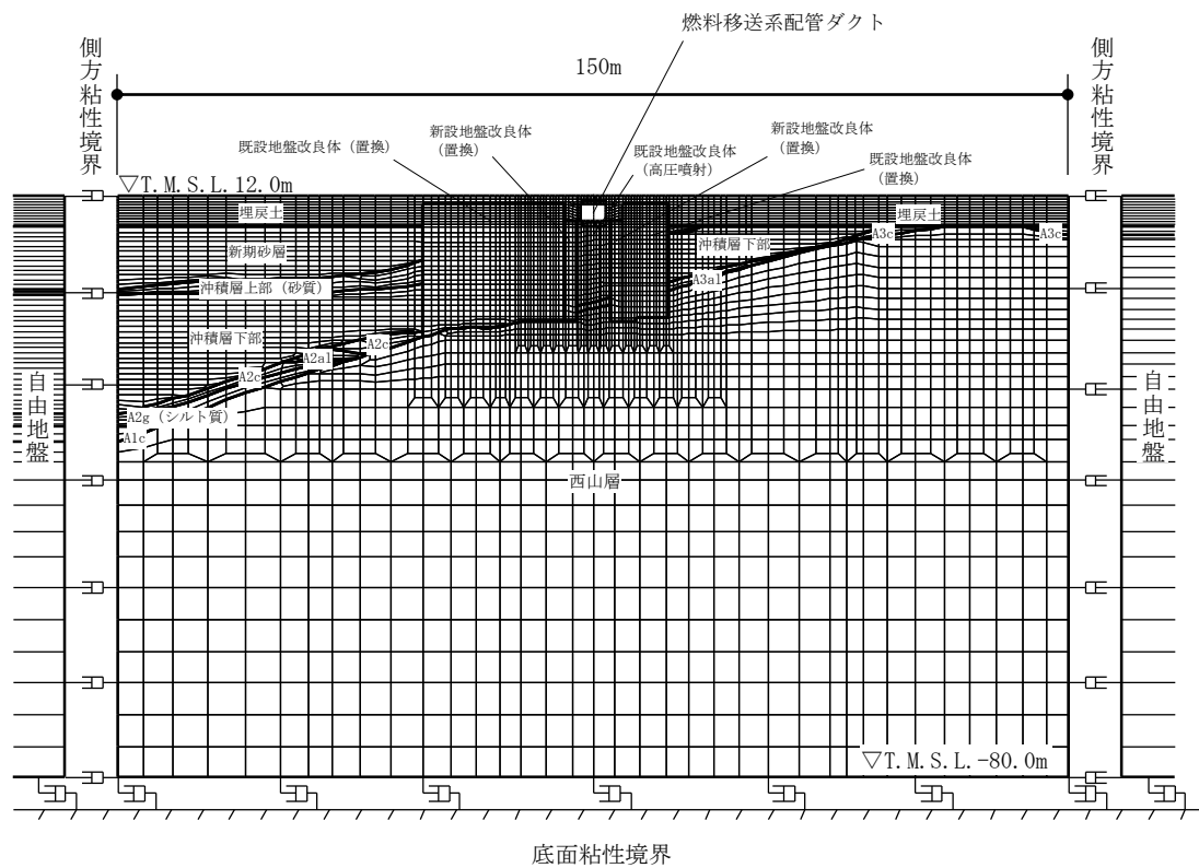
図 3-11 (2) 燃料移送系配管ダクトの地震応答解析モデル (B-B断面)
