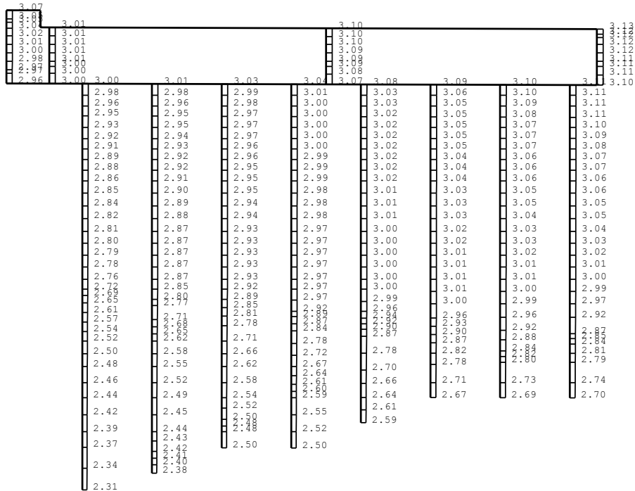
(a) Sd-6EW, 水平
