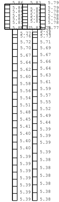
(a) Ss-1++, 水平
