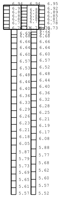
(a) Ss-3—, 水平
