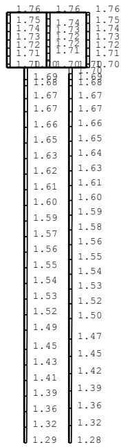
(a) Sd-4NS, 水平
