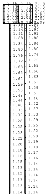
(a) Sd-4NS, 水平
