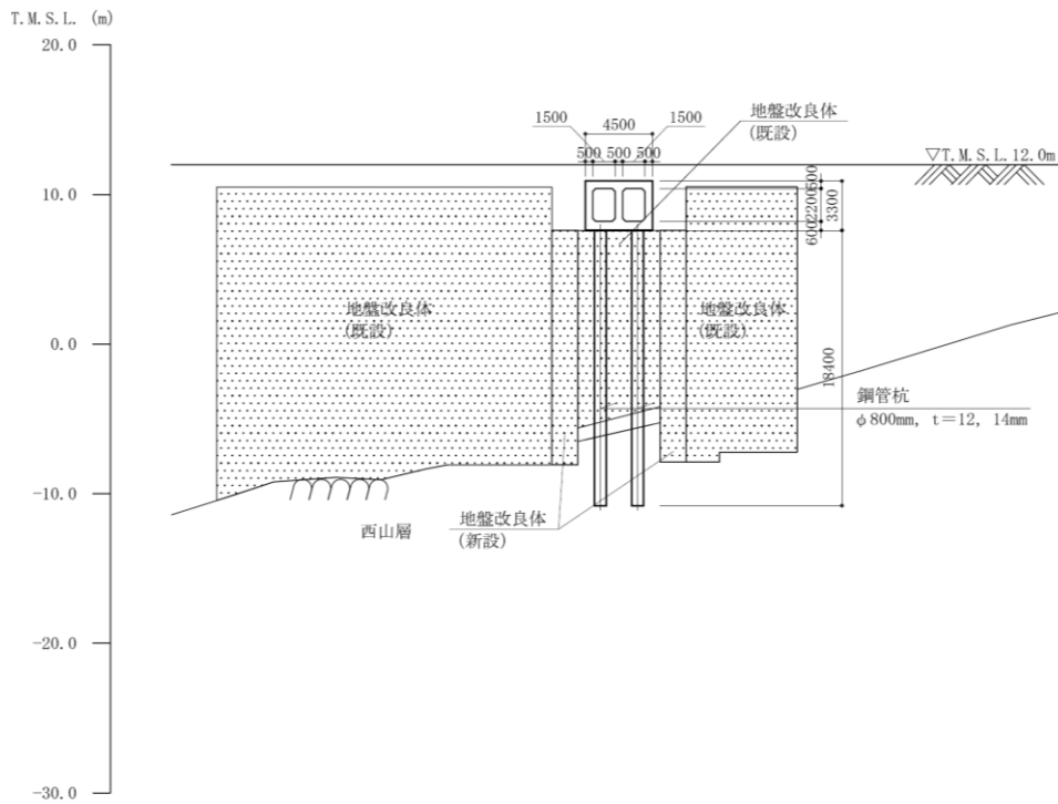
図 2-3 (2) 燃料移送系配管ダクトの断面図 (B-B断面)
