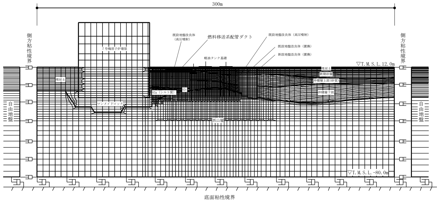
図 3-11 (3) 燃料移送系配管ダクトの地震応答解析モデル (C-C断面 機器・配管系に対する応答加速度抽出用)
