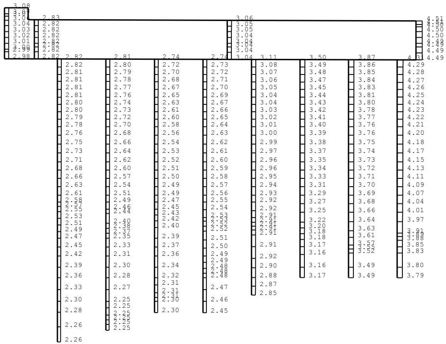
(b) Ss-5EW, 鉛直
