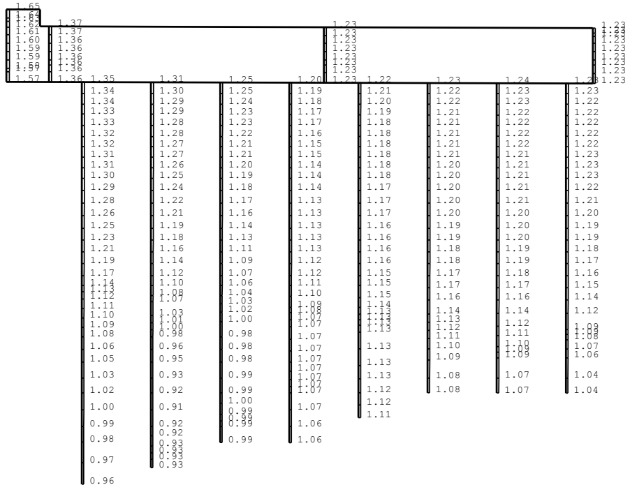
(b) Sd-8+, 鉛直
