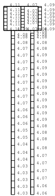
(a) Ss-3+, 水平
