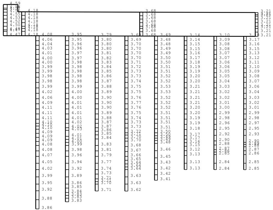
(b) Ss-7EW, 鉛直
