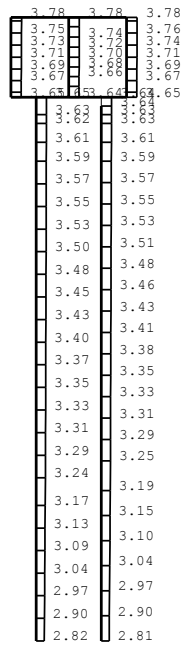
(a) Ss-4NS, 水平
