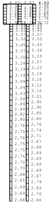
(a) Sd-1-+, 水平
