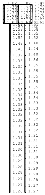
(a) Sd-7NS, 水平
