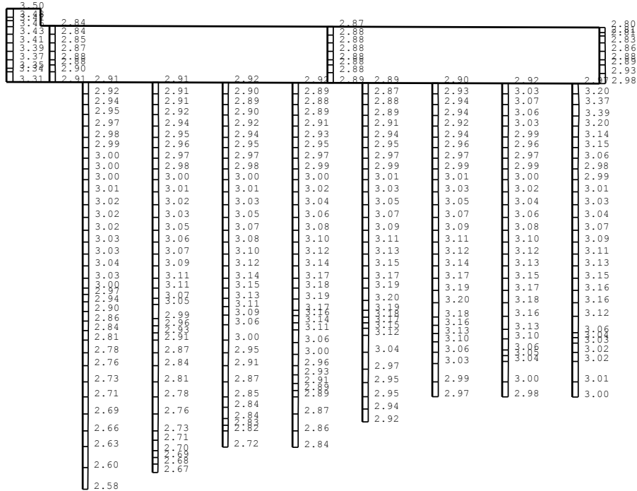
(a) Sd-8+, 水平
