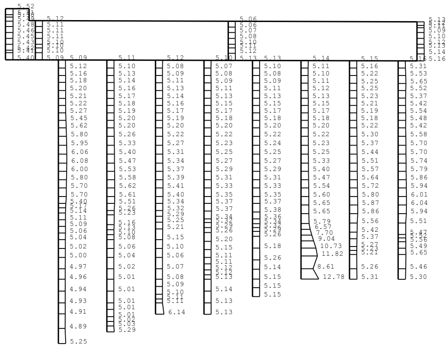
(a) Ss-3—, 水平
