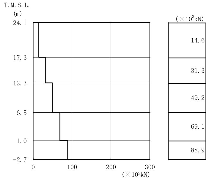
図 4-4 最大応答せん断力 (NS 方向)
