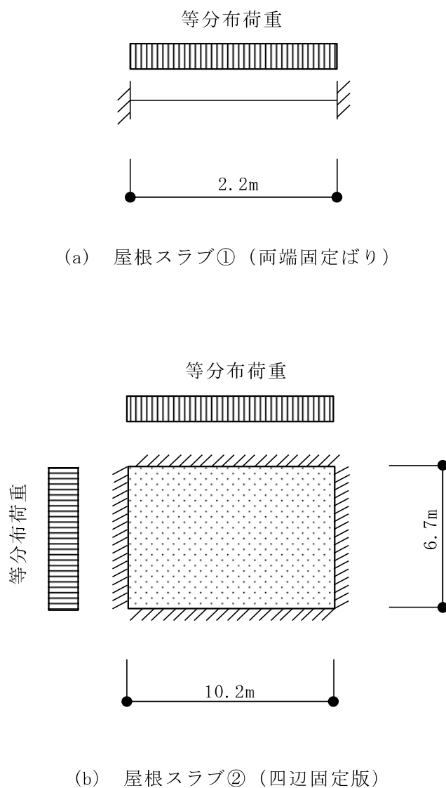
図 3-2 屋根スラブの解析モデル
