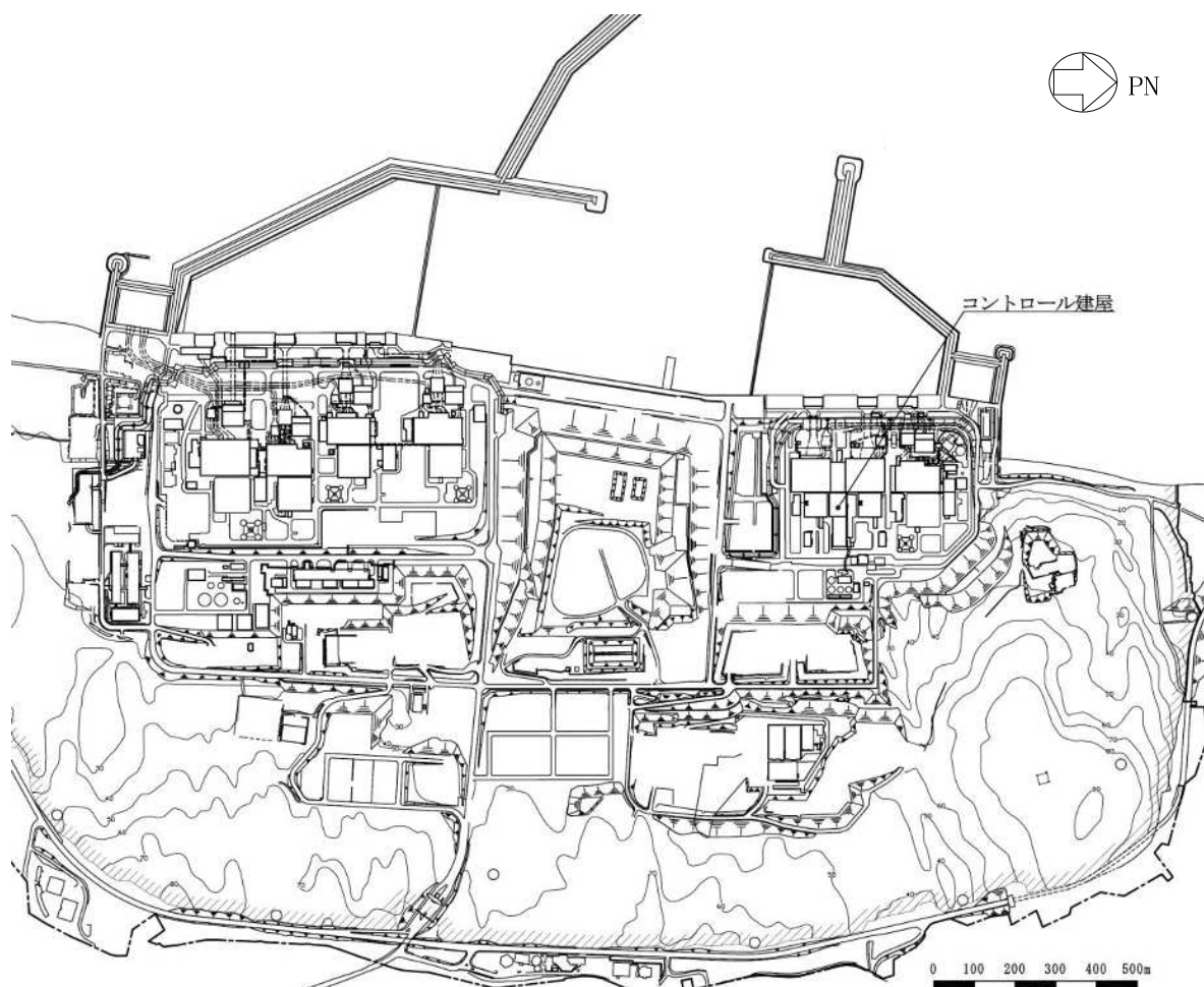
図 2-1 コントロール建屋の配置図
