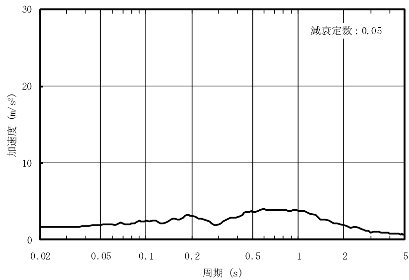
図 3-5 入力地震動の加速度応答スペクトル (年超過確率 10^{-2} 相当地震動, 水平方向, T. M. S. L. -5.5m)
